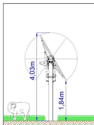
Figura 3. Caratteristiche del pannello
