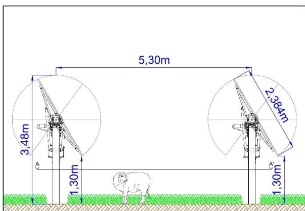
Figura 3. Caratteristiche del pannello
