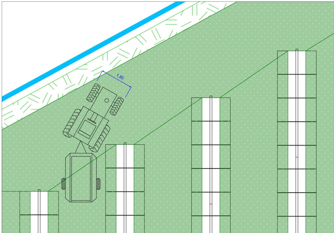
Figura 7. Rappresentazione del raggio di sterzata del macchinario per la raccolta
