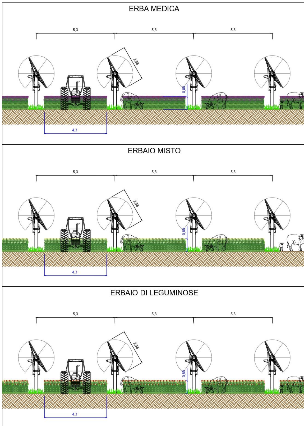
Figura 6. Rappresentazione del prospetto frontale dell'erba medica, erbaio misto ed erbaio di leguminose
