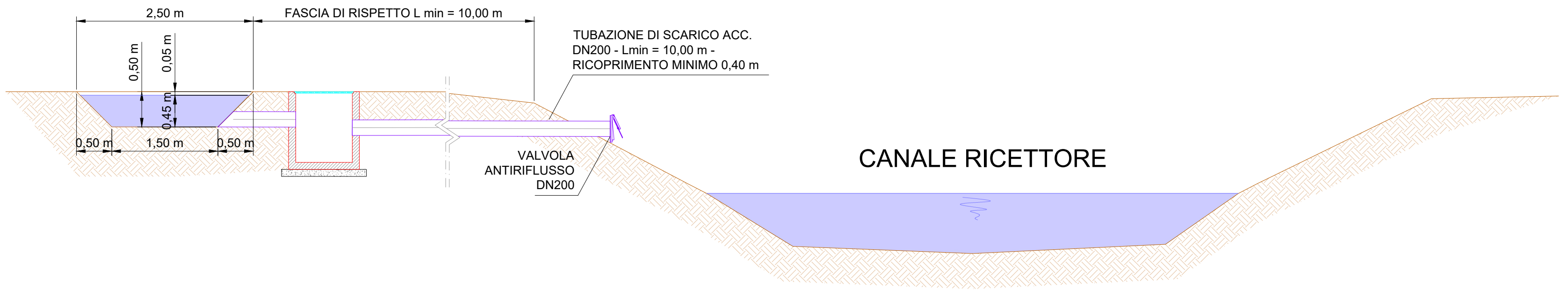
SEZIONE TIPOLOGICA BACINI DI LAMINAZIONE - SCALA 1:50
