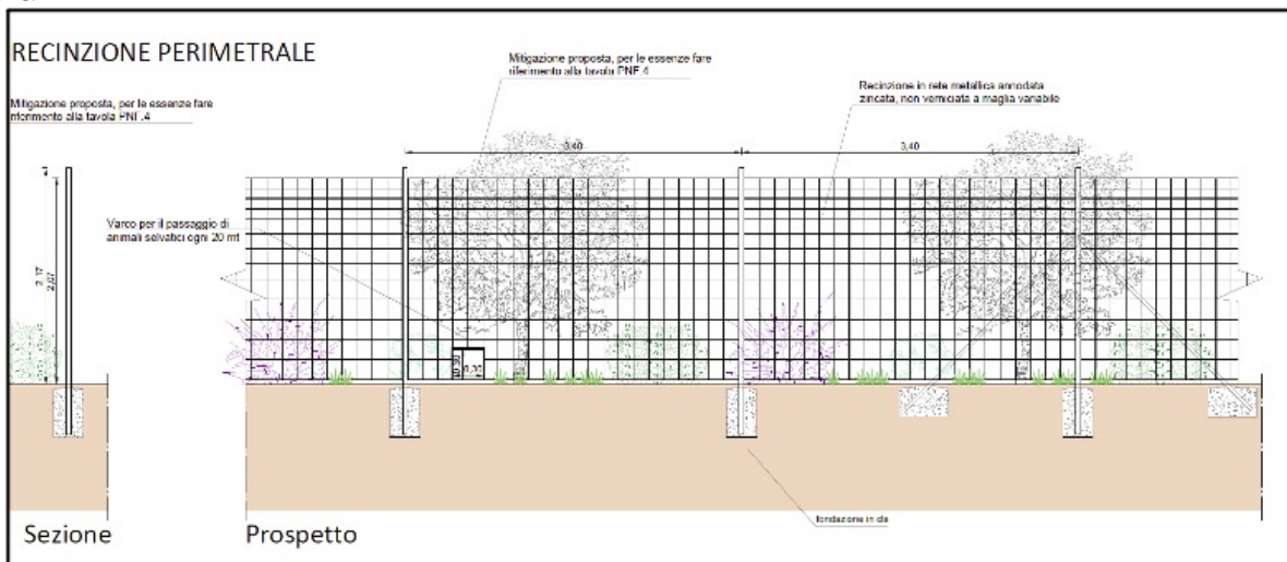
Figura 52 - Recinzione perimetrale con passaggi ecofaunistici
