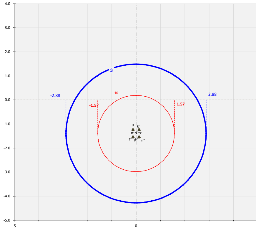
Figura 6: Curve di equilivello per il campo di induzione magnetica generato dalla linea (Sezione 4 – quattro terne a 36 kV)
