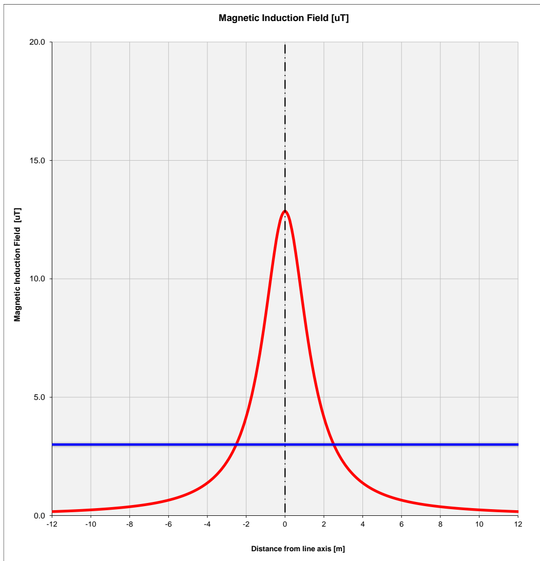
Figura 4: Andamento dell'induzione magnetica prodotta dalla linea in cavo per la sezione 4 (quattro terne a 36 kV)
