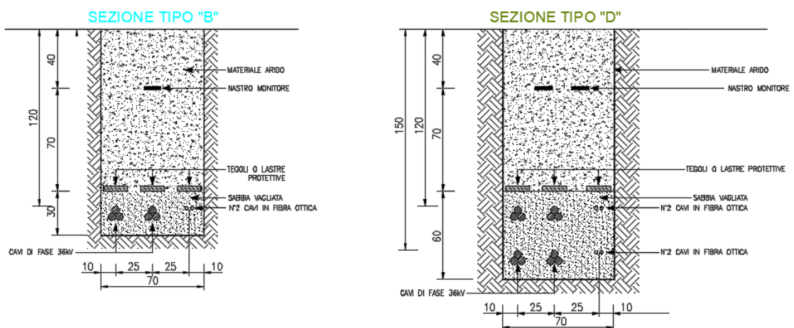
Figura 1: Sezioni tipiche di posa della linea in cavo su strade sterrate
