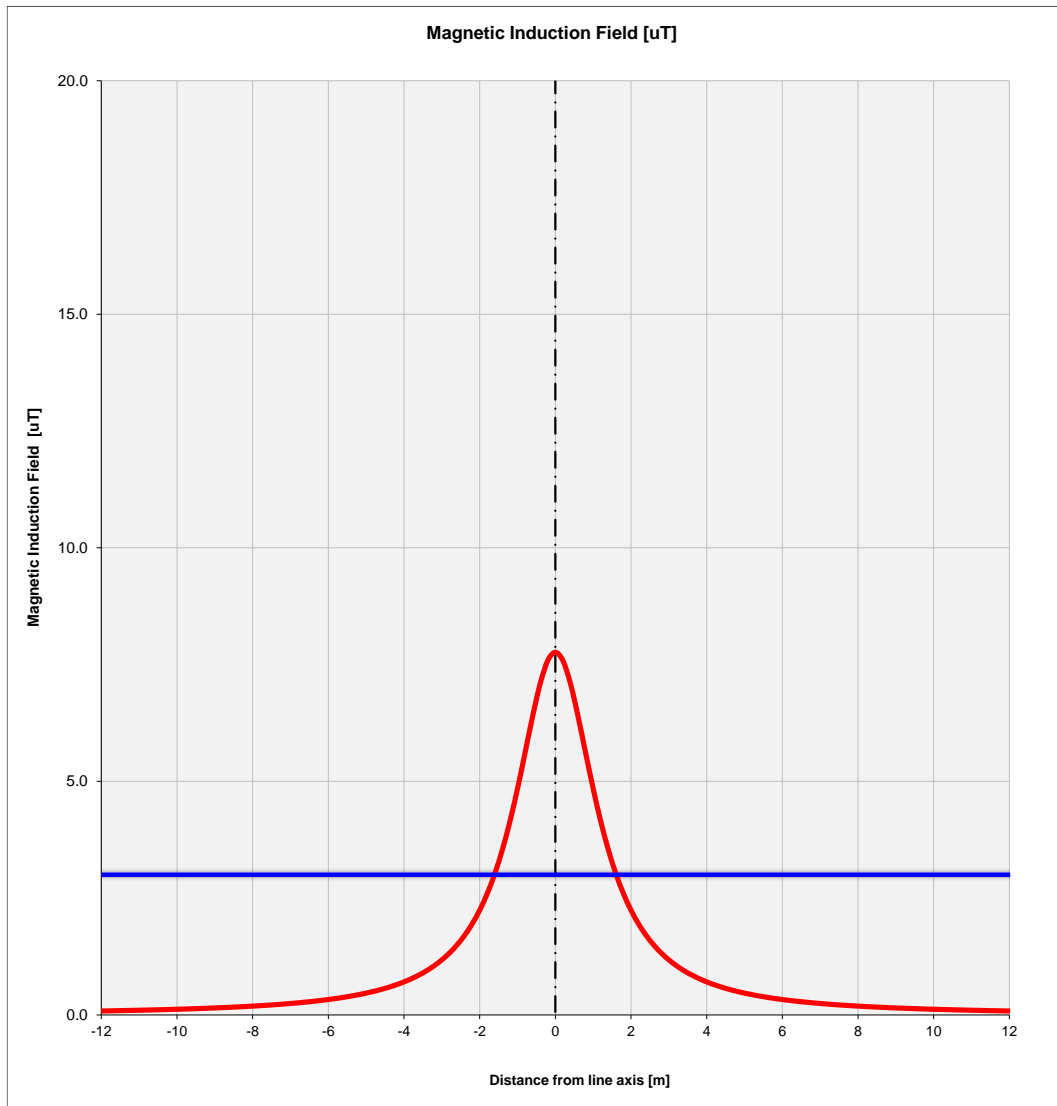
Figura 3: Andamento dell'induzione magnetica prodotta dalla linea in cavo per la sezione 2 (due terne a 36 kV)
