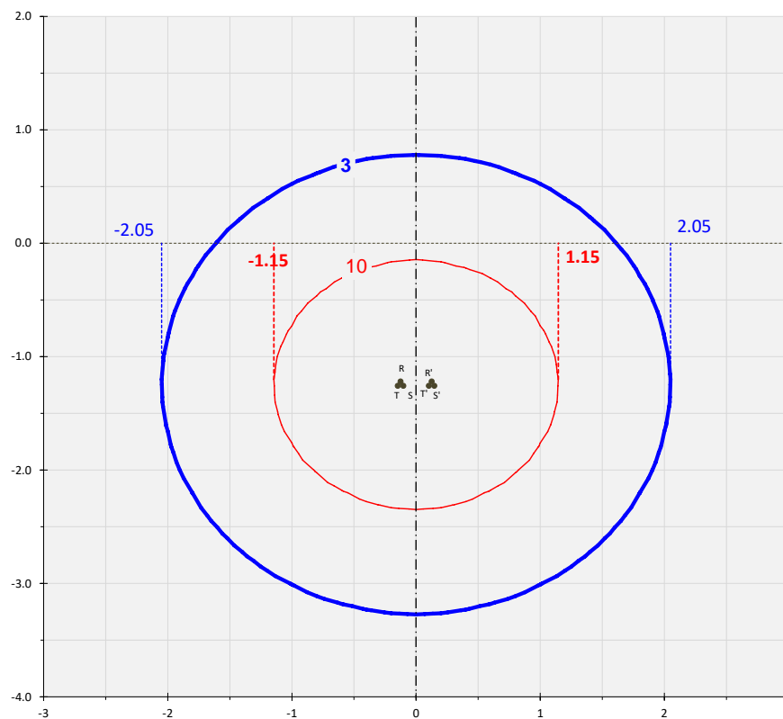
Figura 5: Curve di equilivello per il campo di induzione magnetica generato dalla linea (Sezione 2 – due terne a 36 kV)
