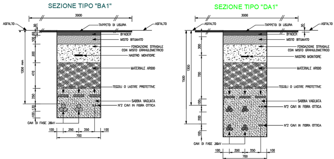
Figura 2: Sezioni tipiche di posa della linea in cavo su sede stradale
