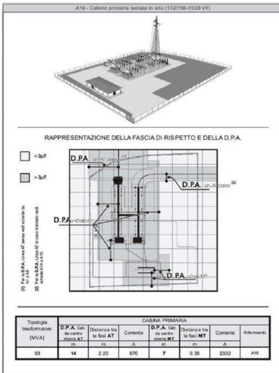
Figura 5.14. – Cabina Primaria MT/AT
