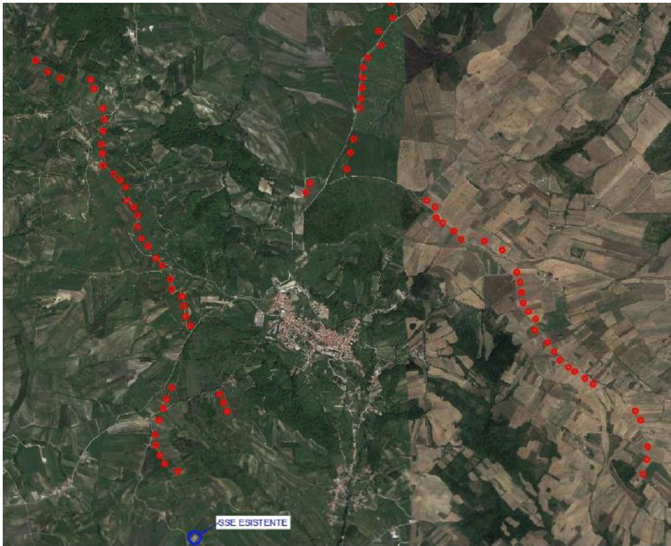
Figura 4.1. – Impianto eolico esistente da dismettere.
