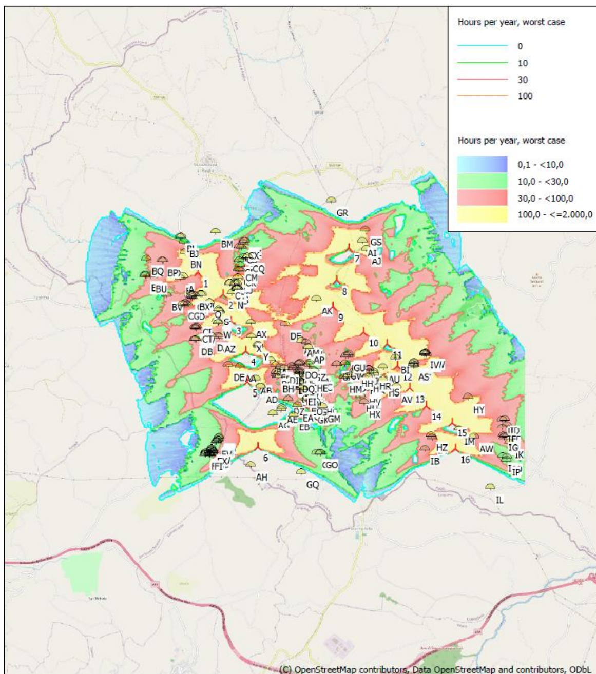
Figura 5.15. – Mappa delle aree soggette ad ombreggiamento.
