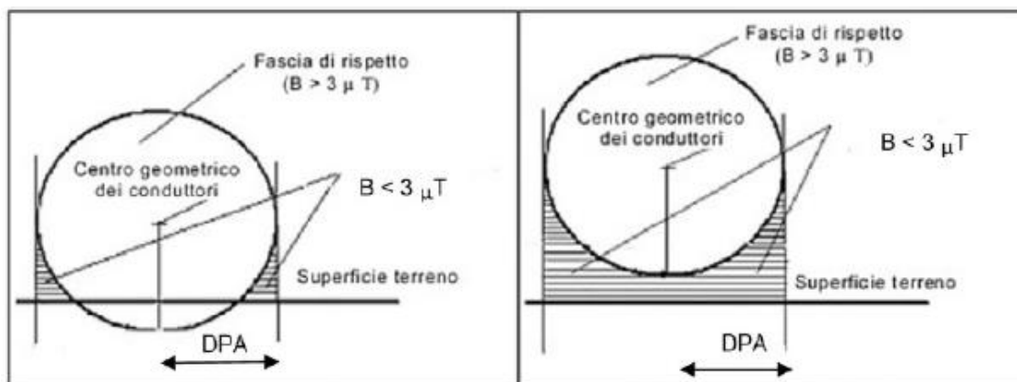
Figura 5.13. – Scheda di principio per la definizione della Fascia di Rispetto e della DPA .
