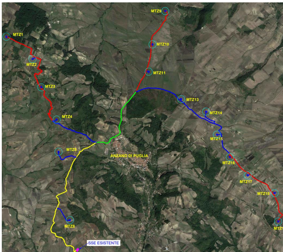
Figura 4.2. – Impianto eolico di progetto.
