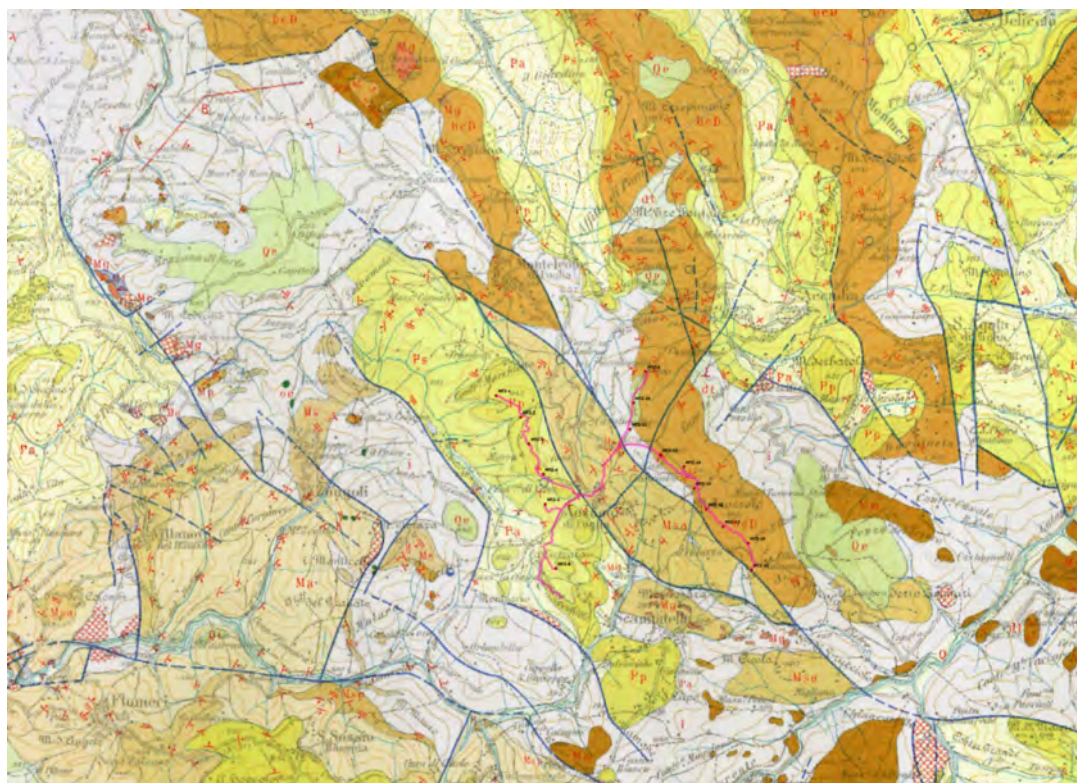
Stralcio Carta Geologica
