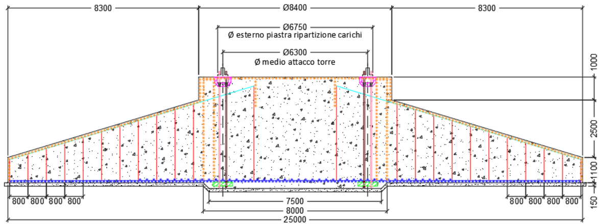
Figura 1 – Sezione fondazione di progetto
