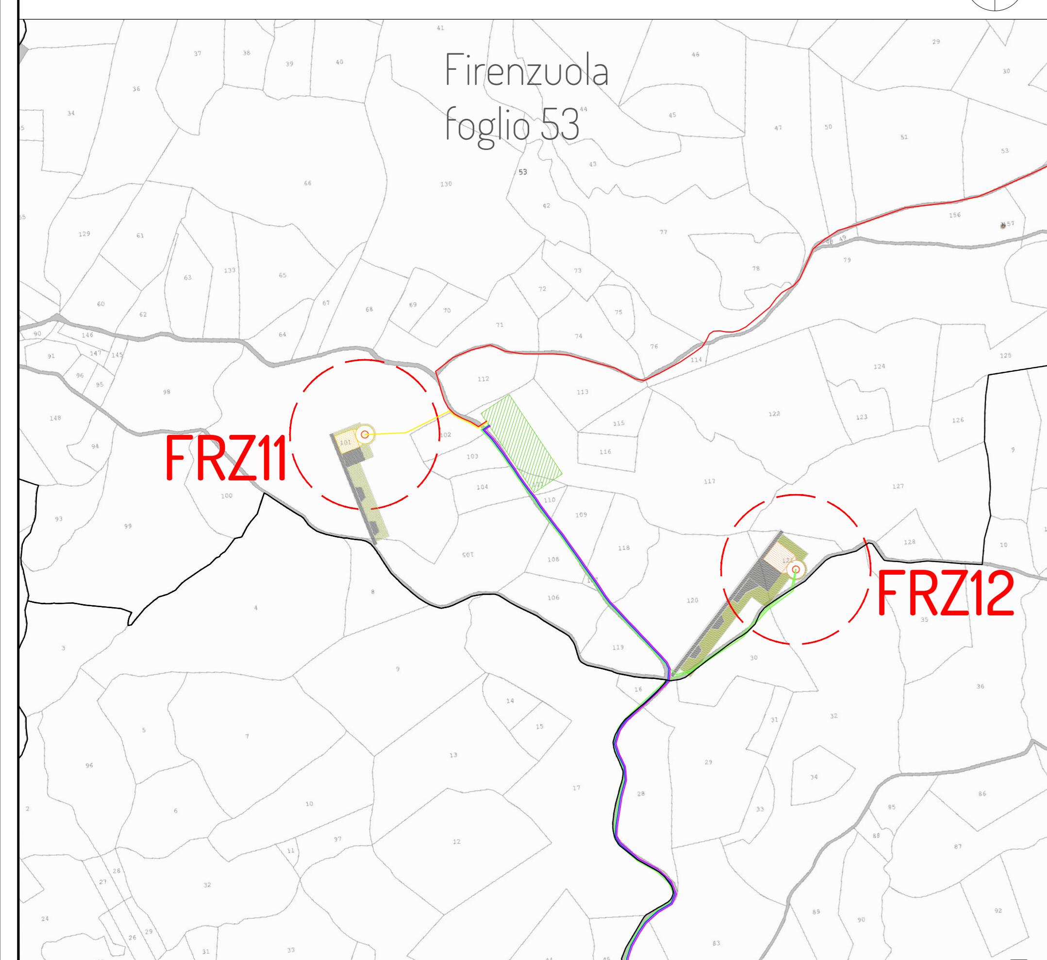
Planimetria su catastale ubicazione cabina di raccolta e BESS scala 1:4.000
