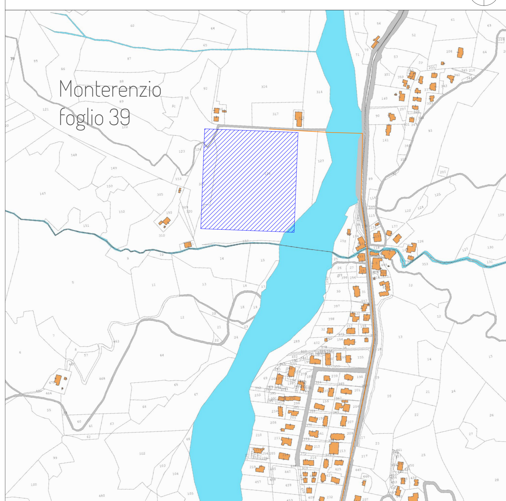
Planimetria su catastale ubicazione Stazione RTN scala 1:4.000
