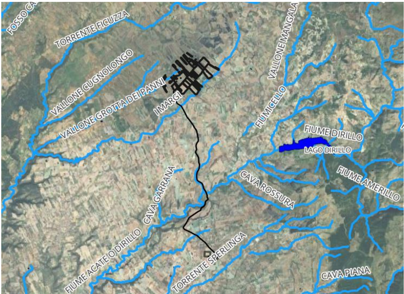
Figura 6: Idrografia dell'area di studio e dettaglio
