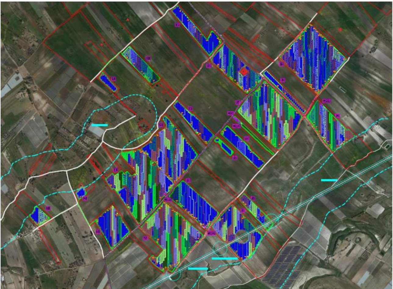
Figura 32 - Planimetria generale impianto
