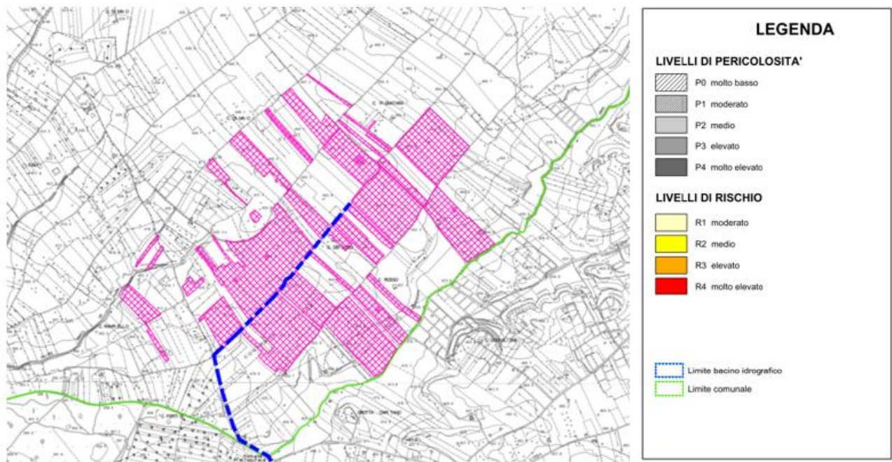
Figura 23. Stralcio Carta pericolosità e rischio geomorfologico - C451_CT2_D_AP_1011 INQUADRAMENTO SU PAI
