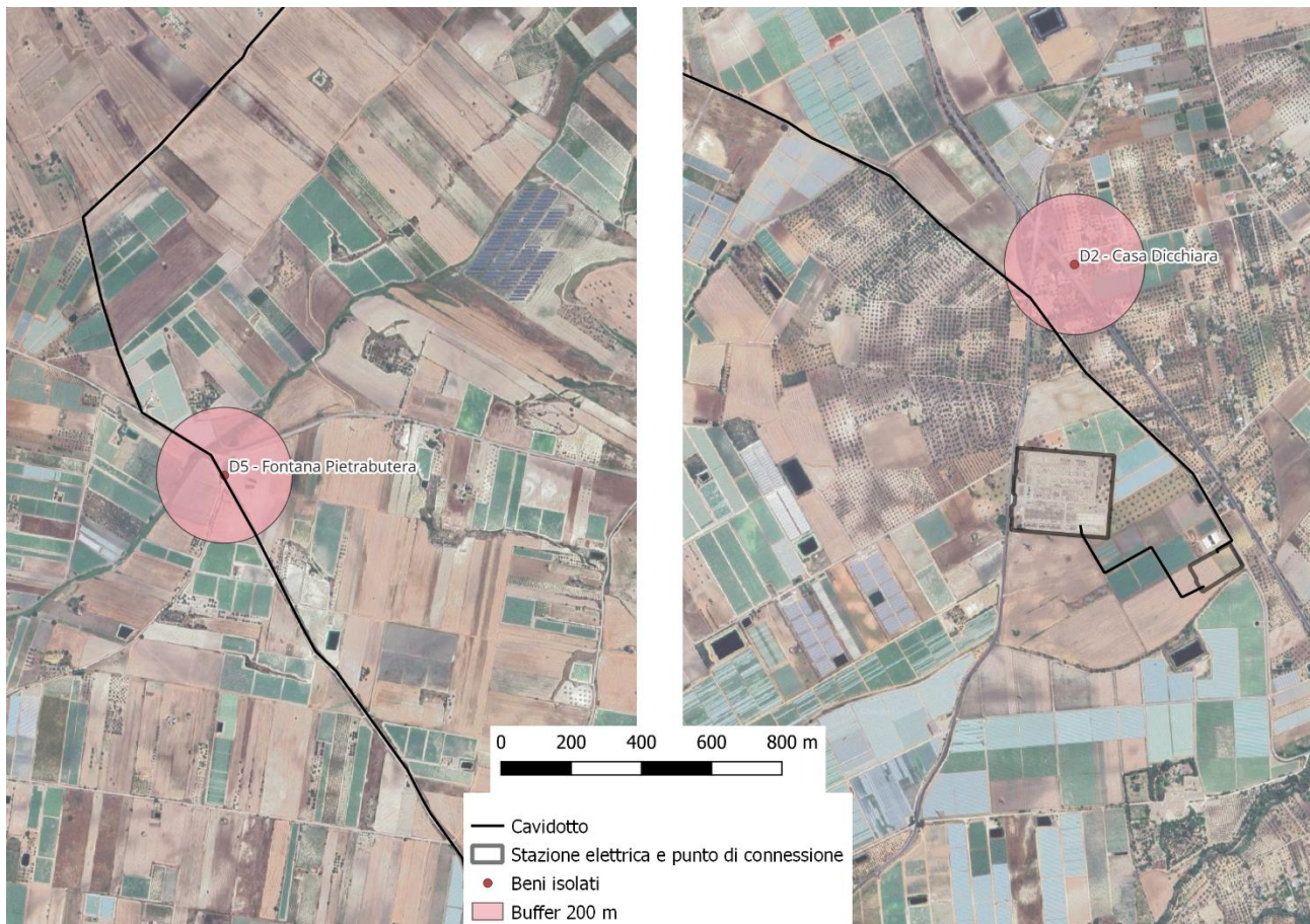
Figura 31. Beni isolati e relativo buffer su tracciato del cavidotto
