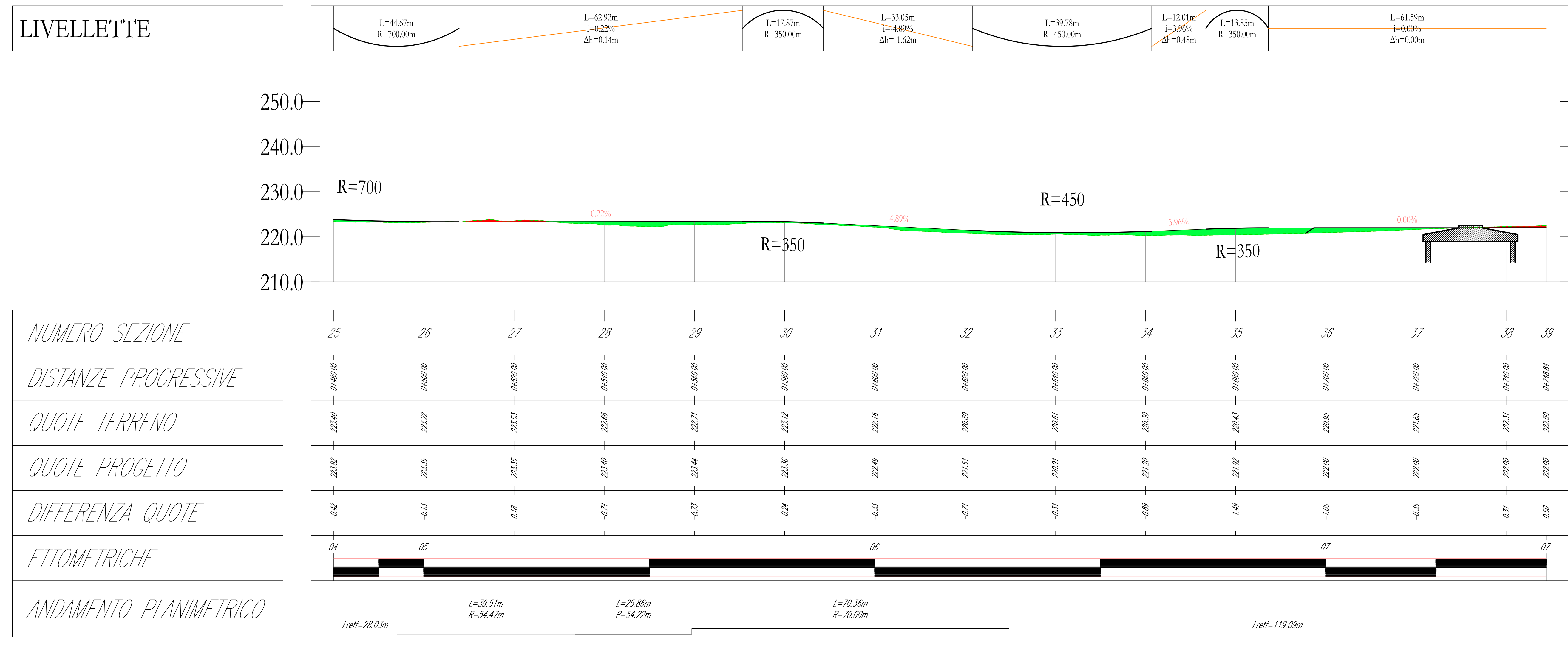
Profilo: Profilo longitudinale DU02_2 Q.Rif. : 210.00
