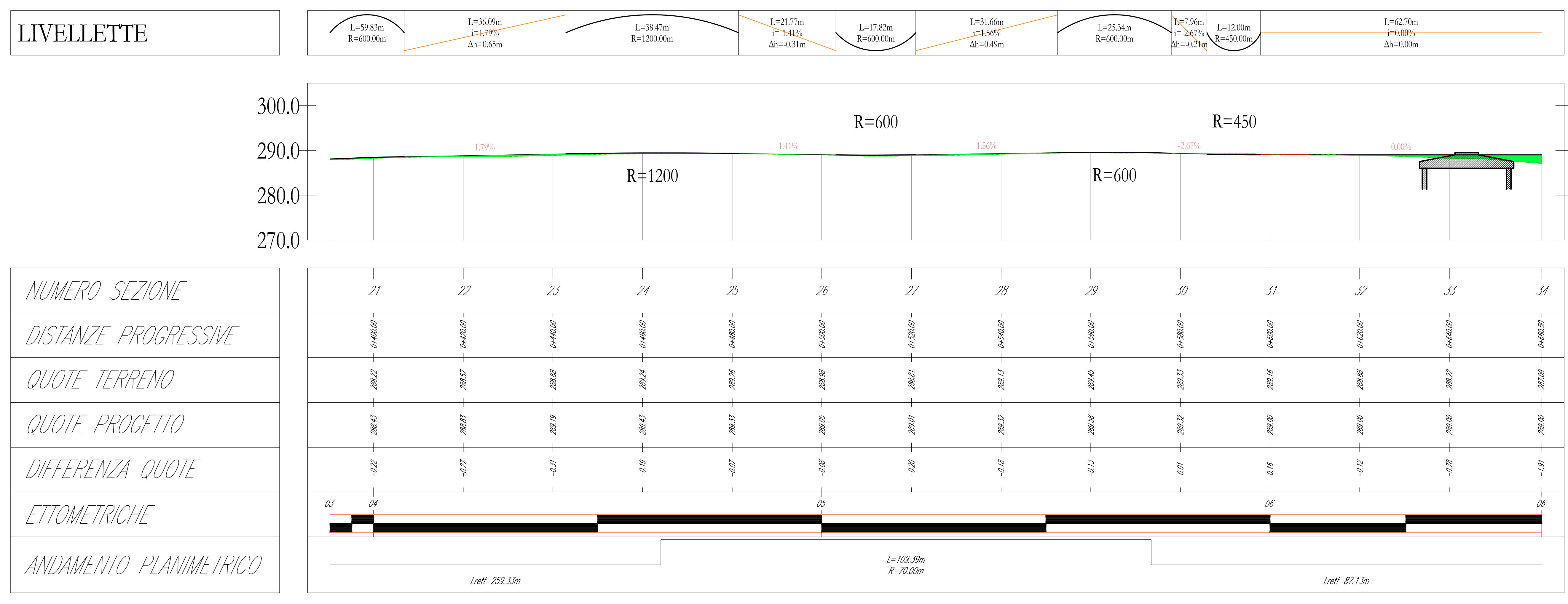
Profilo: Profilo longitudinale DU14_2 Q.Rif. : 270.00
