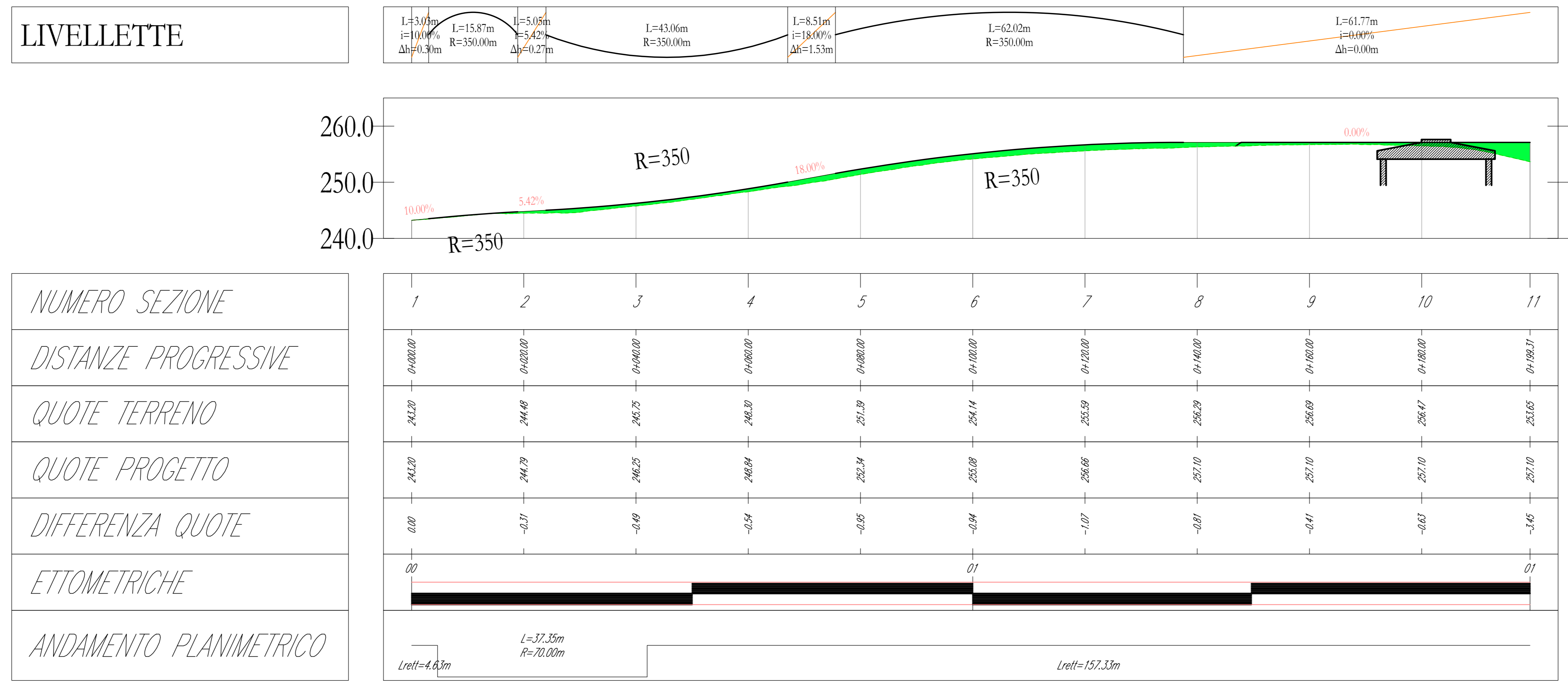
Profilo: Profilo longitudinale DU15 Q.Rif. : 240.00
