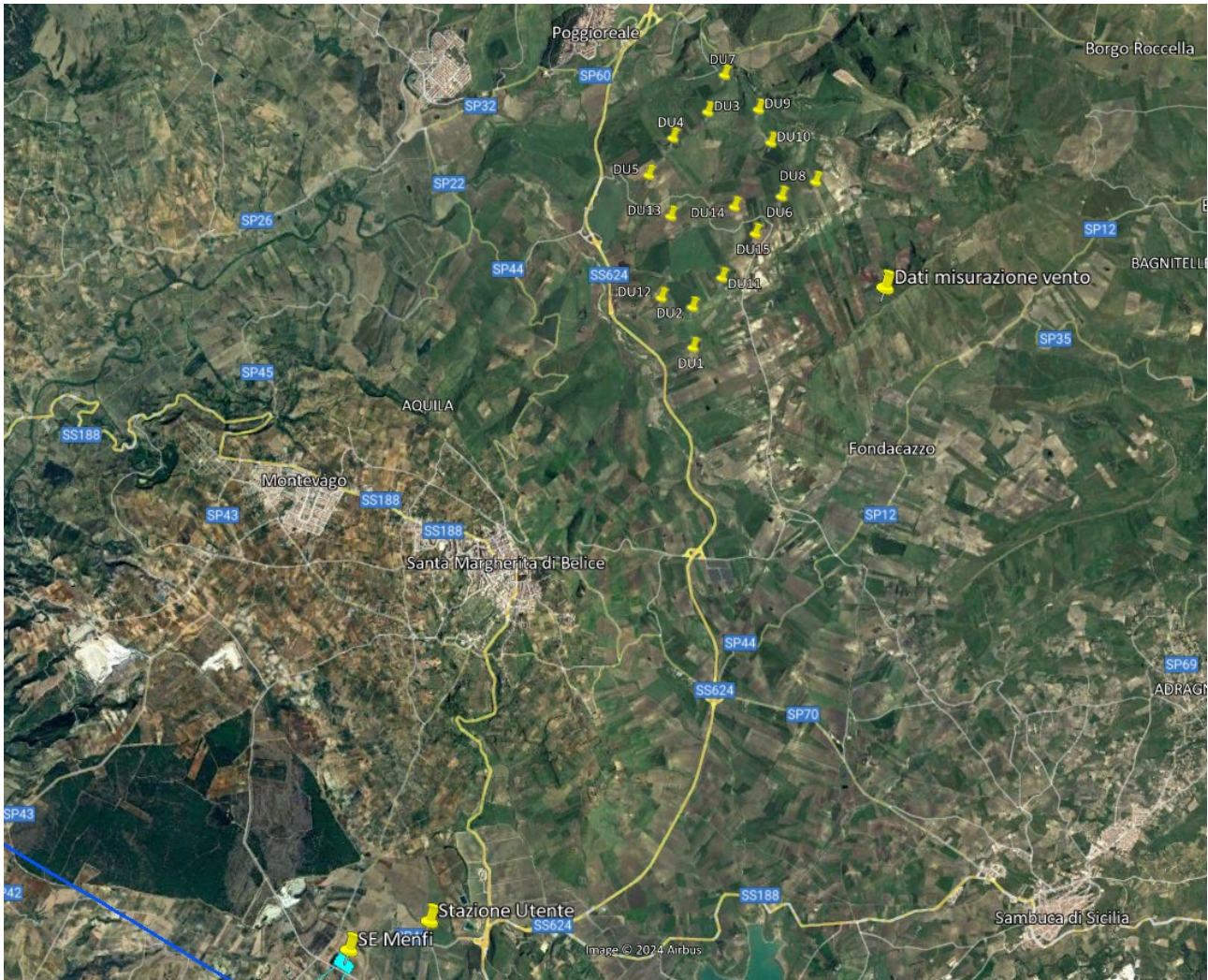
Figura 2 – Localizzazione aerogeneratori Progetto e sito di misurazione dei dati del vento (“ Dati vento ”)
