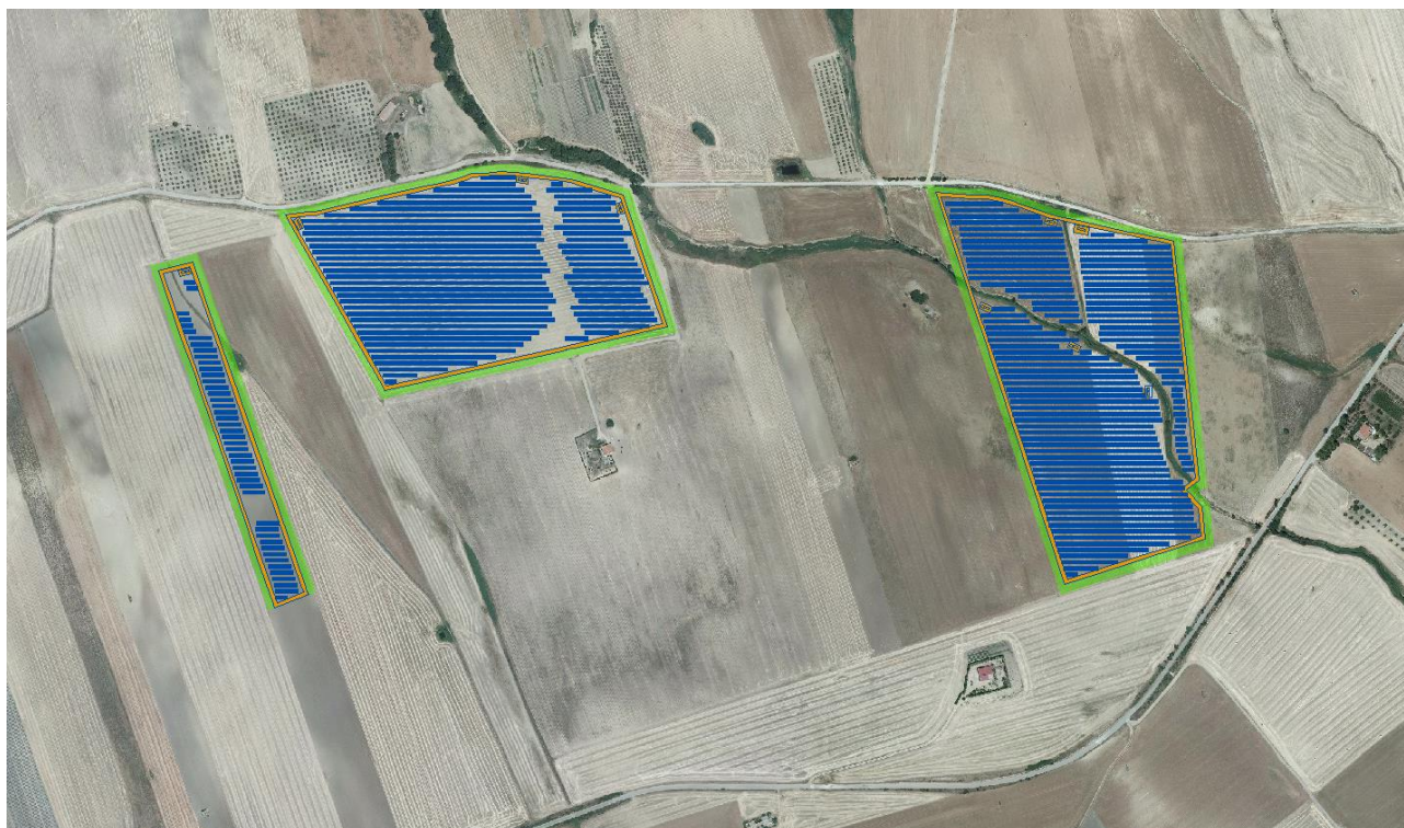
Figura 4.5. – Layout del sistema fotovoltaico con supporti fissi.
