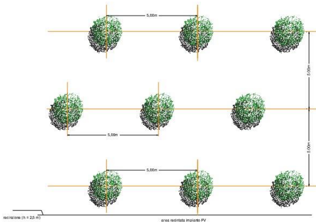
figura 3.19_ stralcio planimetria oliveto
