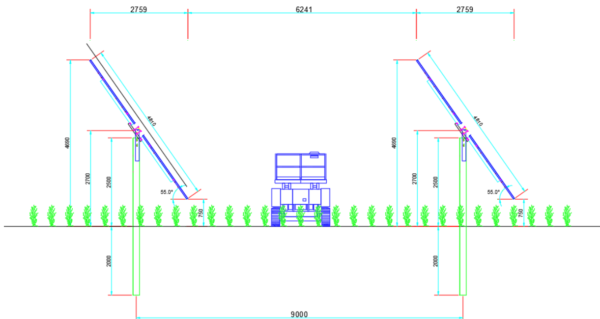
Figura 3.2b. – Tracker - configurazione orizzontale
