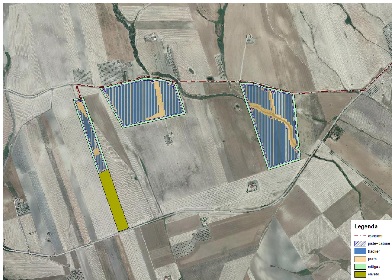
Figura 3.1 – Area di progetto con indicazione degli interventi agronomici e posizionamento dei moduli fotovoltaici.
