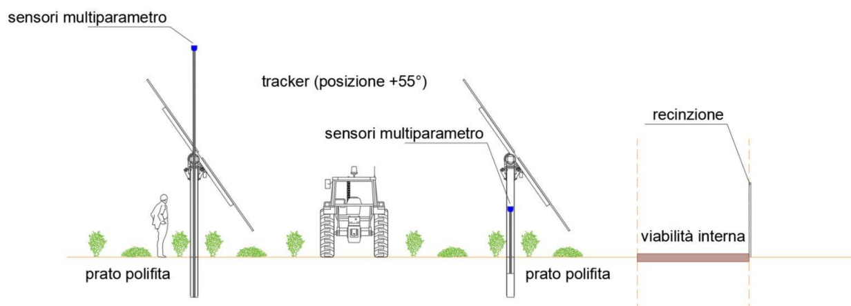
Figura 4.10. – Schema di posizionamento delle stazioni meteorologiche interne al campo agrivoltaico.
