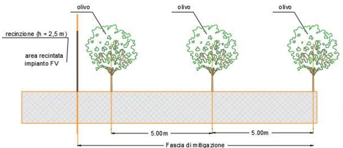
figura 3.20: stralcio sezione oliveto
