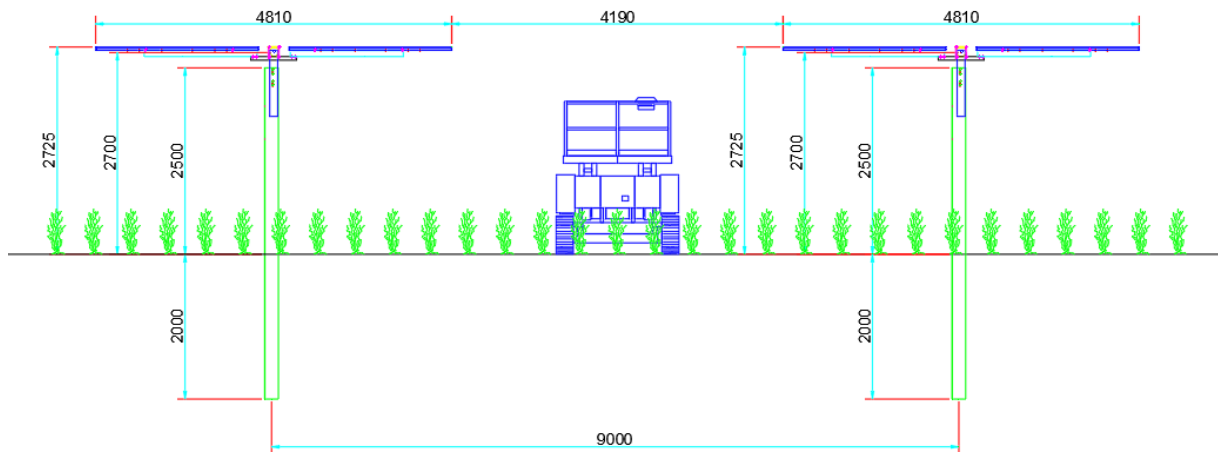
Figura 3.2a. – Tracker - configurazione orizzontale
