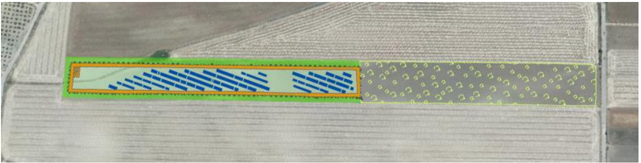
Figura 4.2a. – Layout del sistema agrivoltaico con tracker – dettaglio
