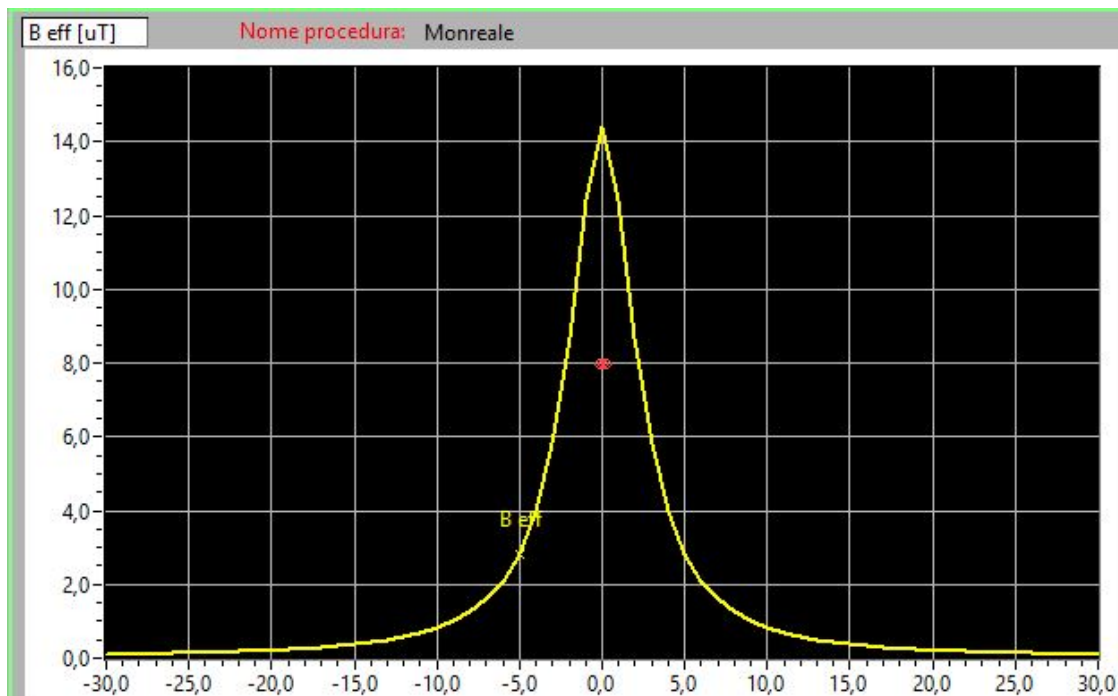
Profilo laterale del campo magnetico al suolo con cavi posizionati ad una profondità di 1,5 m
