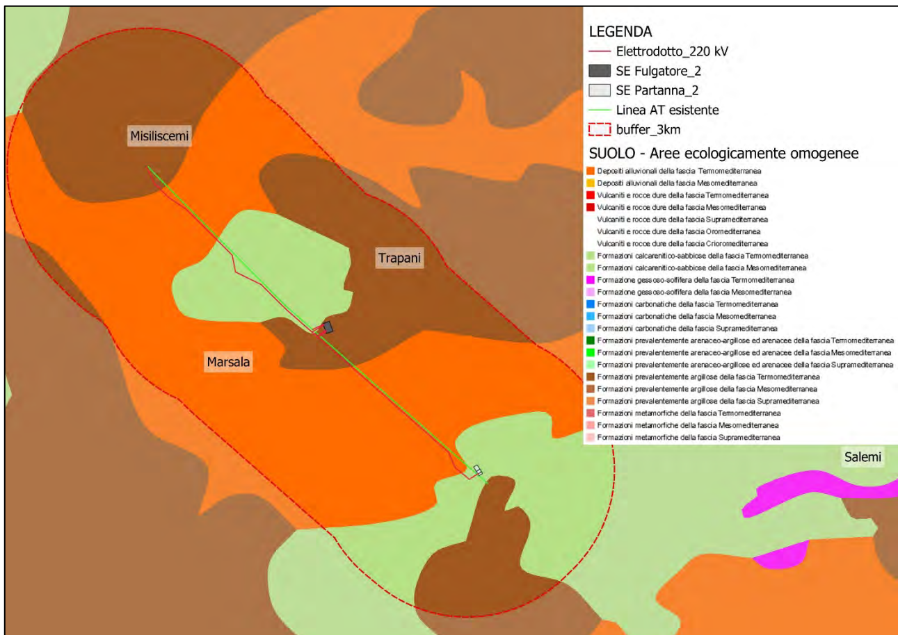
Figura 8 – Aree ecologicamente omogenee
