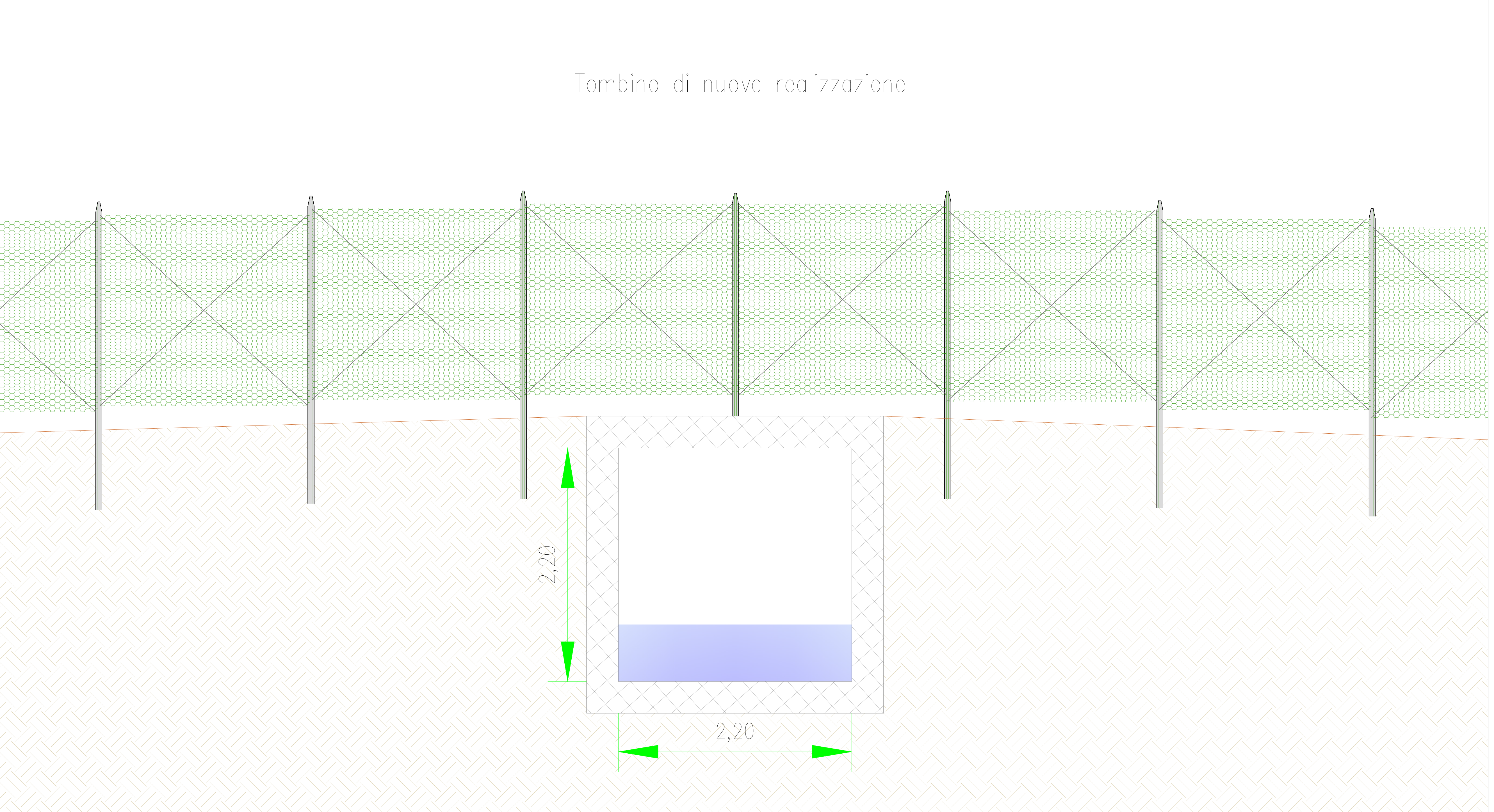
Sezione B-B' - Scala 1:20
