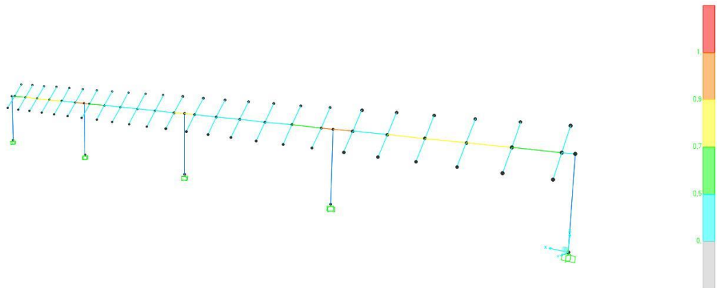
Figura 9 – coefficienti di sicurezza verifica a taglio (elementi cold formed) configurazione 55°
