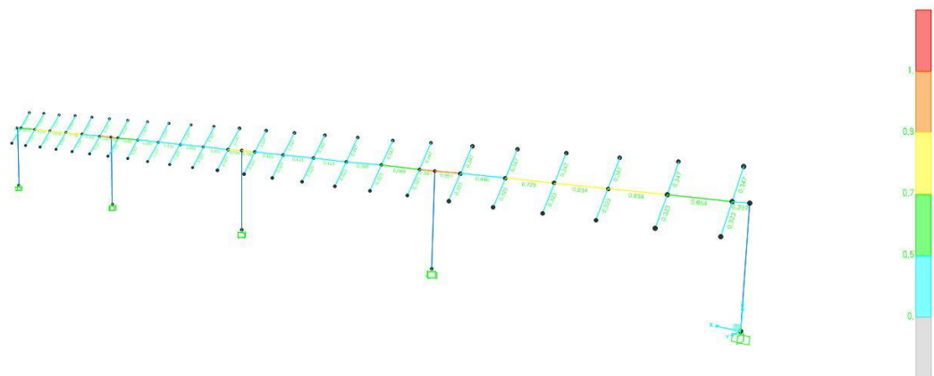
Figura 7 – coefficienti di sicurezza verifica di instabilità (elementi cold formed) configurazione 55°
