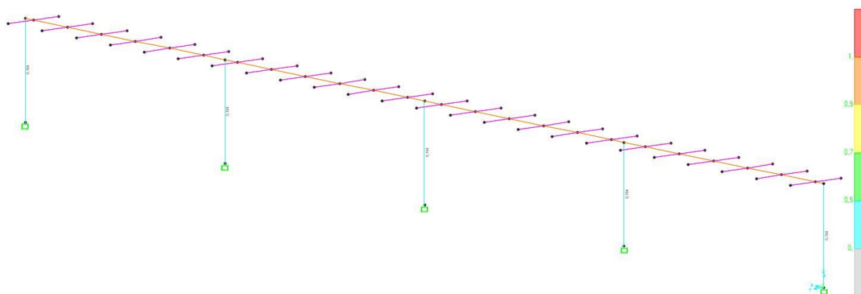
Figura 2 – coefficienti di sicurezza verifica di instabilità configurazione 0°
