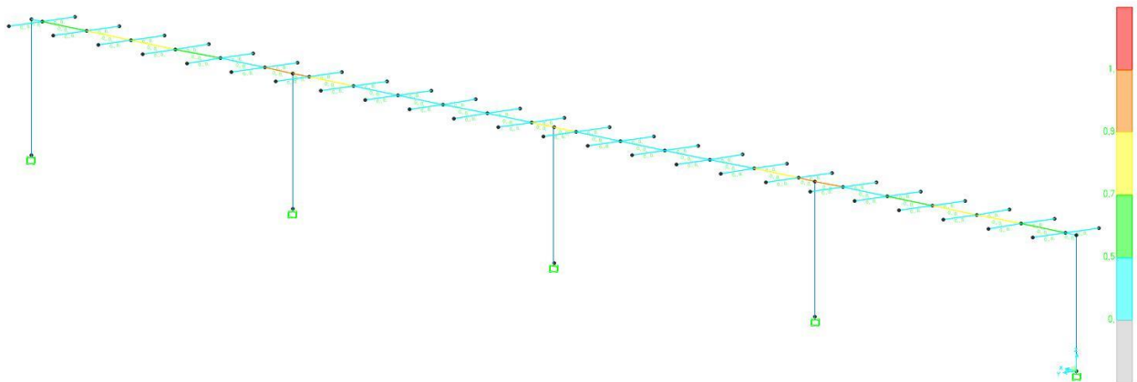
Figura 5 – coefficienti di sicurezza verifica a taglio (elementi cold formed) configurazione 0°
