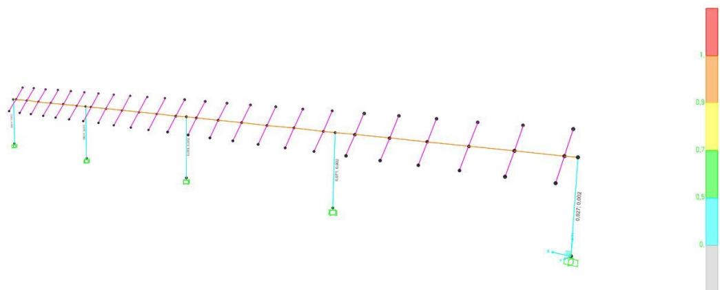
Figura 8 – coefficienti di sicurezza verifica a taglio configurazione 55°
