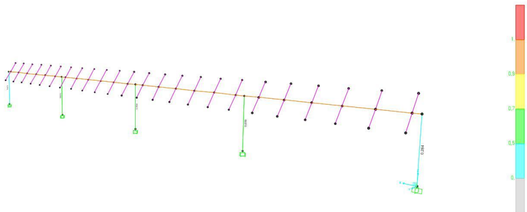
Figura 6 – coefficienti di sicurezza verifica di instabilità configurazione 55°
