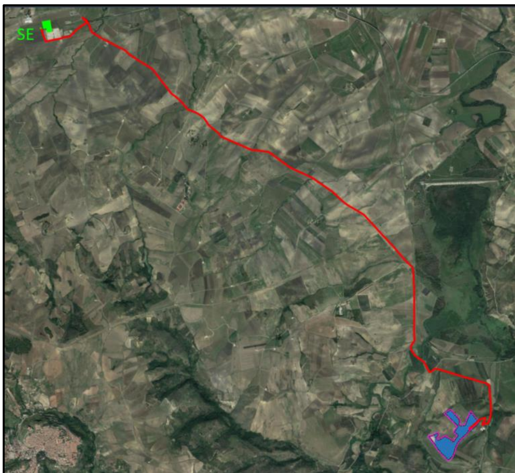
Figura 8 - Connessione alla RTN: confine catastale (in magenta), percorso del cavidotto (in rosso), futuro ampliamento della SE (in verde)
