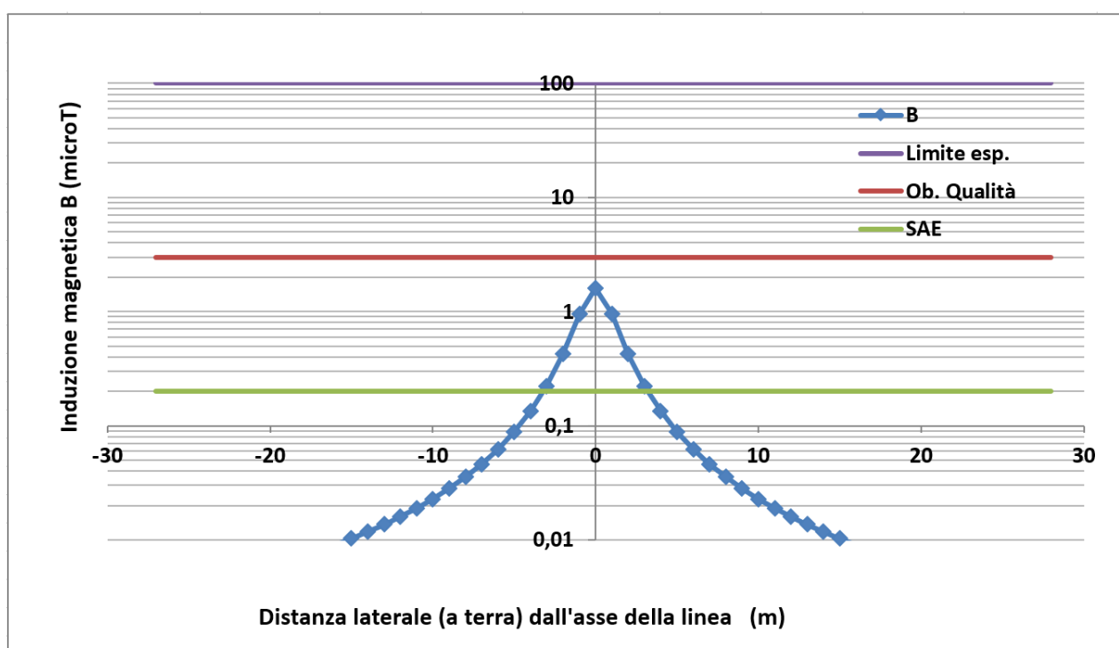
Figura 7 – Campo di induzione magnetica B ( \mu T ) generato dal cavidotto interno AT del progetto agrivoltaico in relazione ai limiti di esposizione e obiettivo di qualità-R1
