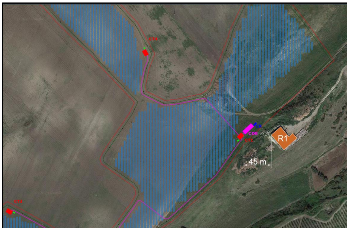
Figura 6 – Layout dell’impianto con indicazione dei ricettori potenzialmente sensibili
