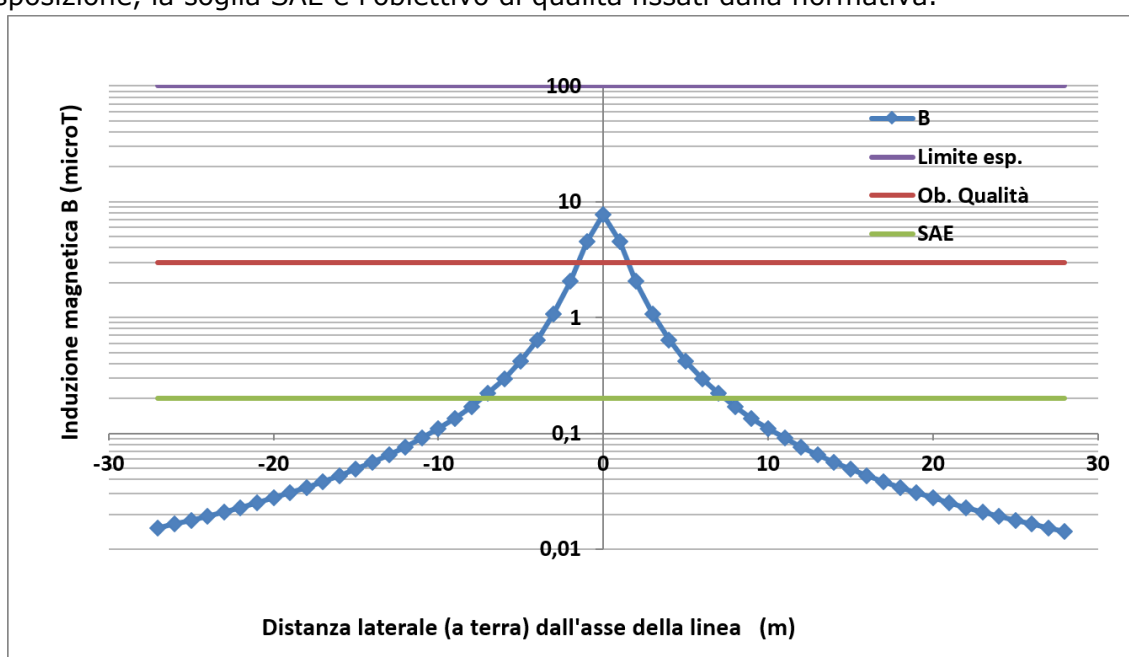
Figura 16 – Campo di induzione magnetica B ( \mu T ) generato dal cavidotto singolo di evacuazione AT del progetto agrivoltaico in relazione ai limiti di esposizione e obiettivo di qualità.
