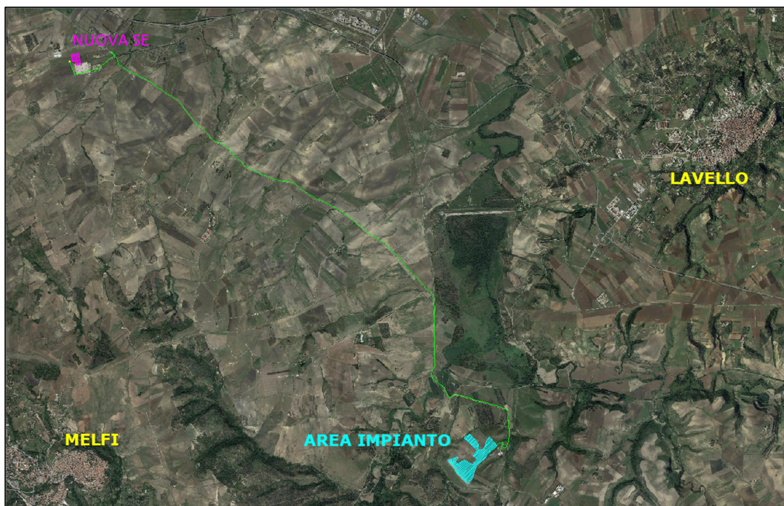
Figura 1 – Stralcio su ortofoto dell’impianto FV con indicazione della connessione al futuro ampliamento della SE “Melfi” – 36 kV
