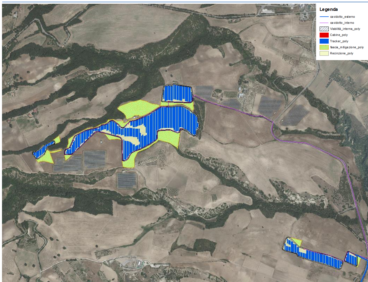
Figura 3.1. – Area di progetto con indicazione degli interventi agronomici e posizionamento dei moduli fotovoltaici.
