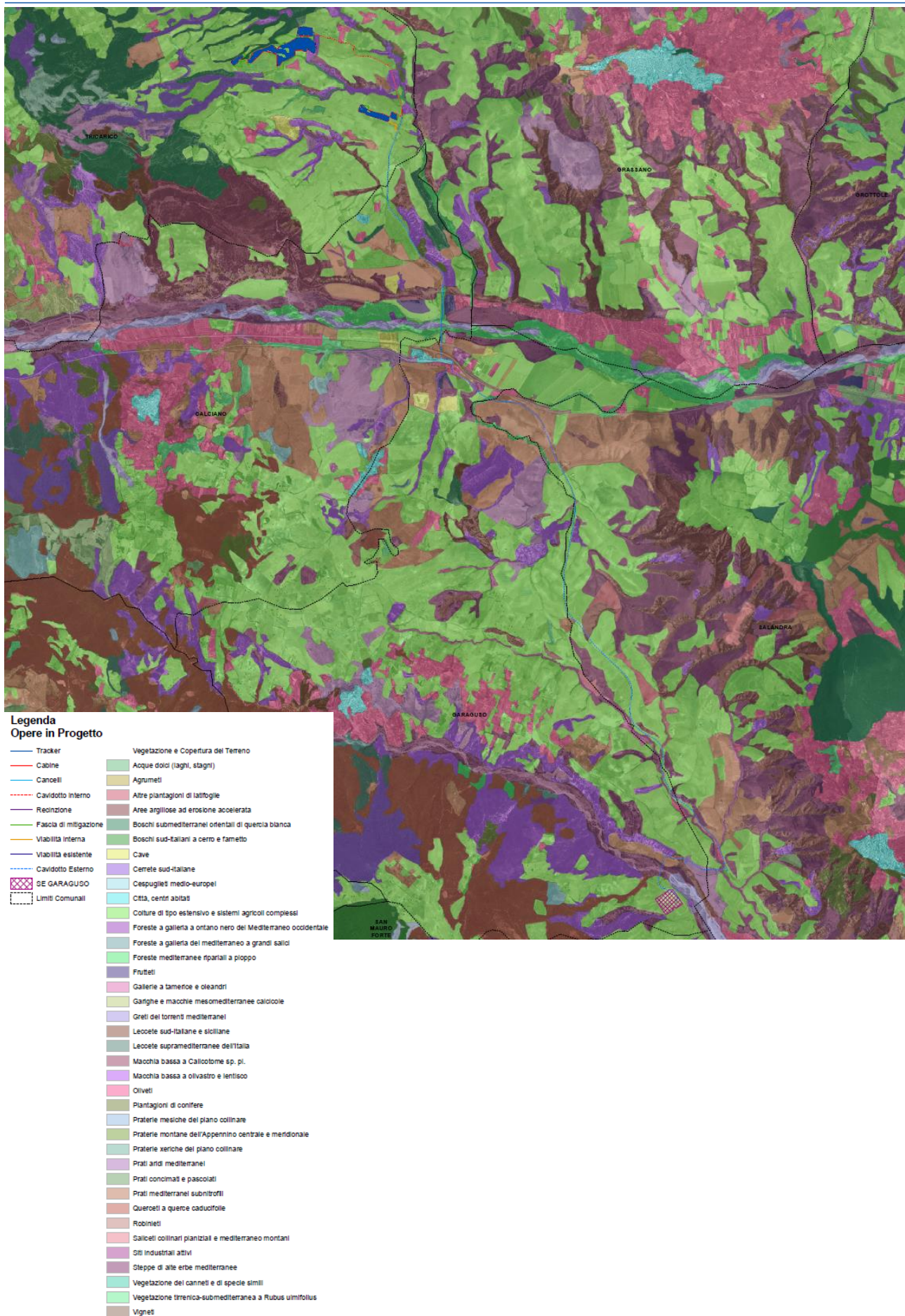
Figura 3.14. – Vegetazione e copertura area vasta.
