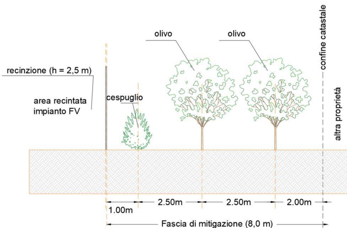
Figura 3.3. – Stralcio di sezione dell'area perimetrale dell'impianto – siepe e doppio filare di olivo.
