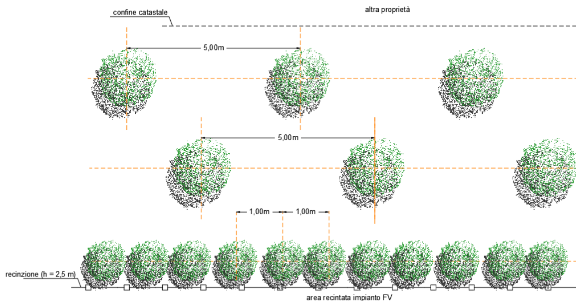
Figura 3.2. – Siepe polispecifica (planimetria di progetto) – siepe e doppio filare di olivo.
