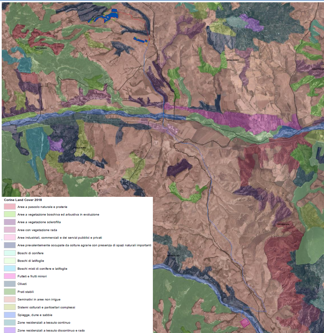
Figura 3.6. – Stralcio Carta Uso del Suolo Corine Land Cover 2018.
