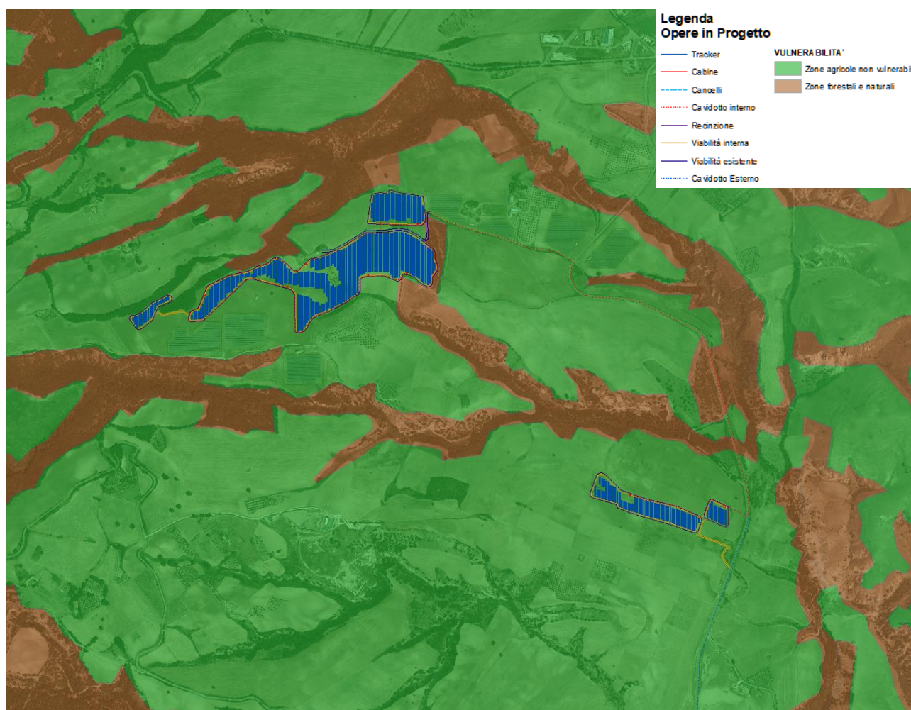
Figura 3.5. – Carta della Vulnerabilità da nitrati di origine agricola.
