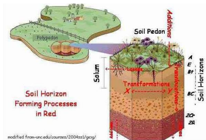
Figura 3.7. – Unità rappresentativa del suolo – PEDON.
