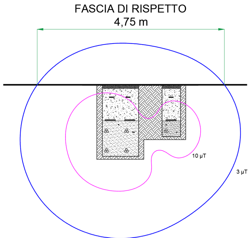
Figura 8: Curve Equicampo - Cinque Terne cavi AT - Tratta 5
