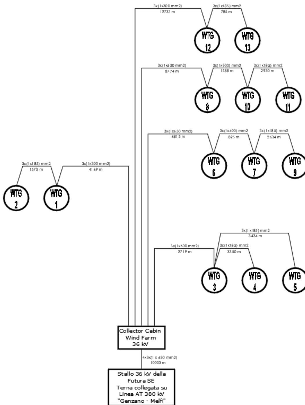
Figura 1 - Schema di collegamento tra WTG - SE Terna
