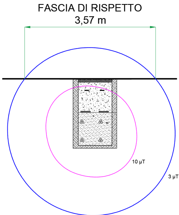
Figura 7: Curve Equicampo –Quattro Terne cavi AT – Tratta 4
