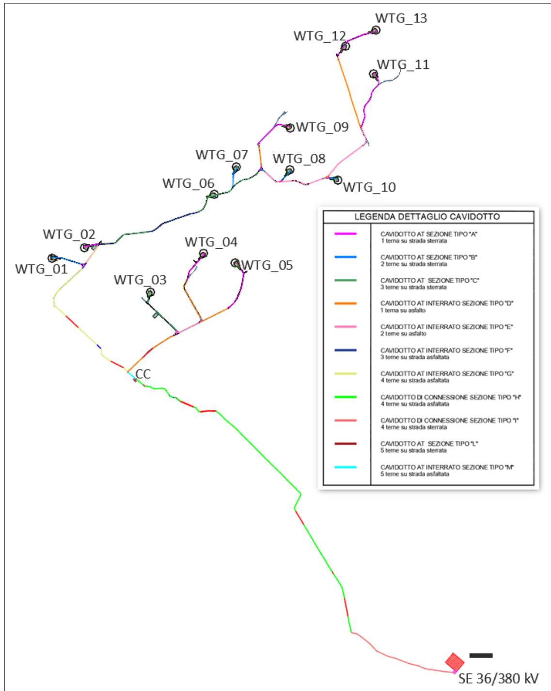
Figura 2: Caratteristiche cavi AT interno ed esterno parco
