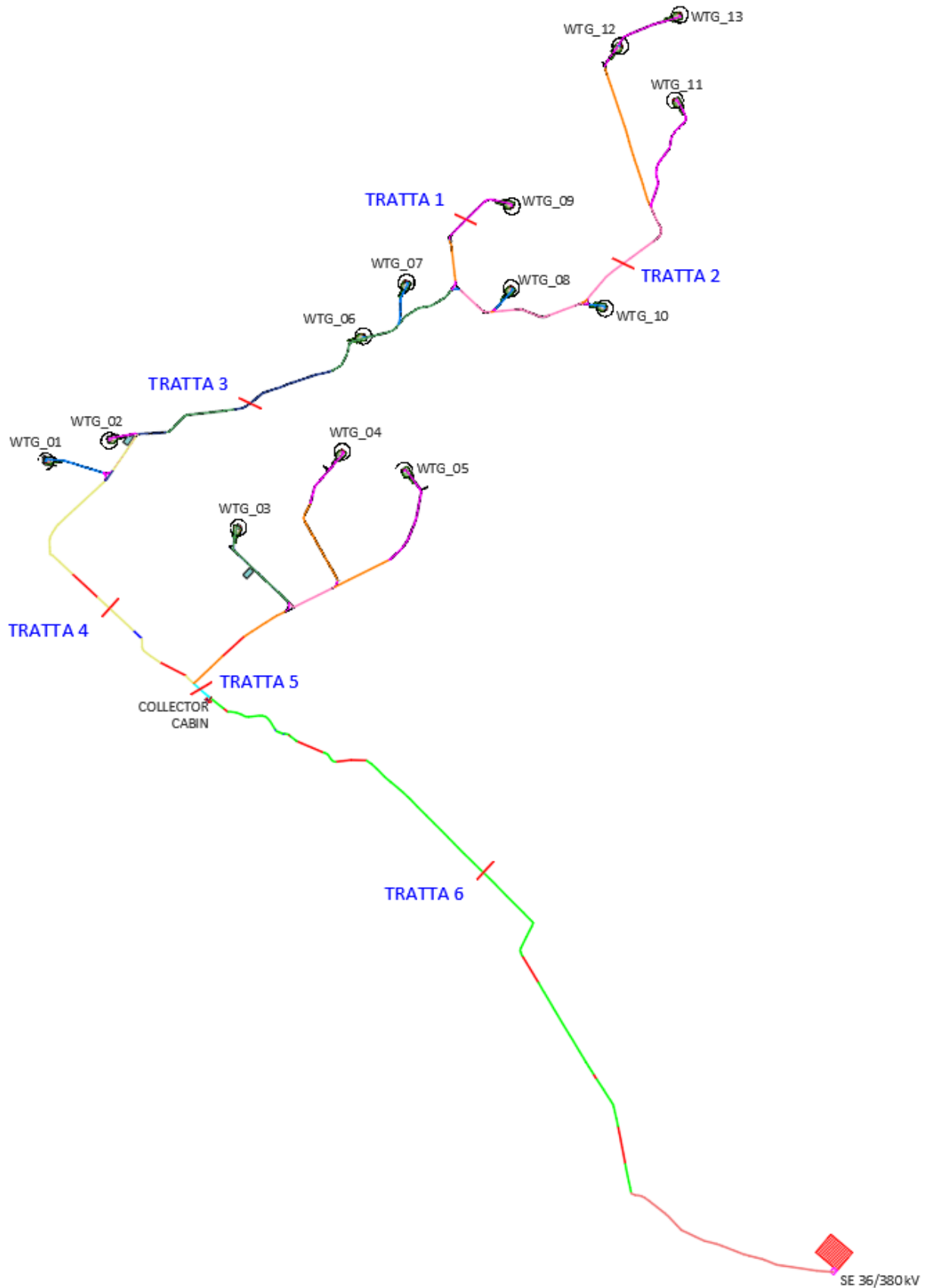
Figura 3: Tratte del percorso del cavo AT studiate ai fini della valutazione dei campi magnetici
