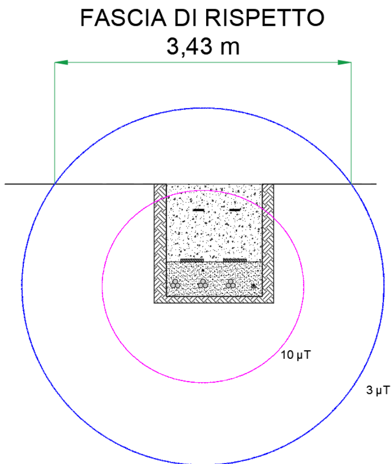
Figura 6: Curve Equicampo - Tre Terne cavi AT - Tratta 3
