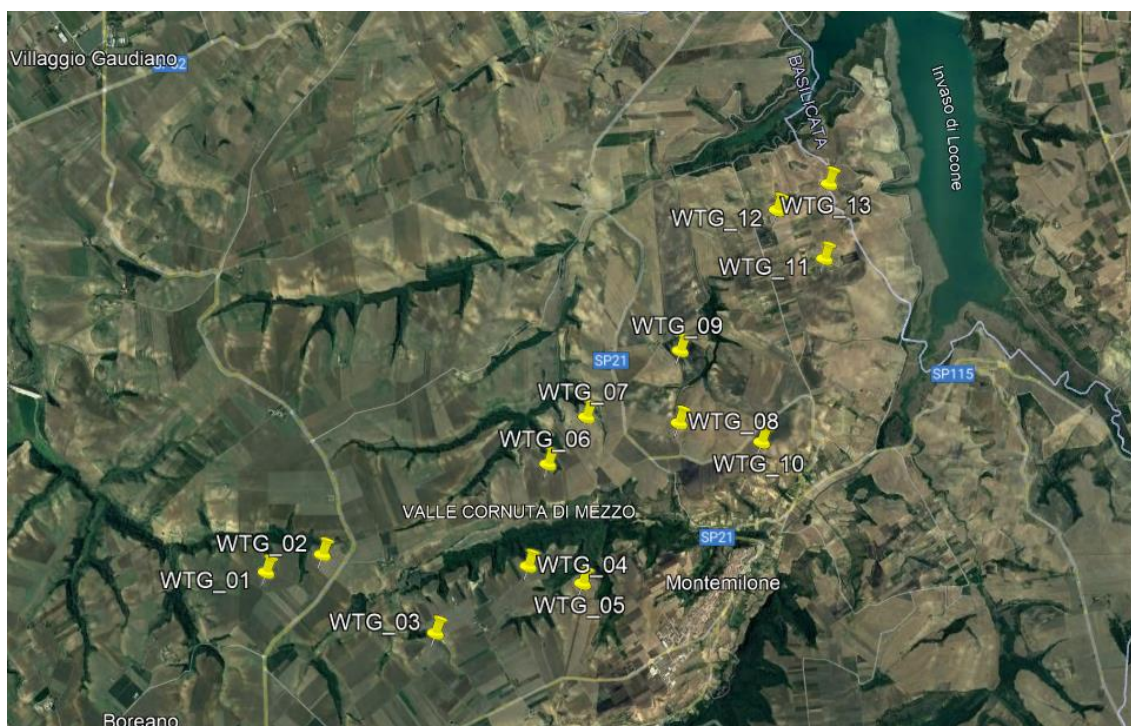
Figura 1: Layout d'impianto su Ortofoto
