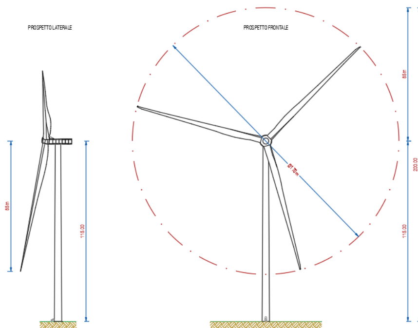
Figura 2: Vista e caratteristiche dell'aerogeneratore di riferimento
