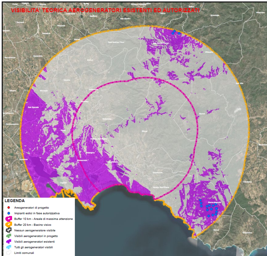
Figura 5 - Mappa dell'intervisibilità dei soli aerogeneratori esistenti ed autorizzati - Metodo 2
