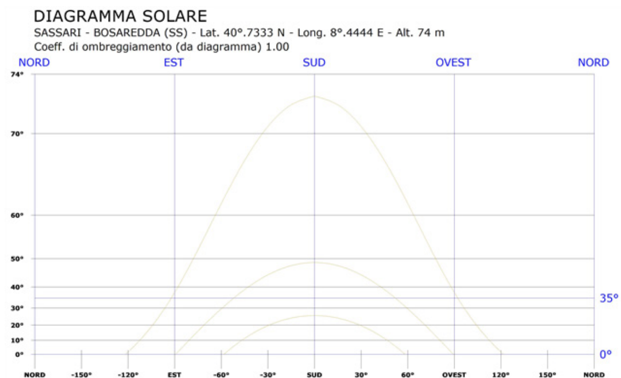
Fig. 2: Diagramma solare
