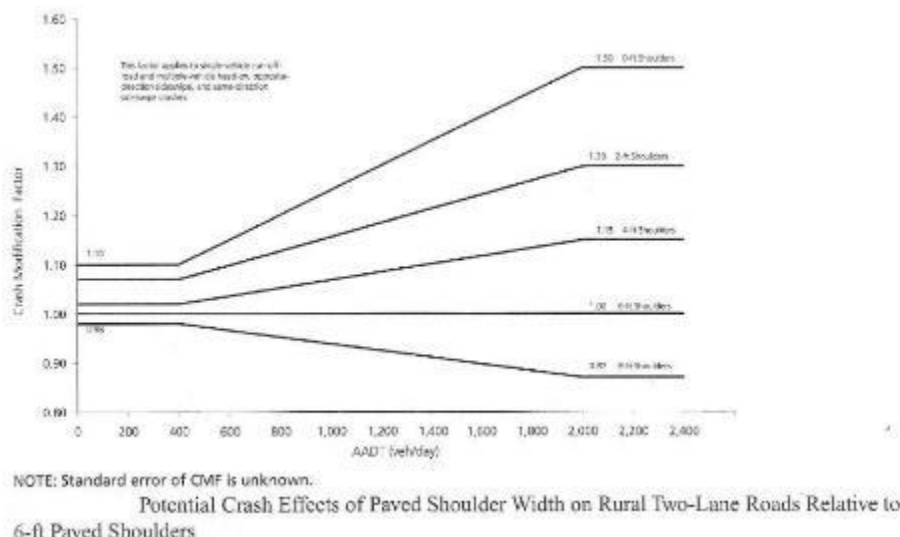
Figura 12: Variazione dei CMF per interventi sulle banchine laterali al variare del traffico (HSM 2010)
