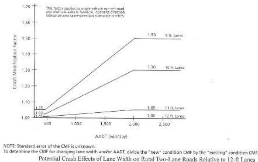
Figura 13: Variazione dei CMF per interventi sulla larghezza delle corsie di marcia (HSM 2010).
