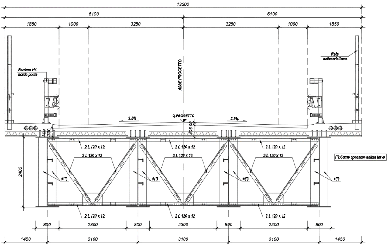
Figura 11: Sezione tipo in viadotto
