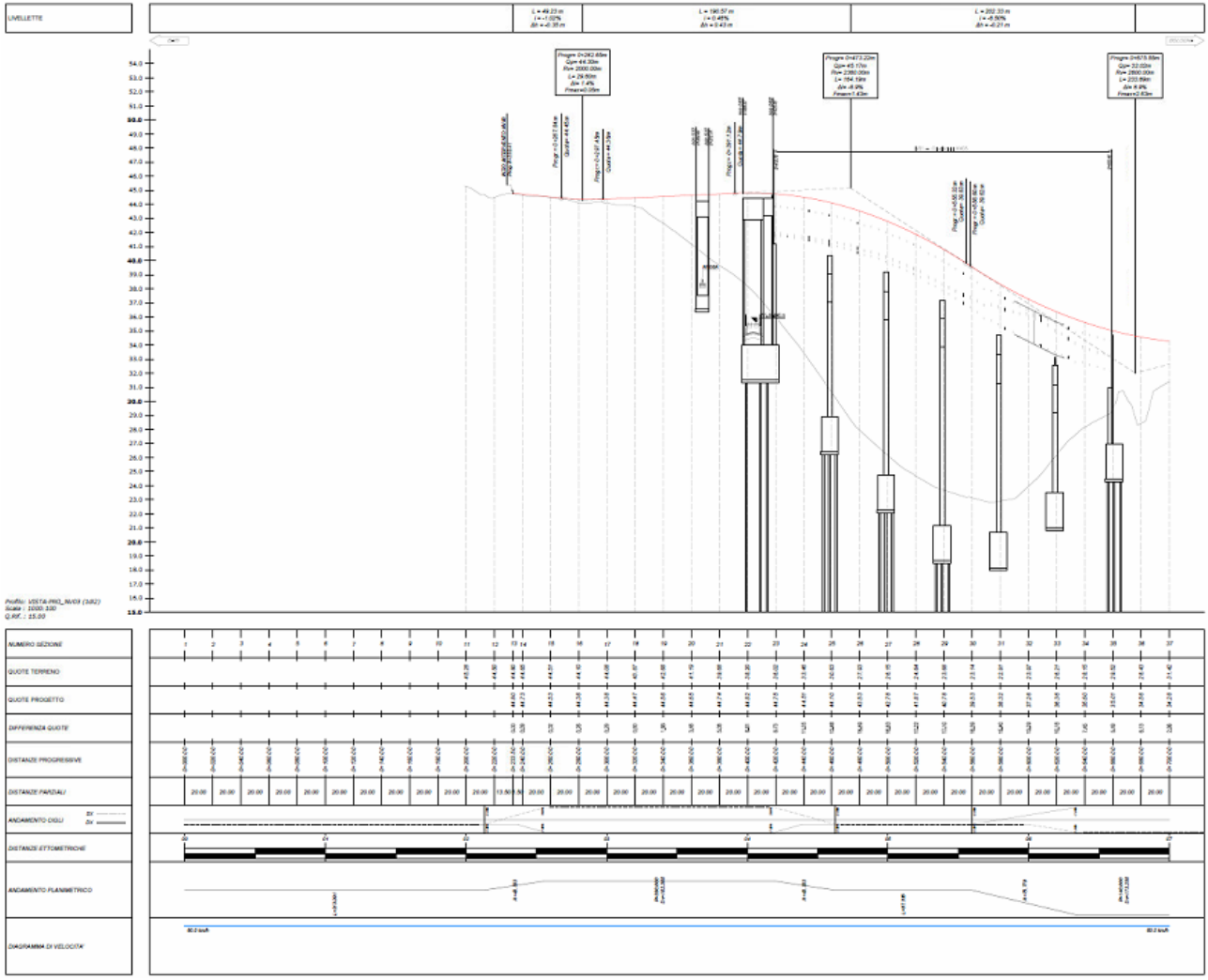
Figura 6: Profilo di progetto (Tav. 1 di 2)
