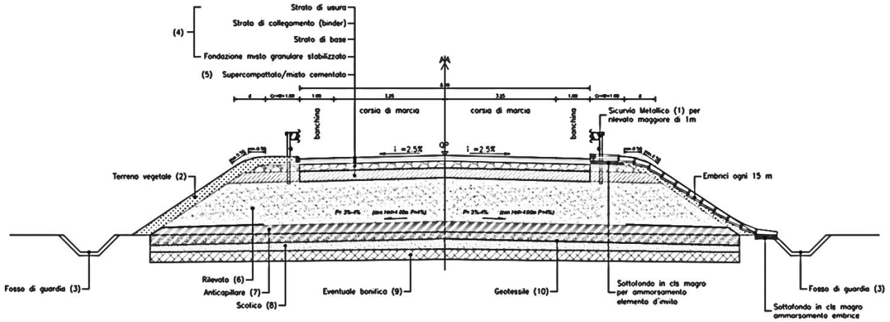
Figura 10 - Sezione tipo in rilevato
