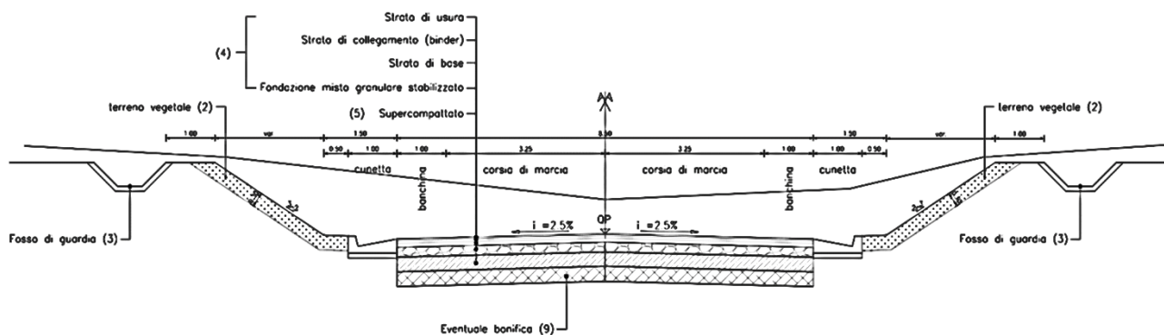
Figura 9 - Sezione tipo in trincea
