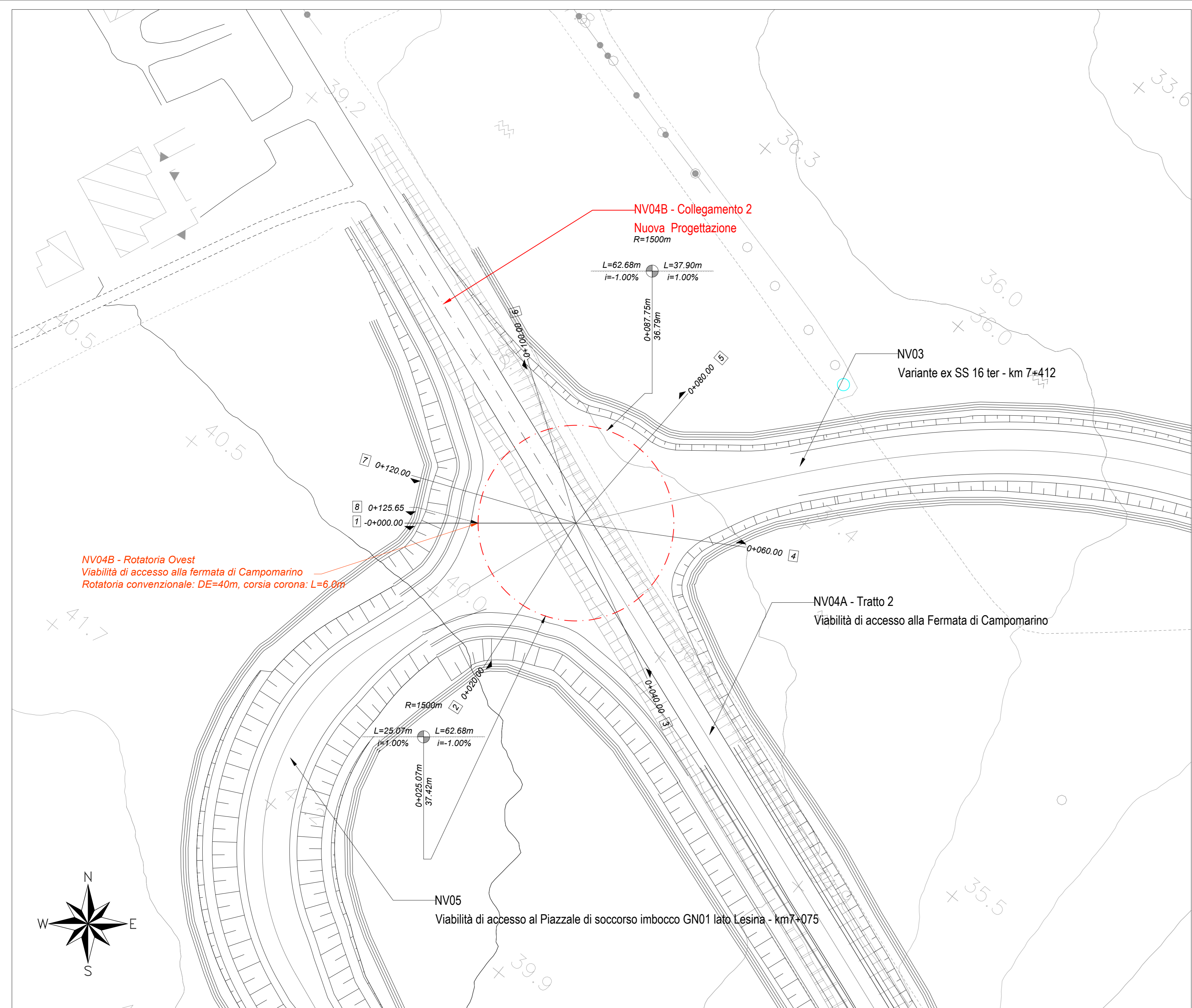
NV04B - Rotatoria Ovest - Planimetria di tracciamento
