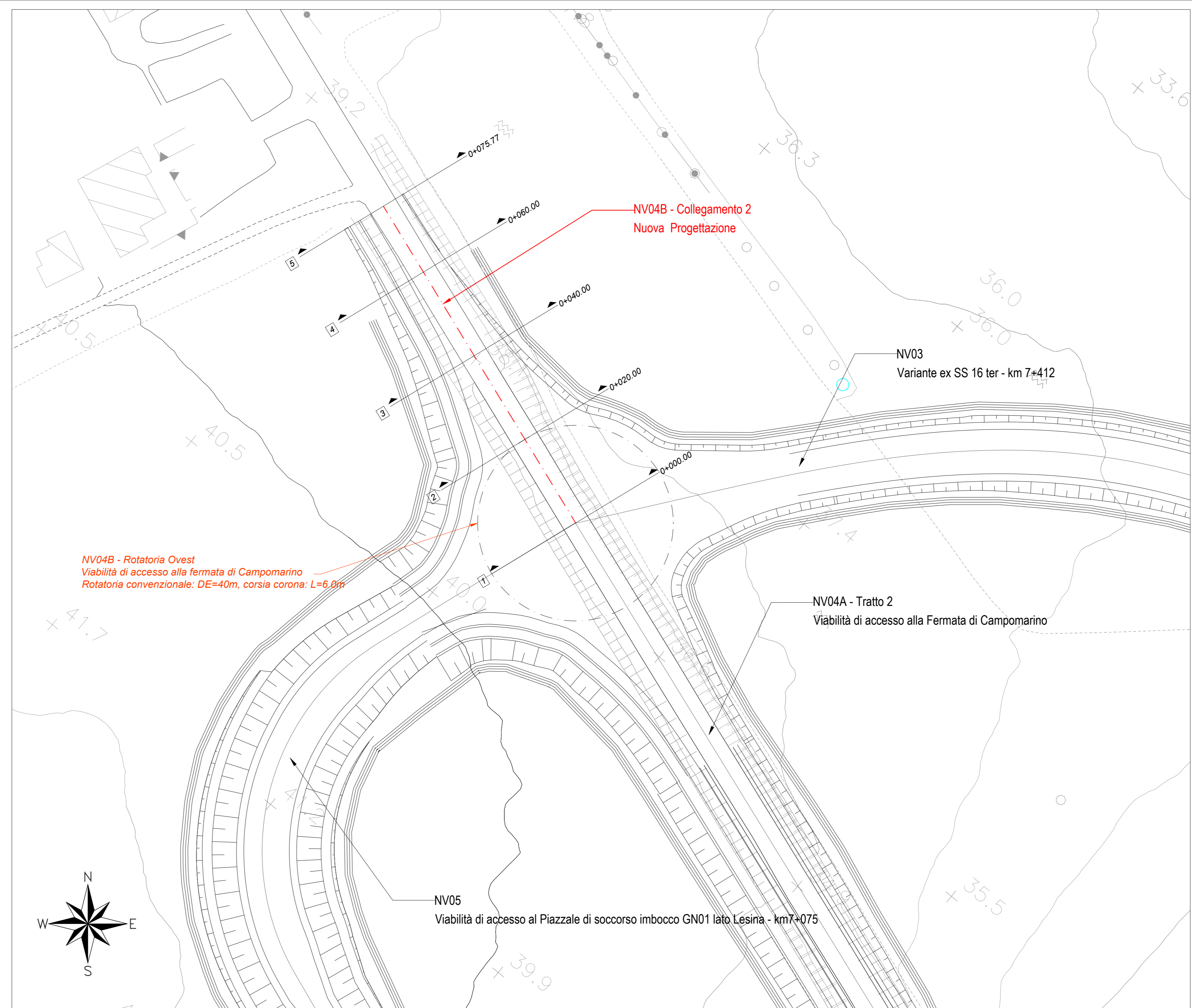
NV04B - Collegamento 2 - Planimetria di tracciamento
