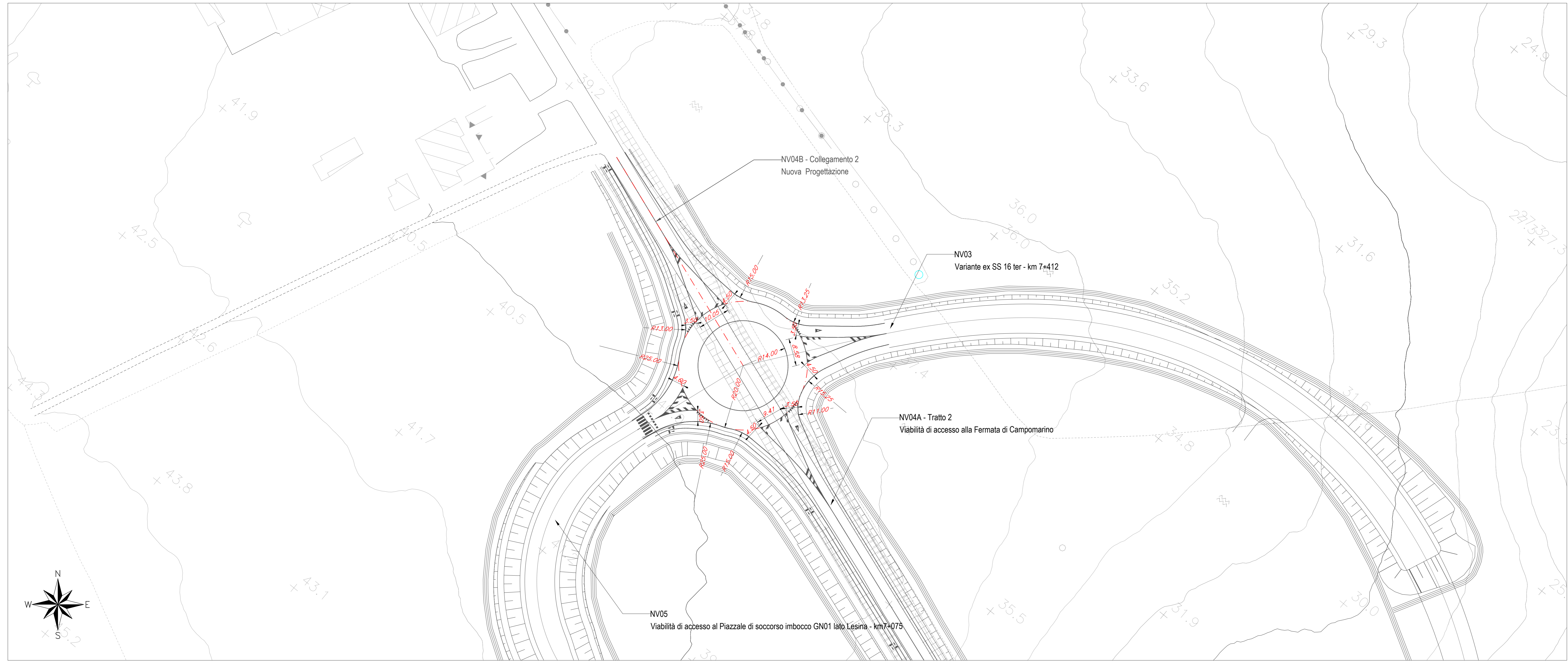
NV04B - Rotatoria Ovest - Planimetria di progetto
