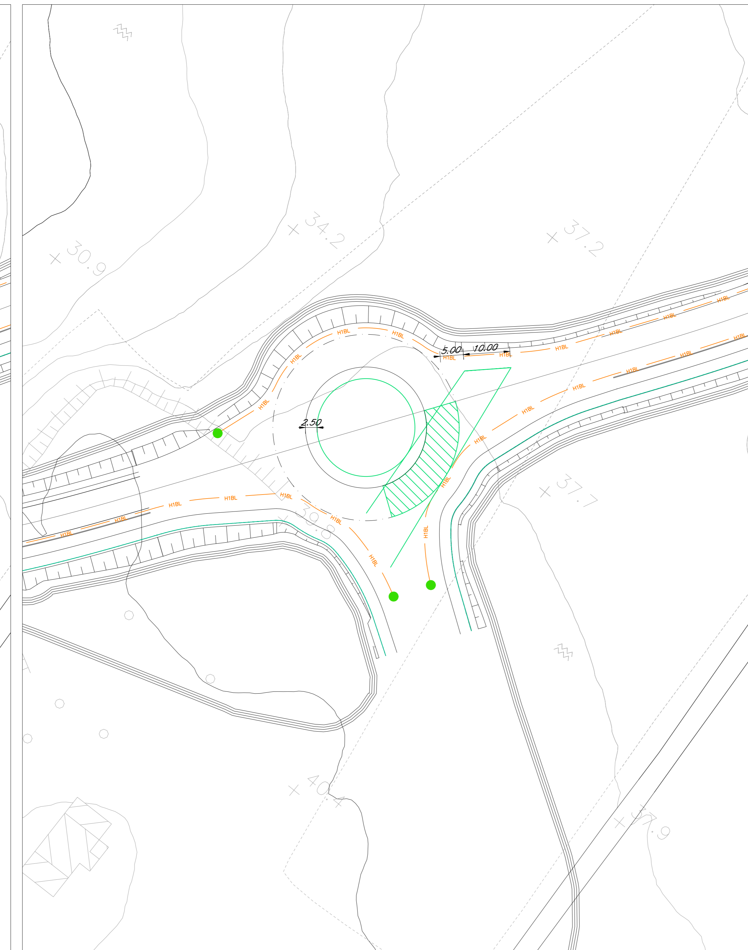
Ramo 1 - Campo di visibilità (NV04A-Tratto 2) Scale 1:500 Ramo 2 - Campo di visibilità (NV04A-Tratto 1) Scale 1:500 Ramo 3 - Campo di visibilità (Viabilità di collegamento alla fermata Campomarino) Scale 1:500
