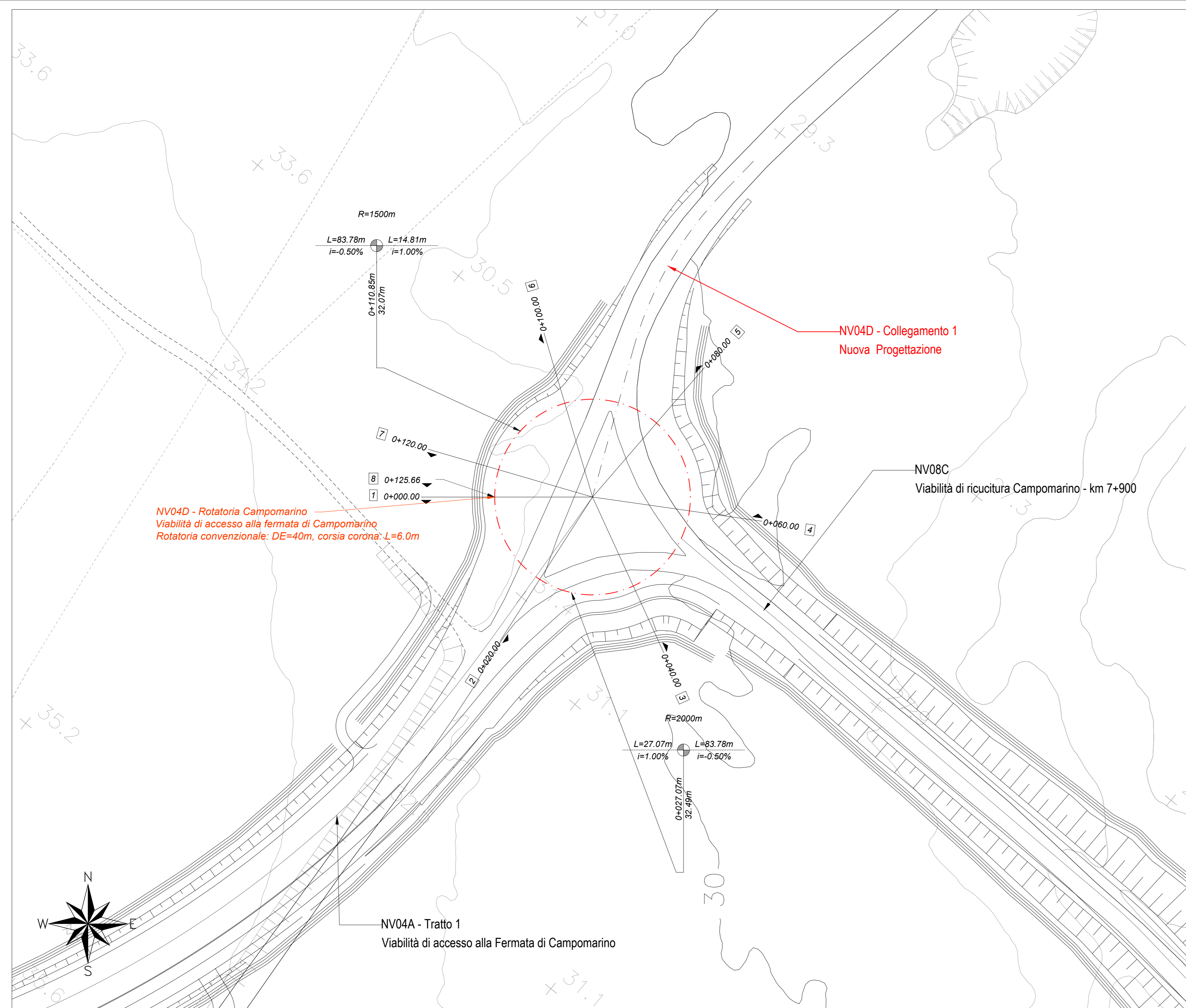
NV04D - Rotatoria Est - Planimetria di tracciamento Scale 1:500
