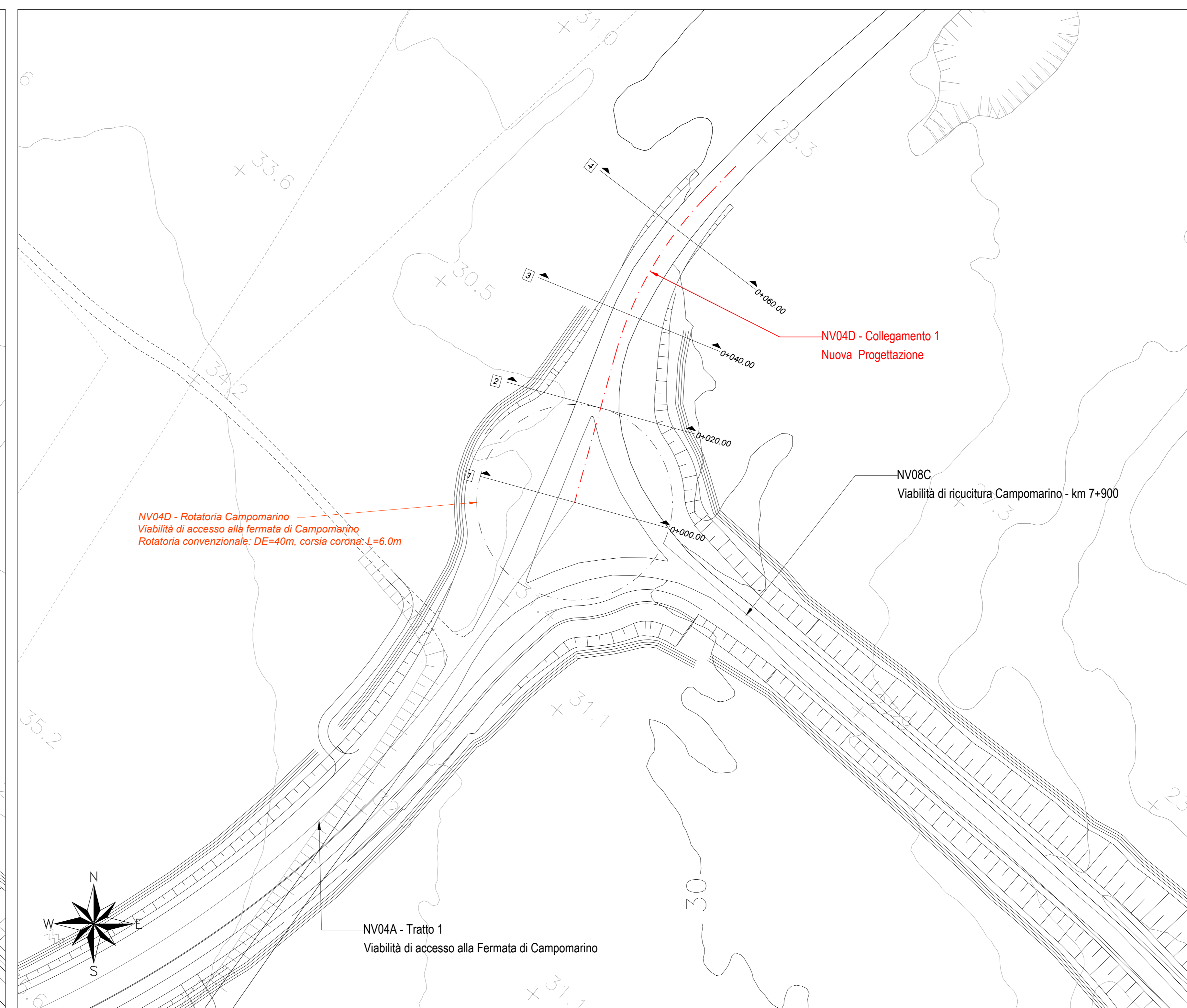
NV04D - Collegamento 1 - Planimetria di tracciamento Scale 1:500
