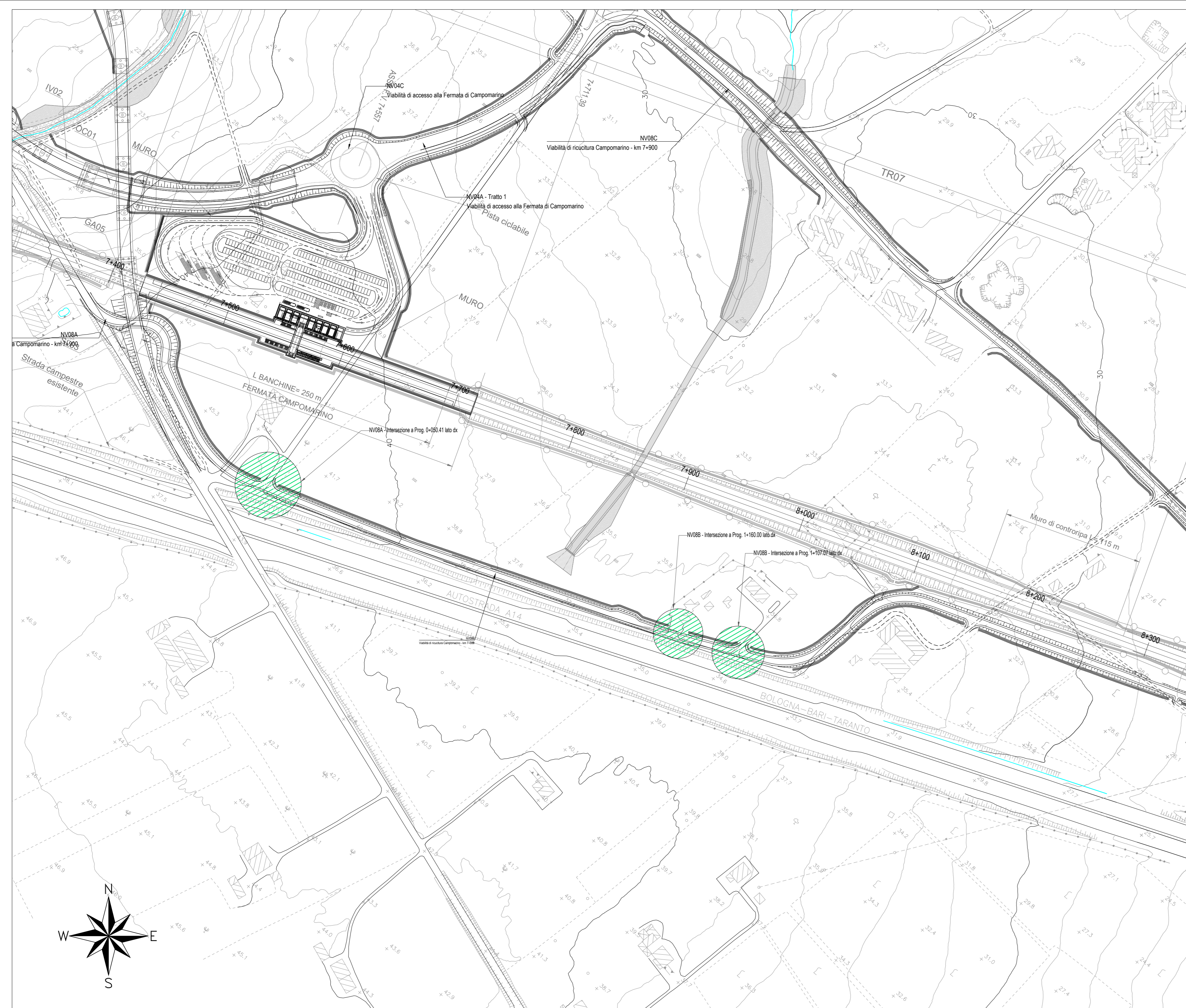
Planimetrica con localizzazione intersezioni Scale 1:2000
