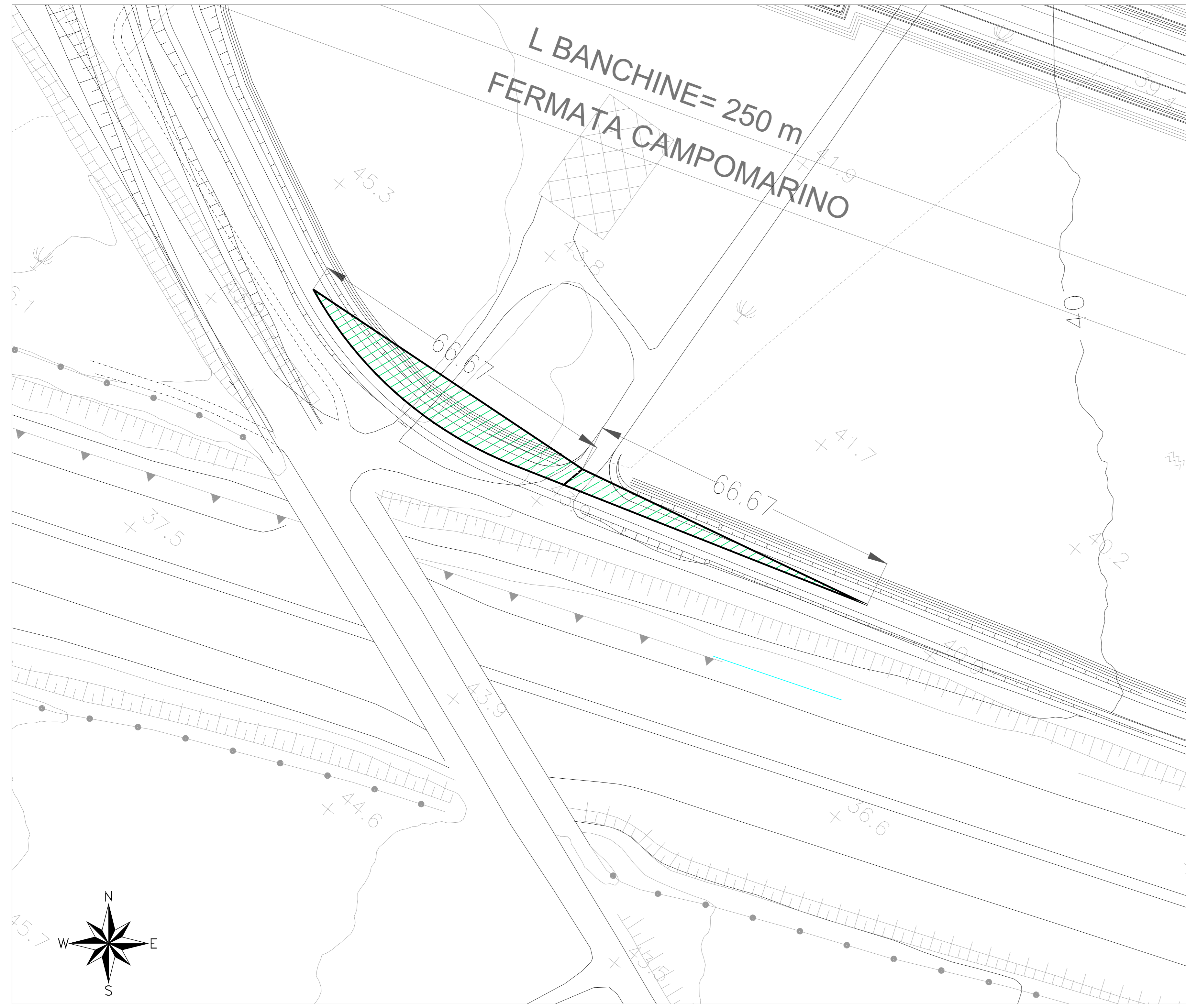
NV08A - Intersezione a Prog. 0+050.41 lato dx - Triangoli di visibilità Scale 1:500
