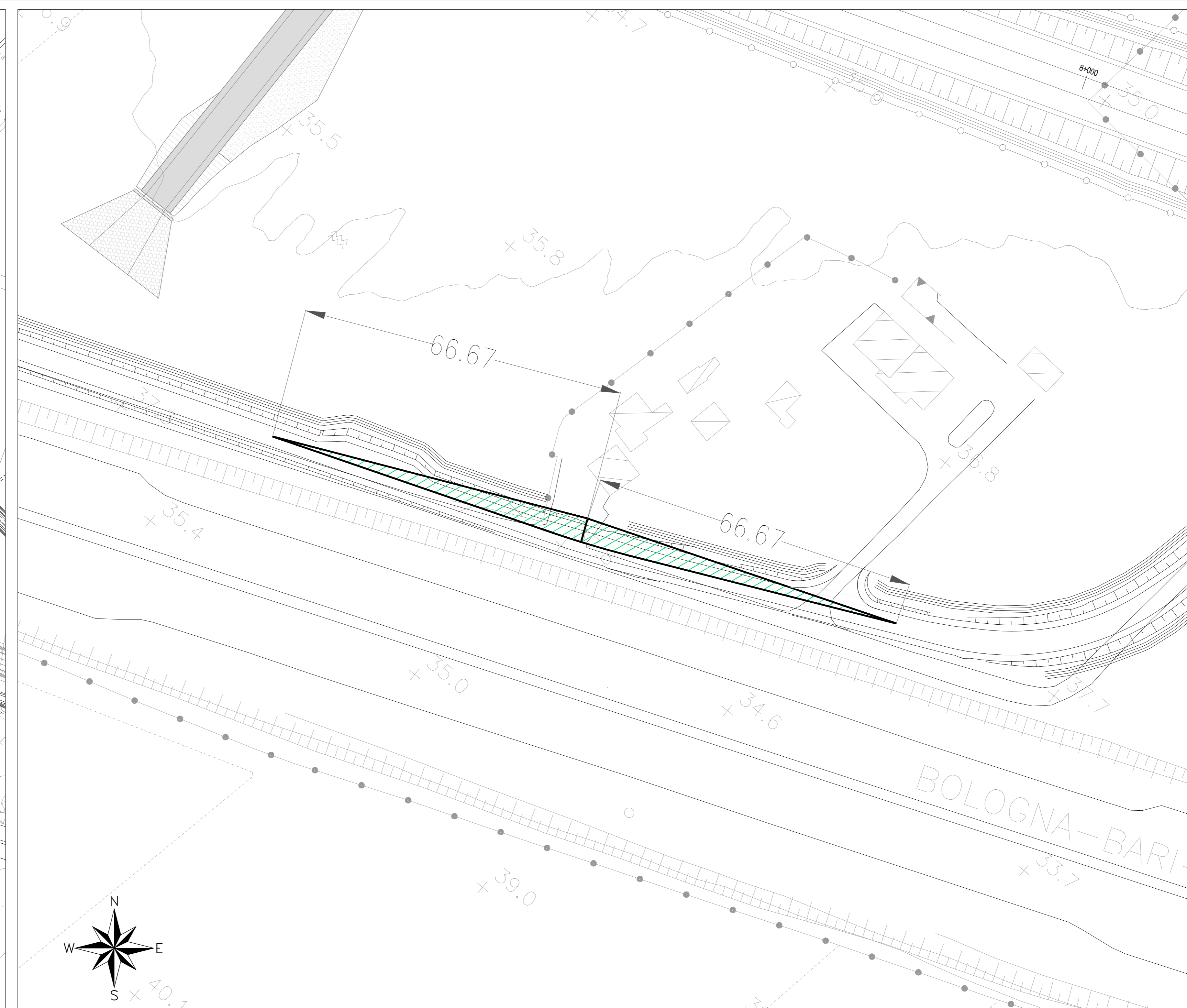
NV08B - Intersezione a Prog. 1+160.00 lato dx - Triangoli di visibilità Scale 1:500
