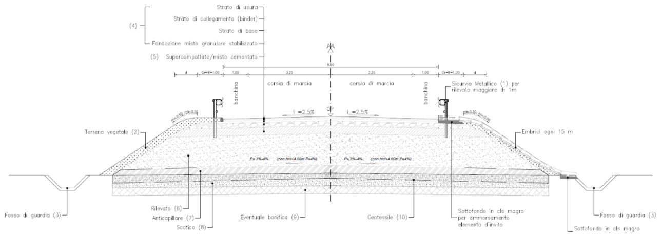
Figura 9 - Sezione tipo in rilevato
