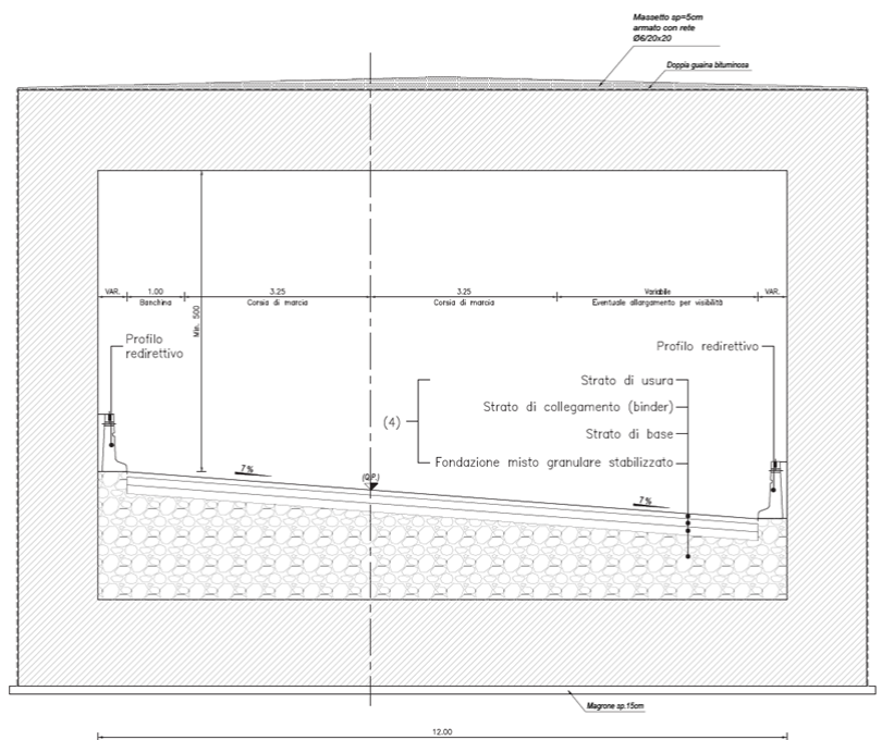
Figura 11 - Sezione tipo in sottovia
