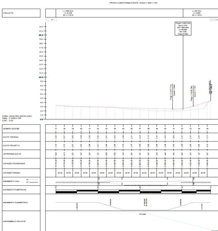
Figura 7: Profilo di progetto (Tav.2/2)
