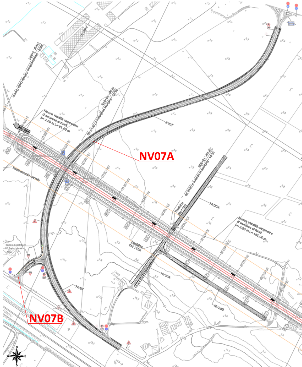
Figura 5: Planimetria di progetto
