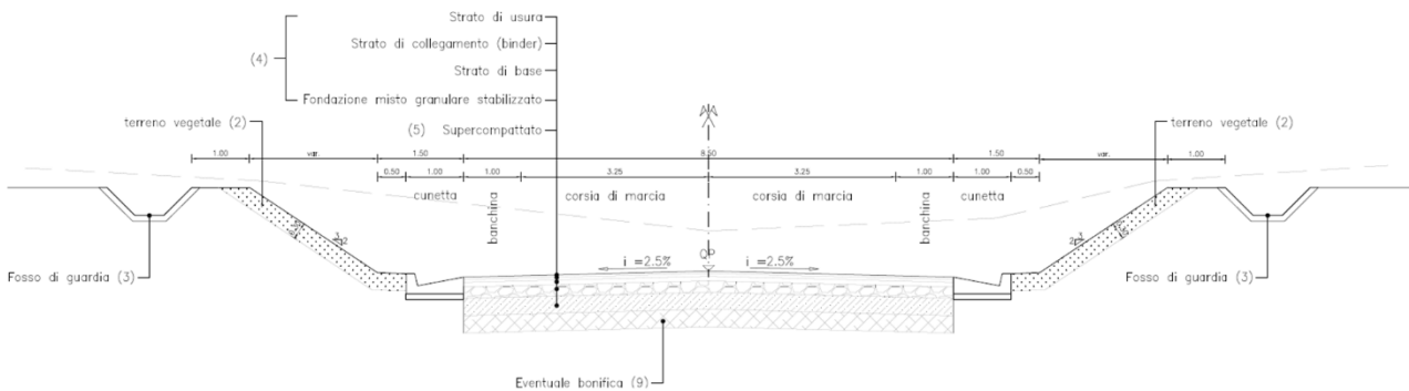
Figura 10 - Sezione tipo in trincea
