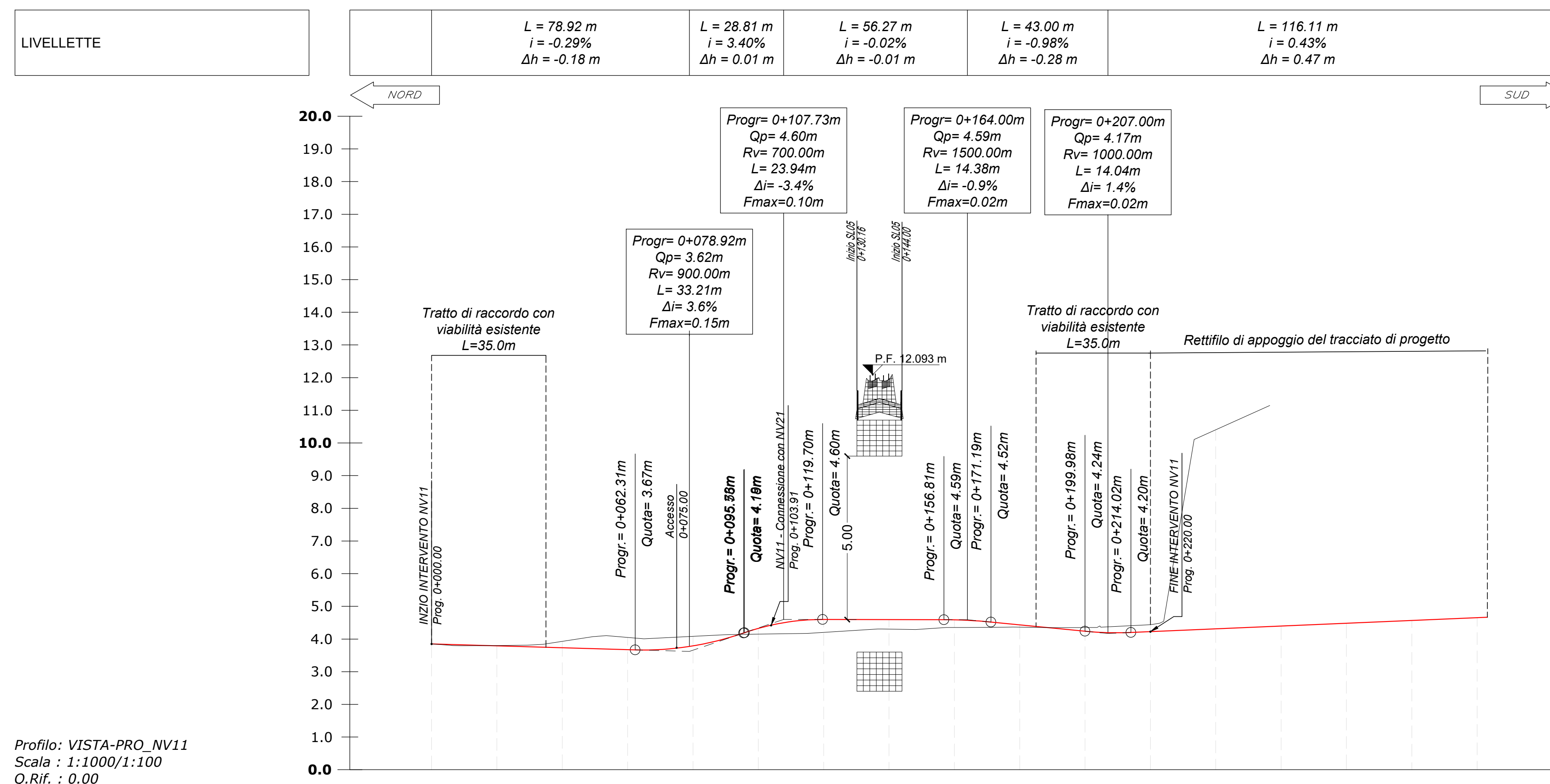
PROFILO LONGITUDINALE NV11 - SCALA 1:1000 / 1:100
