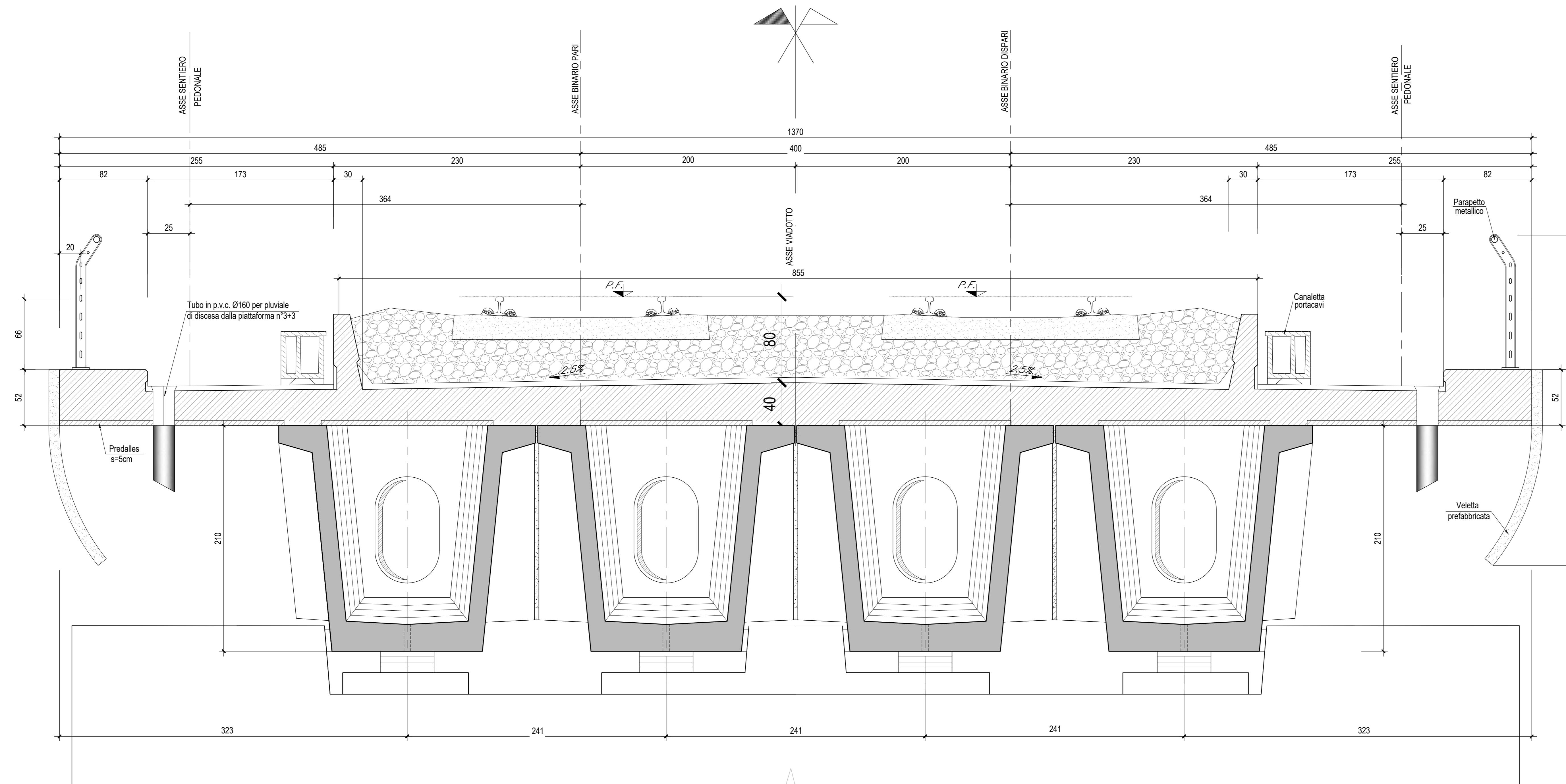
SEZIONE TRASVERSALE A-A-Scala 1:20
