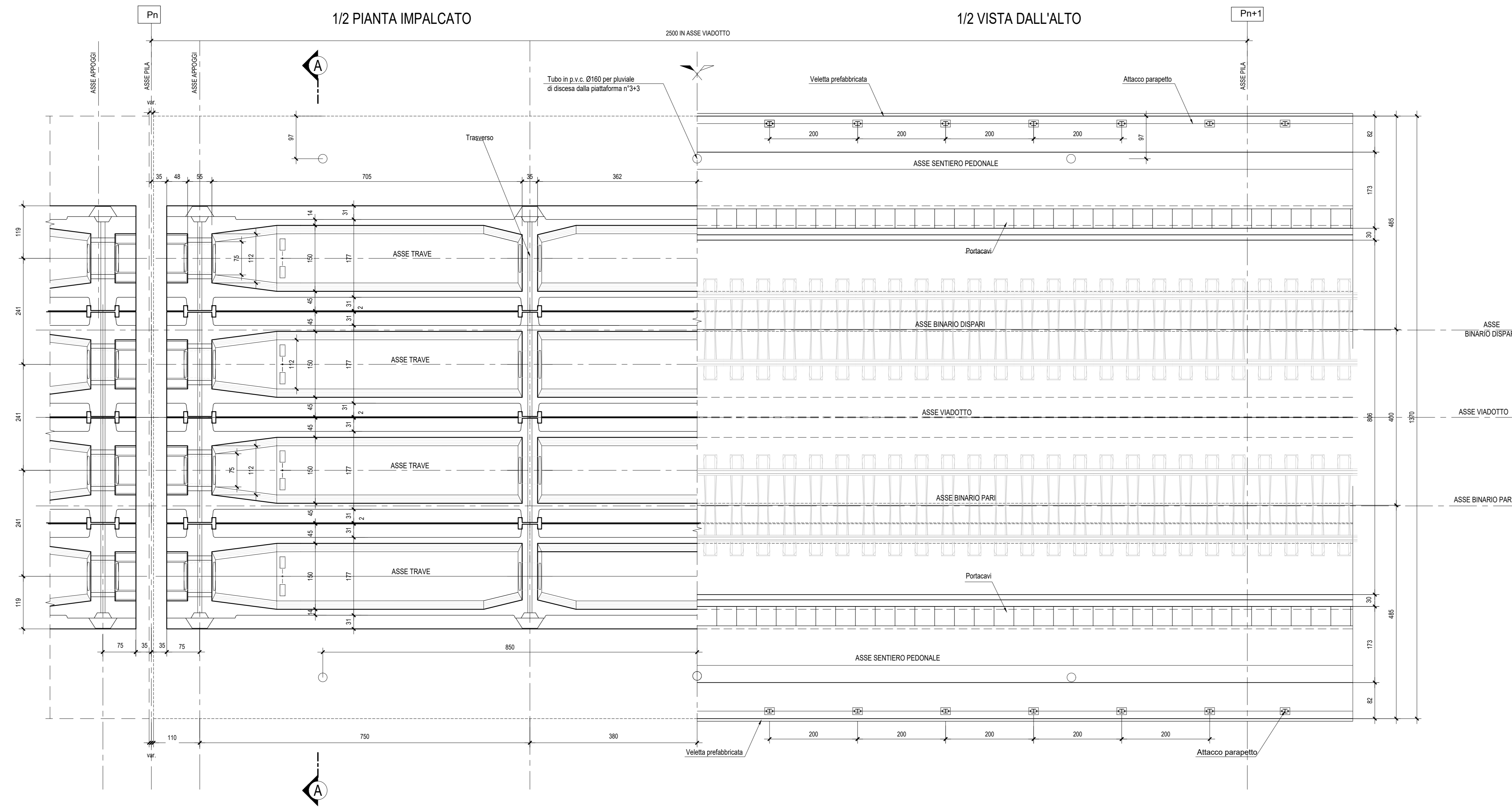
PIANTA IMPALCATO-Scala 1:50
