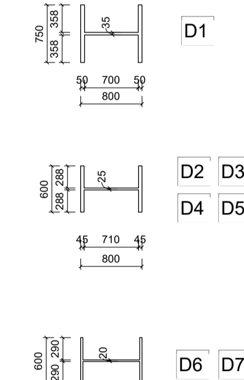
ELEMENTI DIAGONALI TIPICI - SEZIONI TRASVERSALI Scala 1:50
