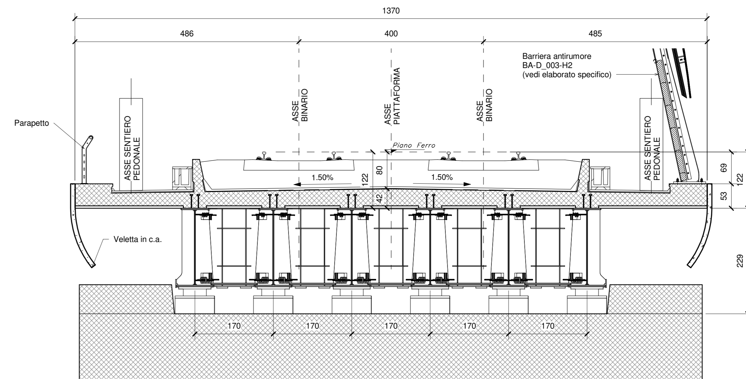
SEZIONE TIPO IN ASSE APPOGGIO SPALLA SP01 Scala 1:50 (Campata L=32.00m)
