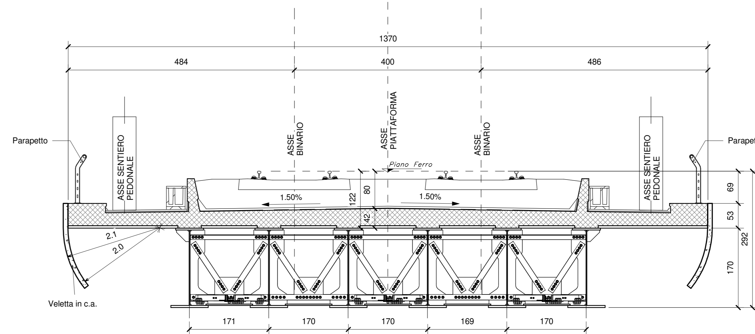
SEZIONE TIPO IN CAMPATA - Scala 1:50 (Campata L=32.00m)
