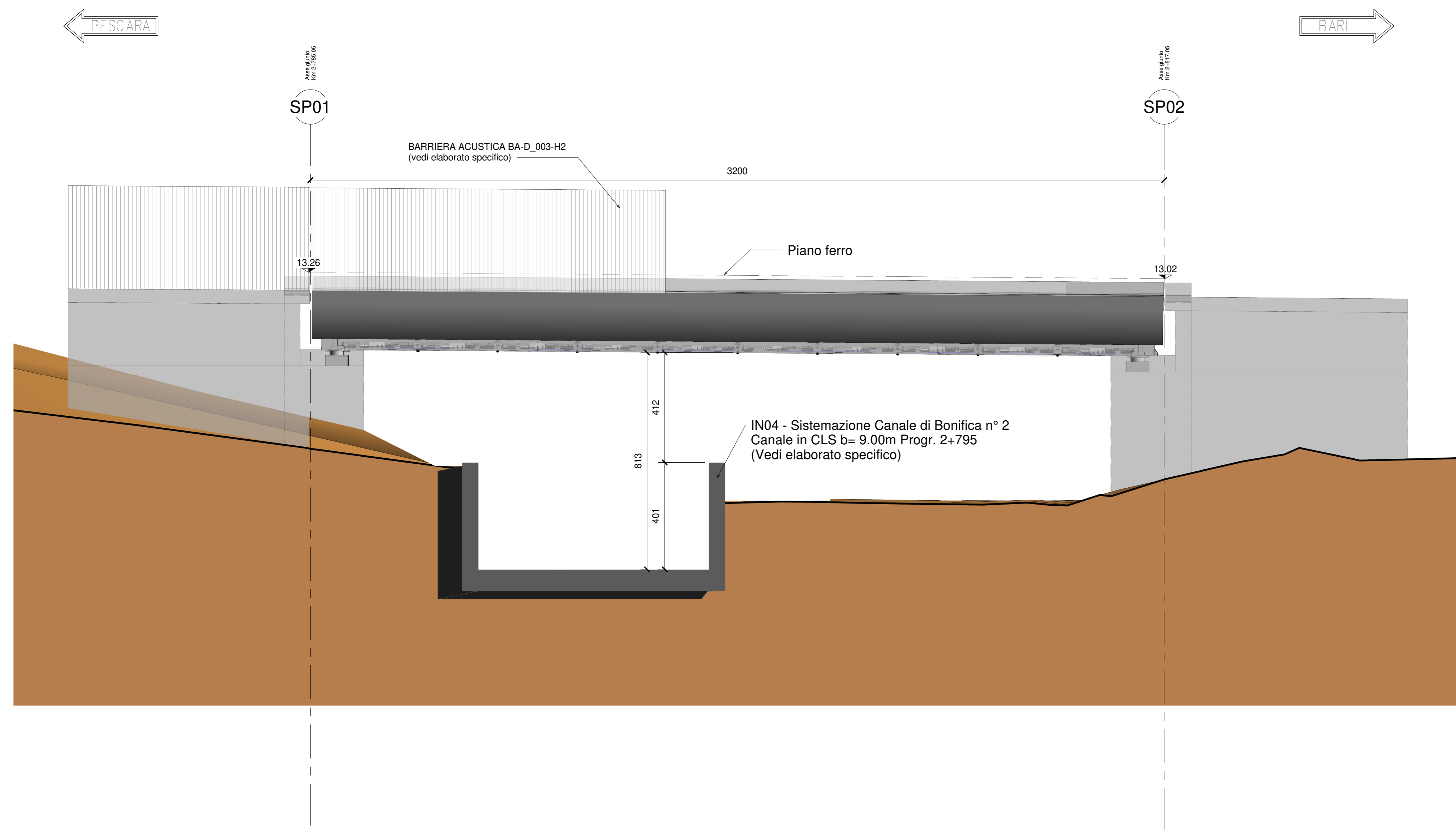
PROSPETTO LONGITUDINALE - Scala 1:100
