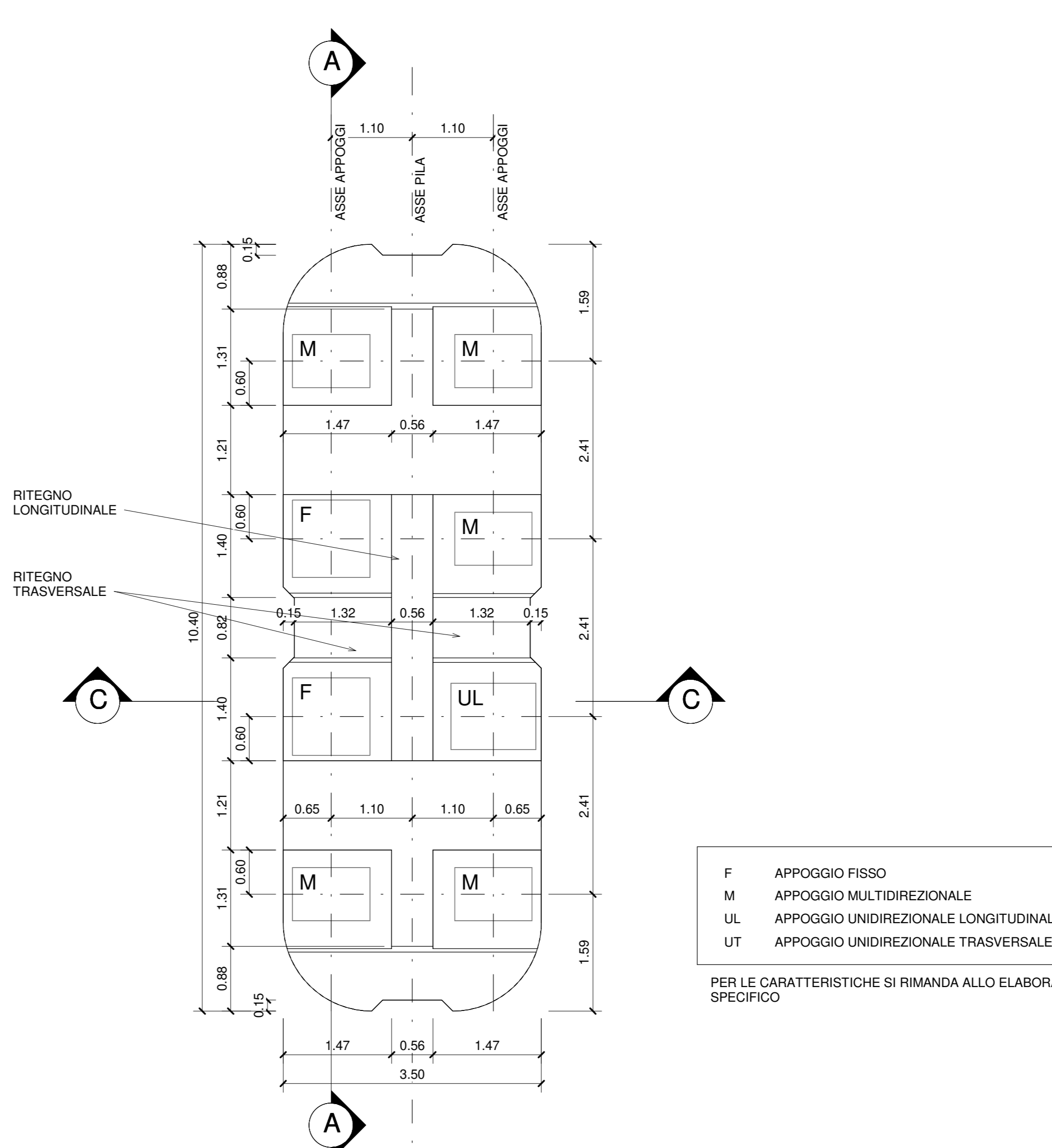
PIANTA PULVINO Scala 1:50
