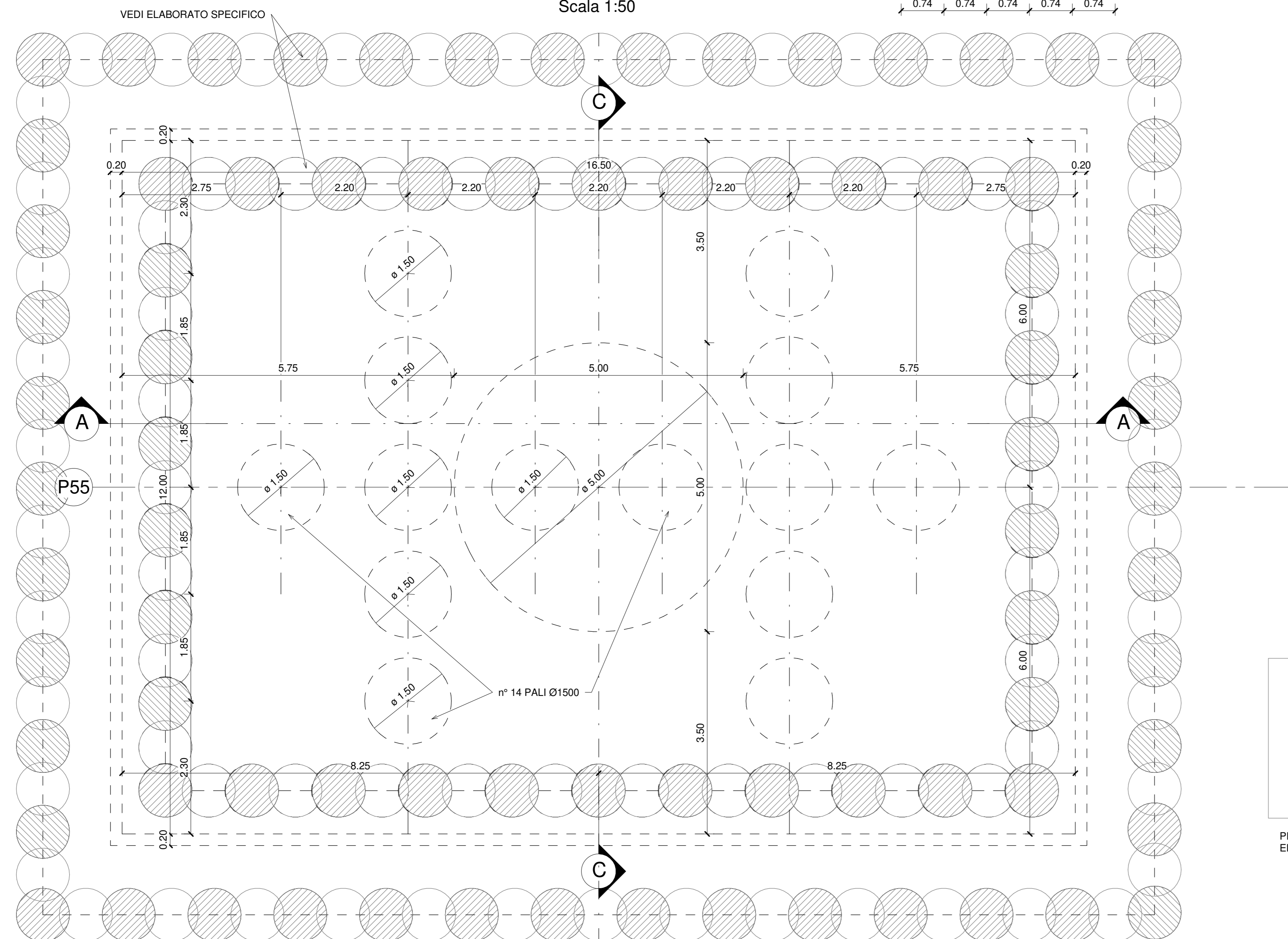
PIANTA FONDAZIONE Scala 1:50
