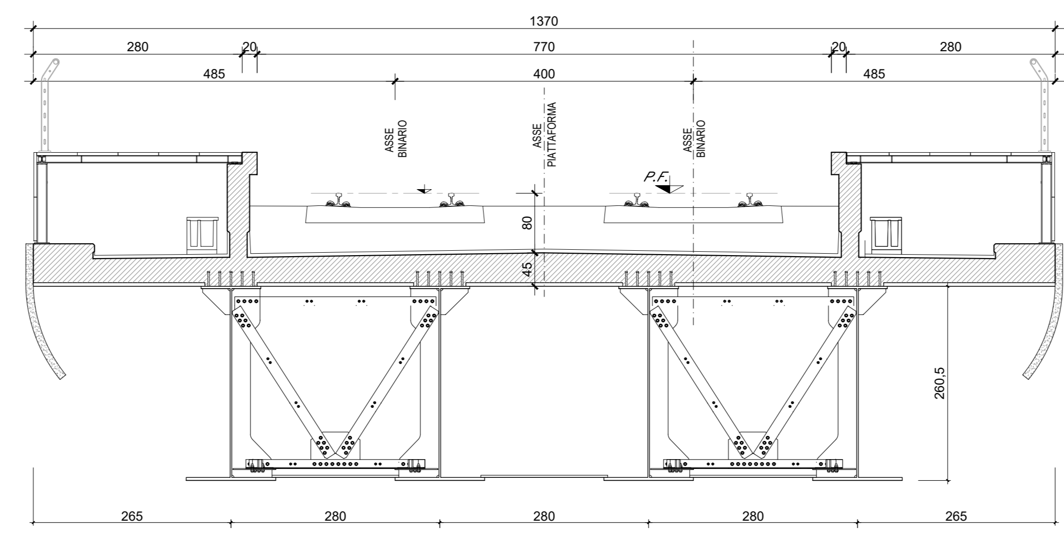
IMPALCATO IN ACCIAIO - Scala 1:50 SEZIONE TRASVERSALE TIPO IN CAMPATA
