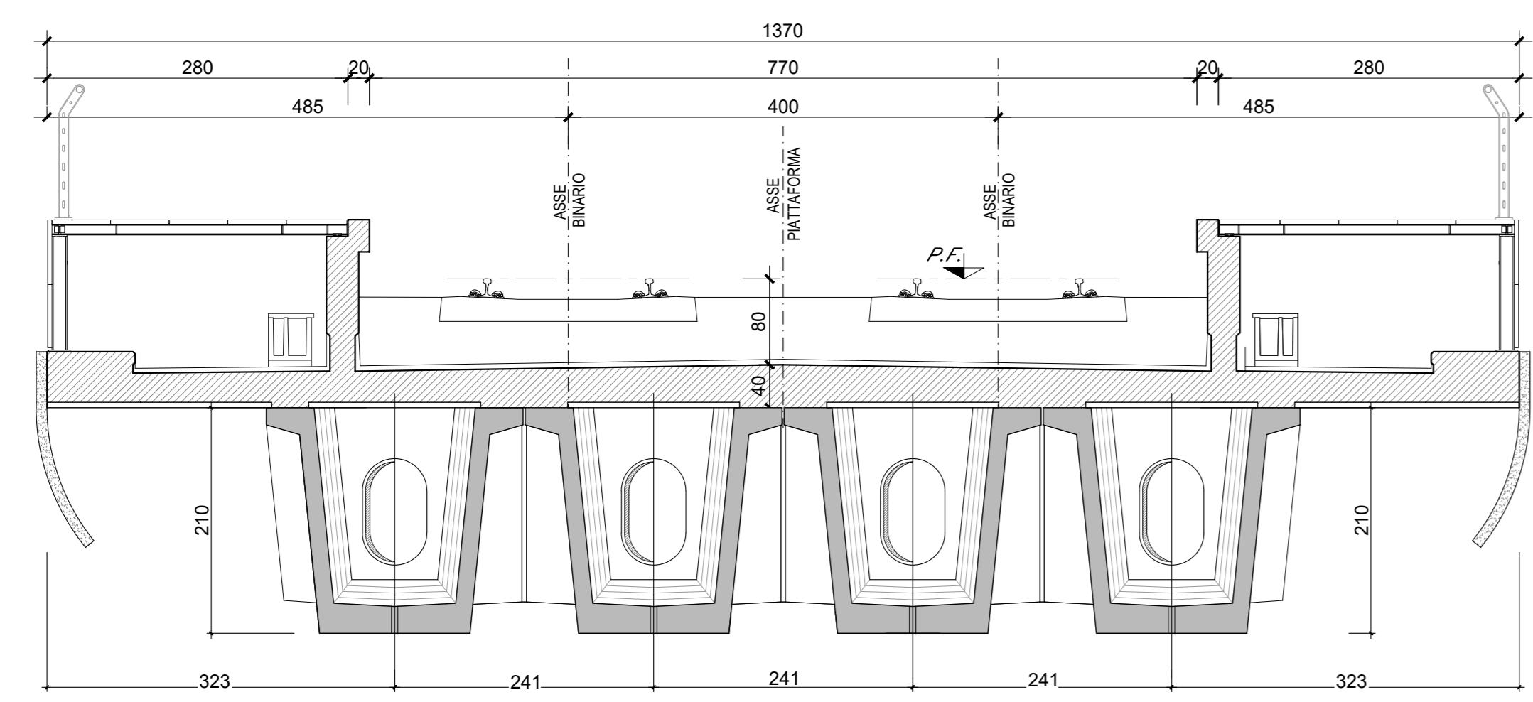
IMPALCATO IN C.A.P. - Scala 1:50 SEZIONE TRASVERSALE TIPO IN CAMPATA
