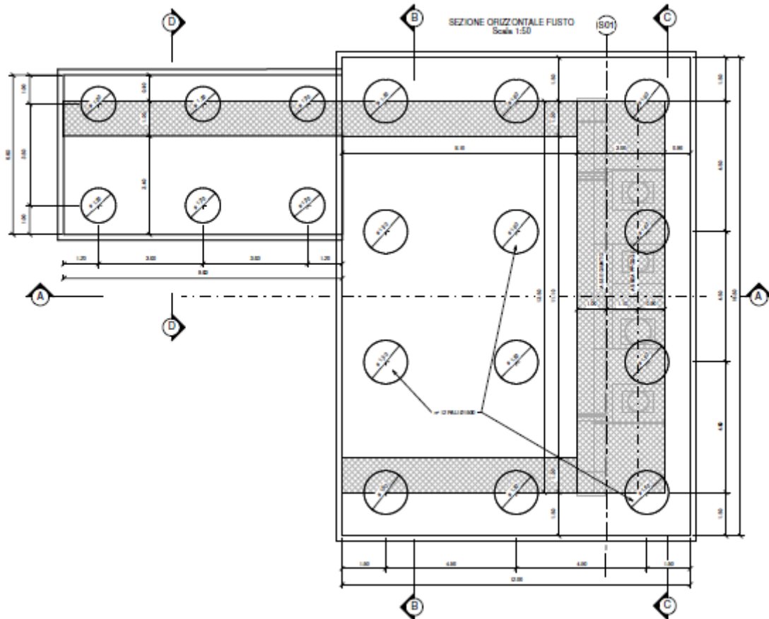
Figura 4 – Vista in pianta
