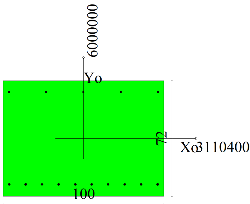
Figura 43 – Sezione trasversale muro di sostegno e relativa armatura
