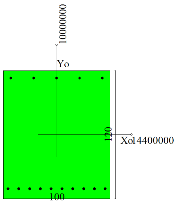
Figura 44 – Sezione trasversale muro d'ala e relativa armatura
