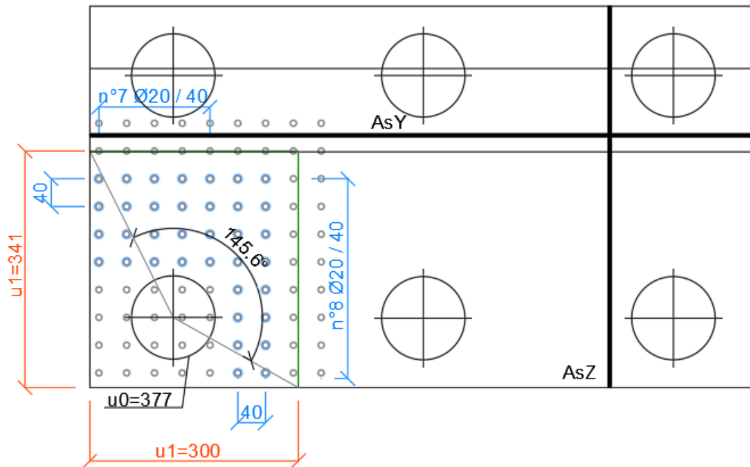
Figura 46 – Schema delle verifiche a taglio-punzonamento per il palo più caricato
