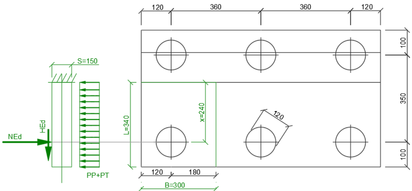
Figura 45 – Schema delle verifiche a flessione del plinto per il palo più caricato
