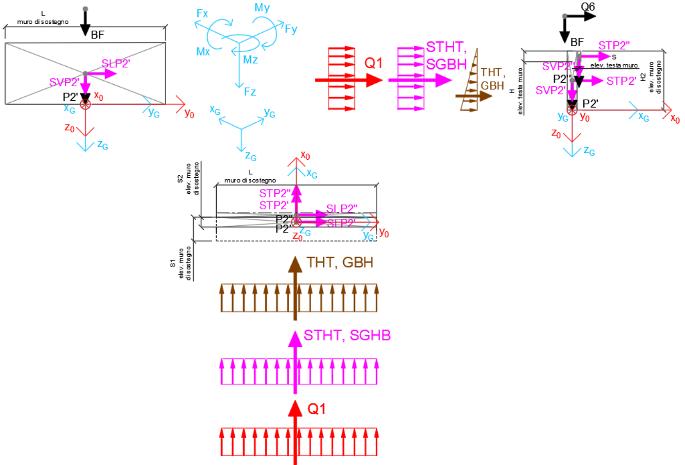
Figura 41 – Schema e sistema di riferimento utilizzato per il calcolo delle azioni applicate
