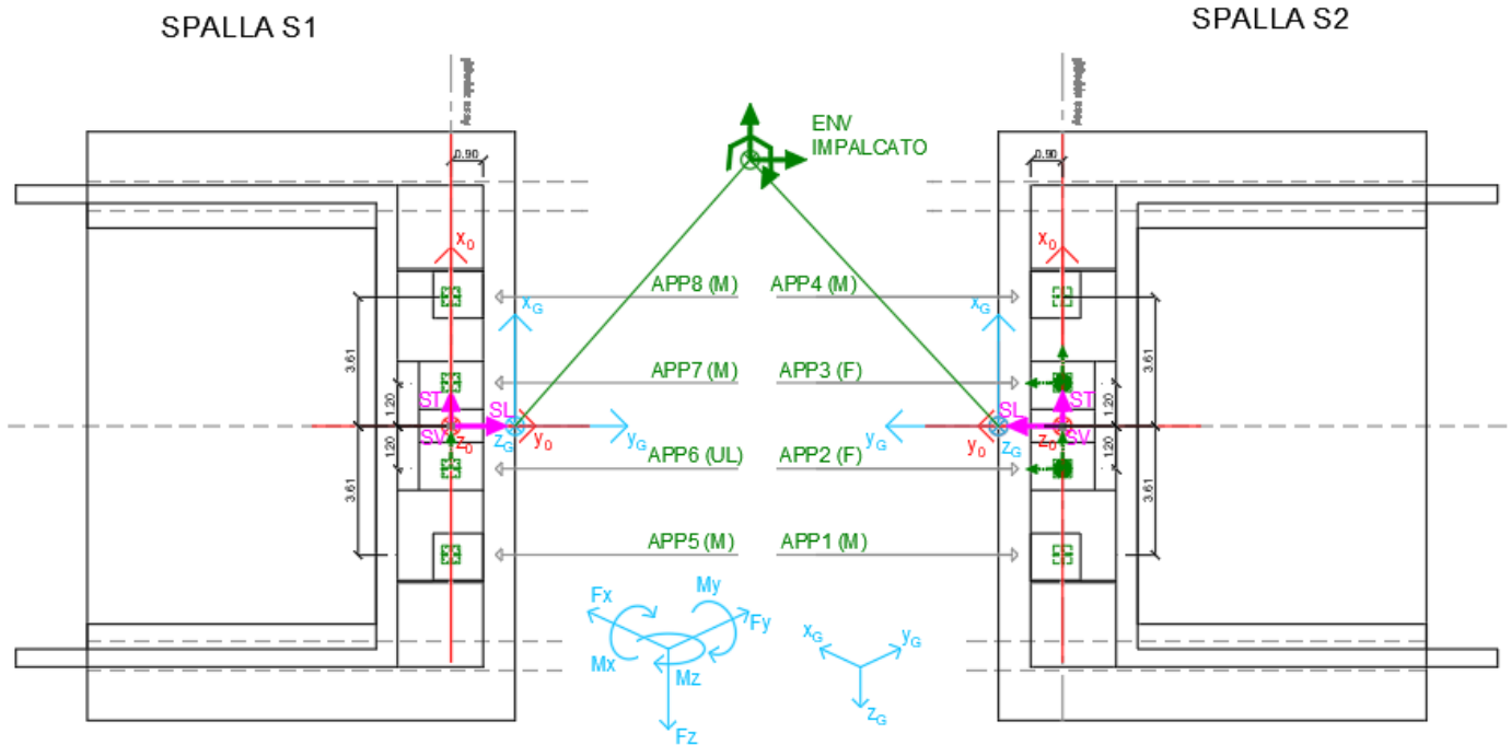
Figura 27- - Schema dei vincoli a terra impalcato
