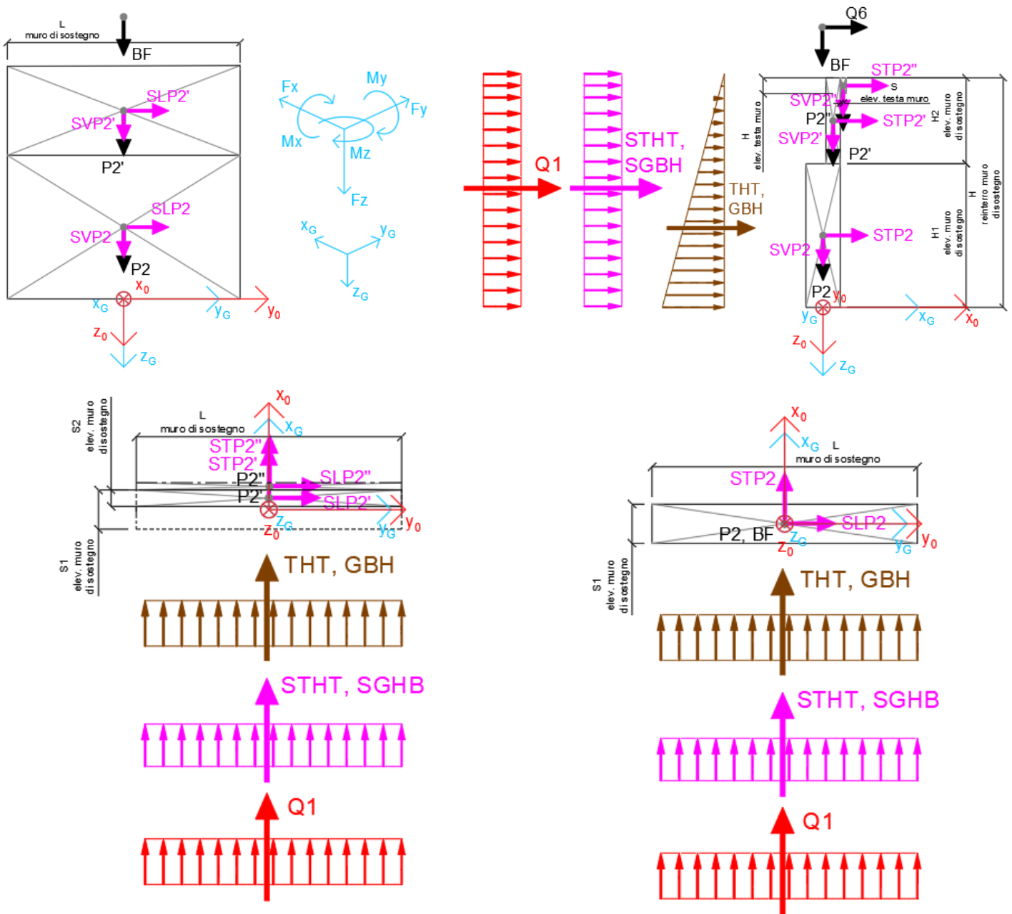
Figura 42 – Schema e sistema di riferimento utilizzato per il calcolo delle azioni applicate
