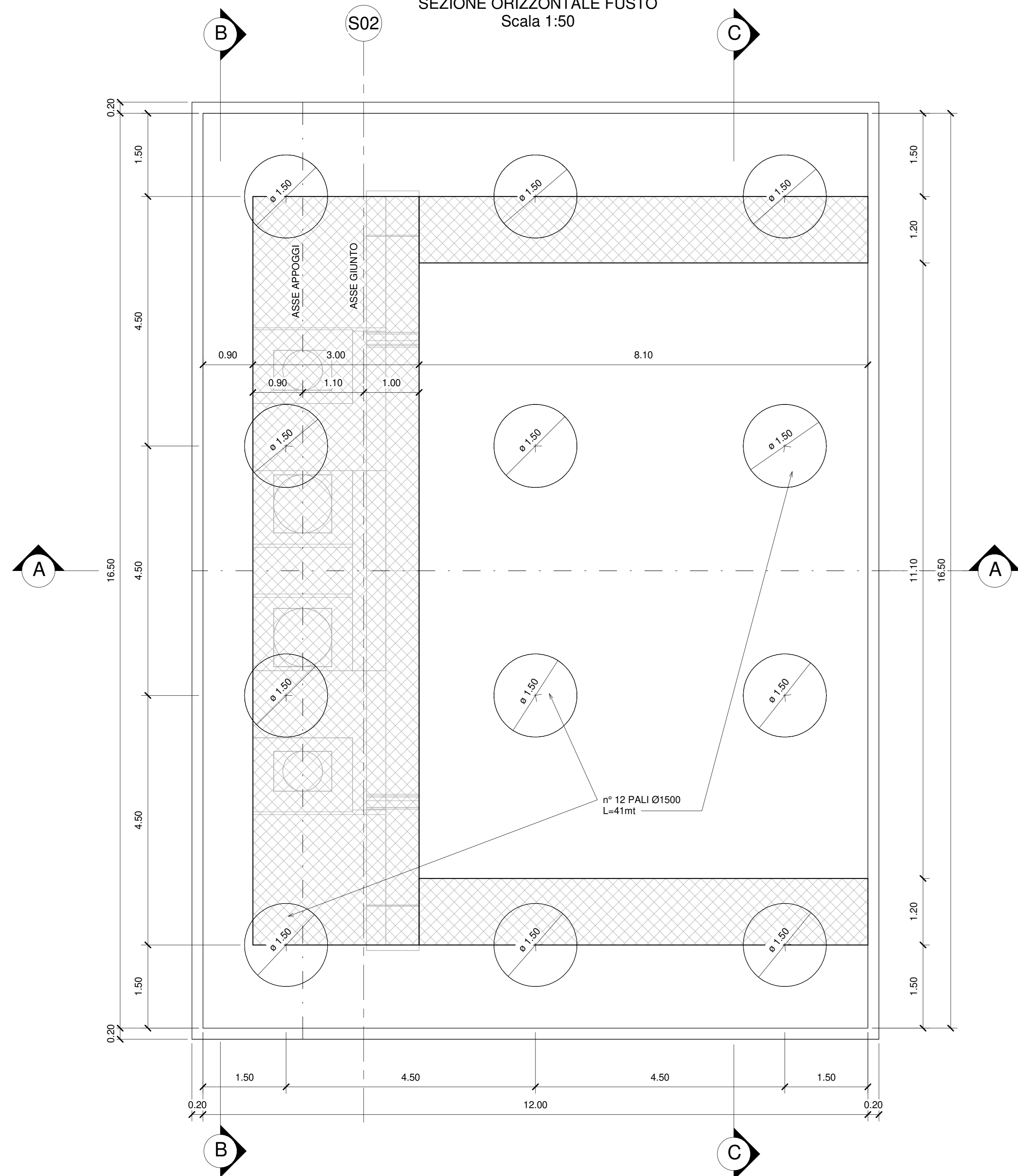
SEZIONE ORIZZONTALE FUSTO Scala 1:50
