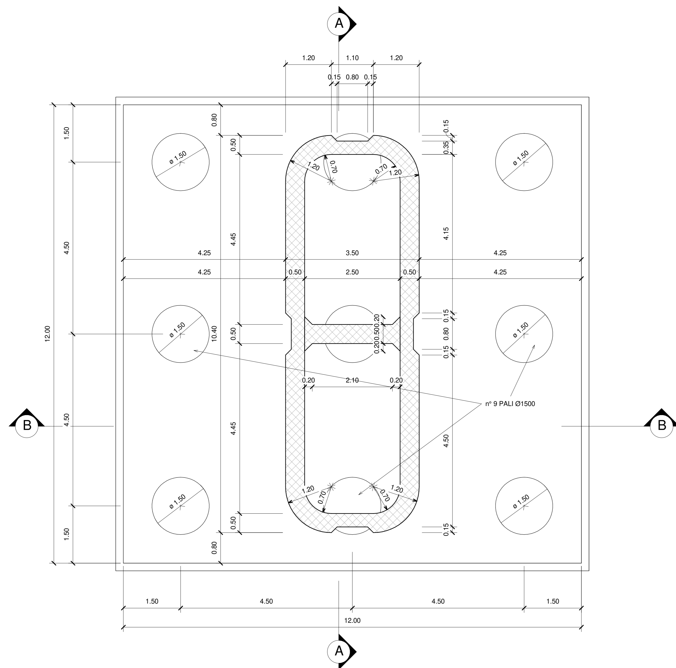
SEZIONE ORIZZONTALE FUSTO Scala 1:50
