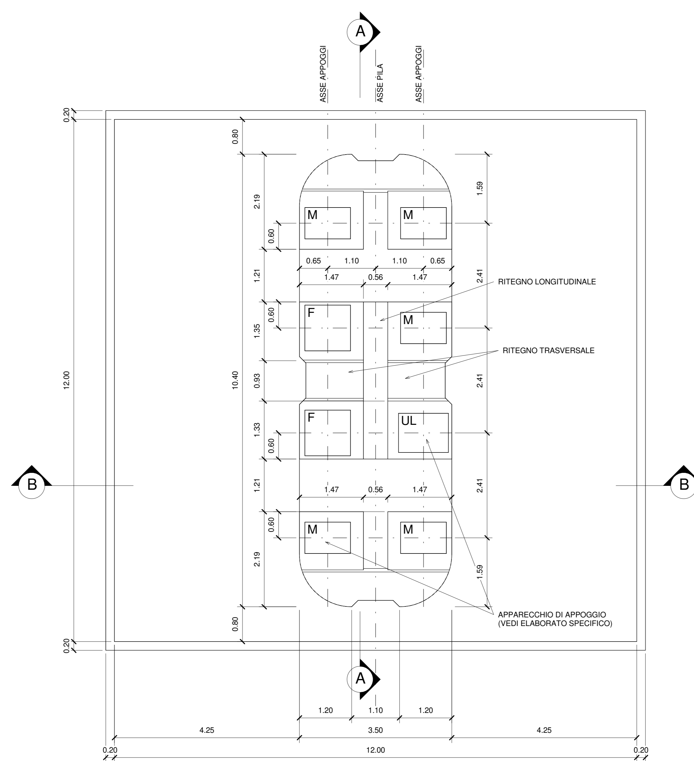
PIANTA PULVINO Scala 1:50
