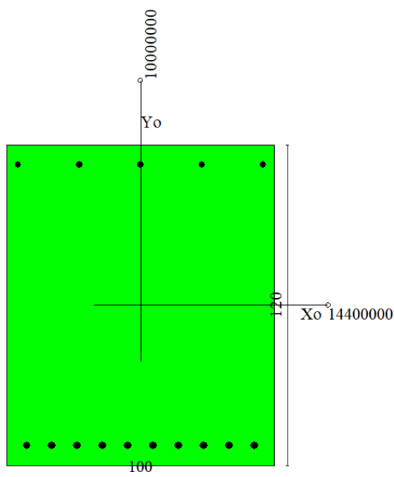
Figura 39 – Sezione trasversale muro d'ala e relativa armatura
