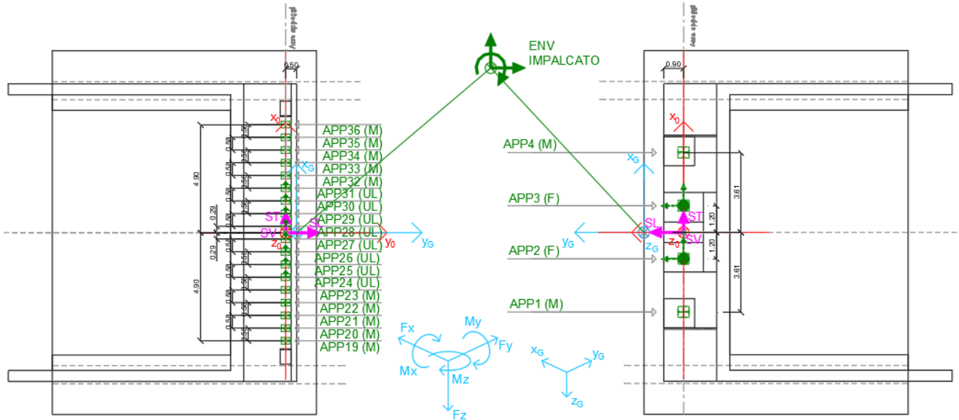
Figura 27- - Schema dei vincoli a terra impalcato
