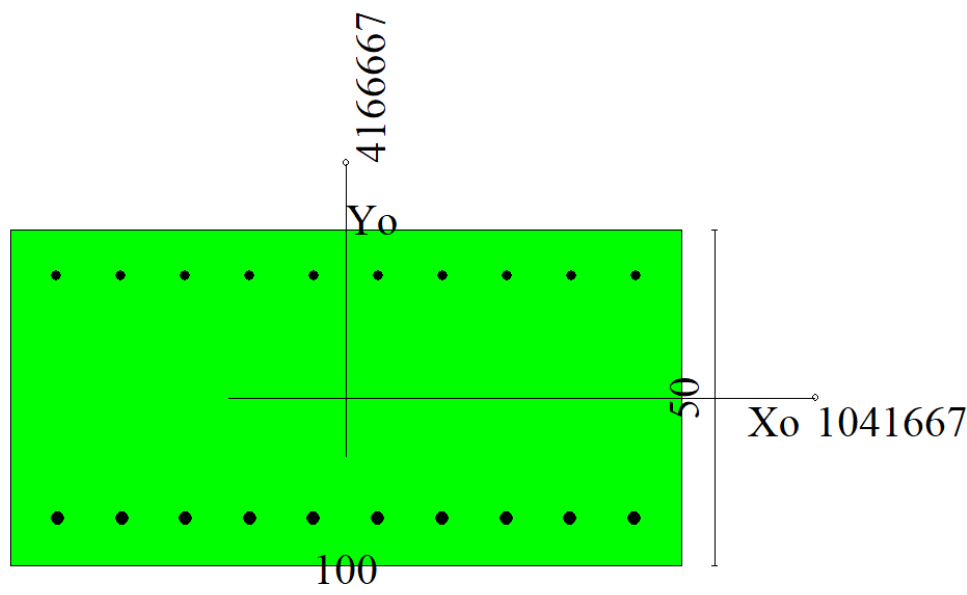
Figura 38 – Sezione trasversale muro d'ala e relativa armatura
