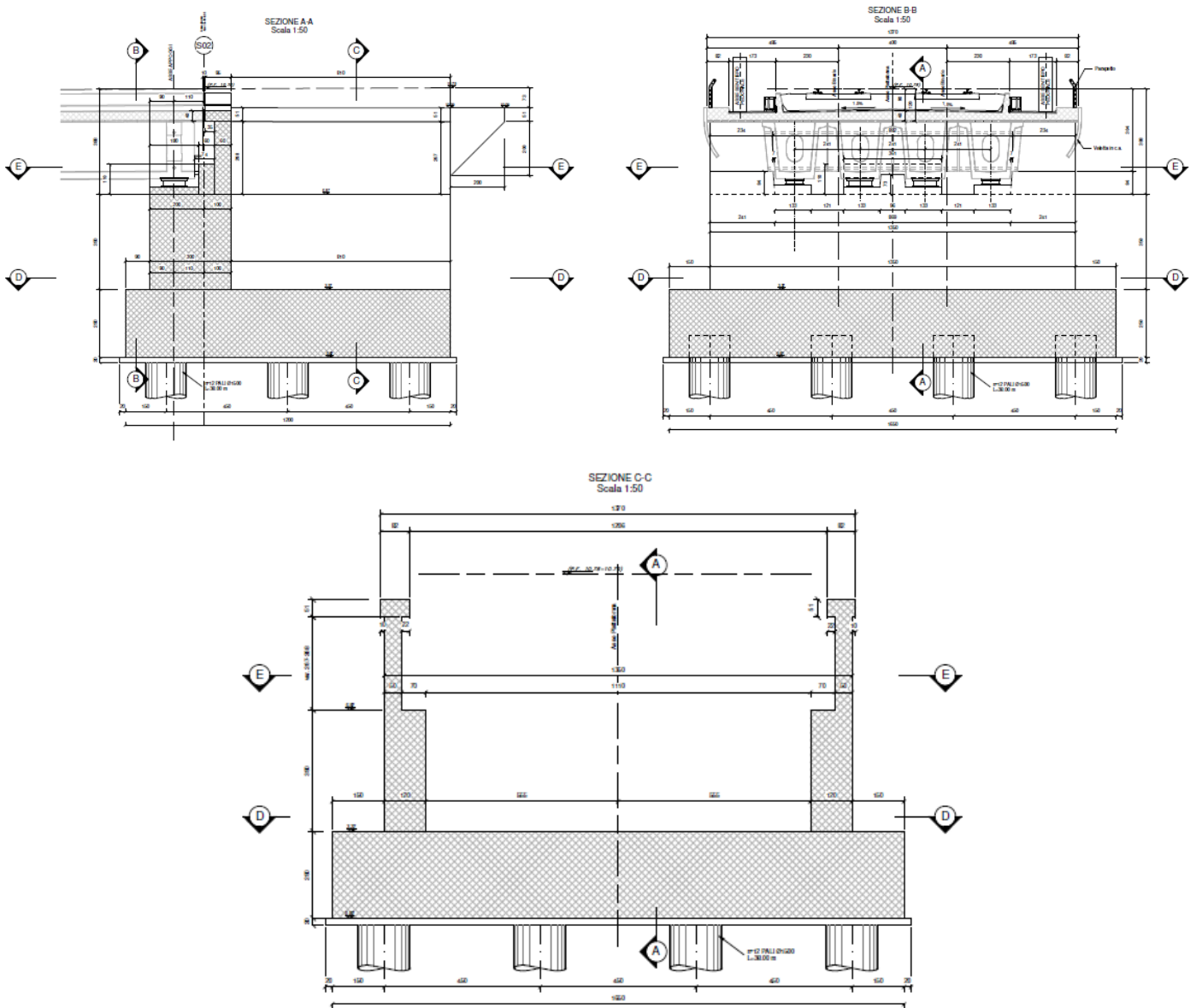
Figura 3 – Sezioni in direzione longitudinale e trasversale
