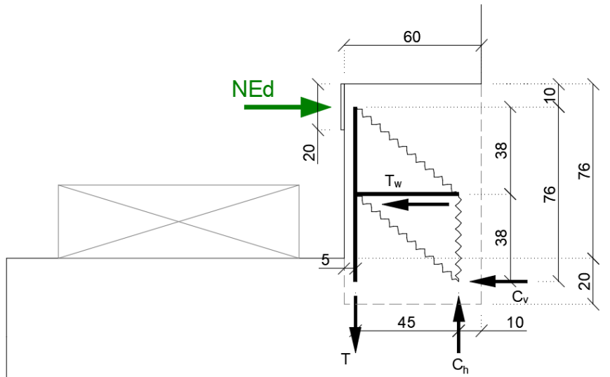
Figura 45 – Schema delle verifiche locali del ritegno longitudinale
