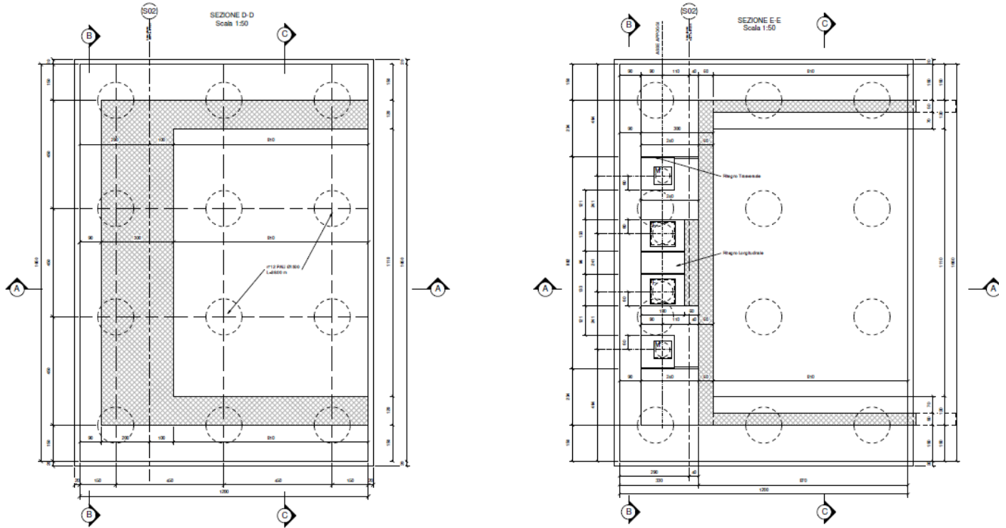
Figura 4 – Vista in pianta
