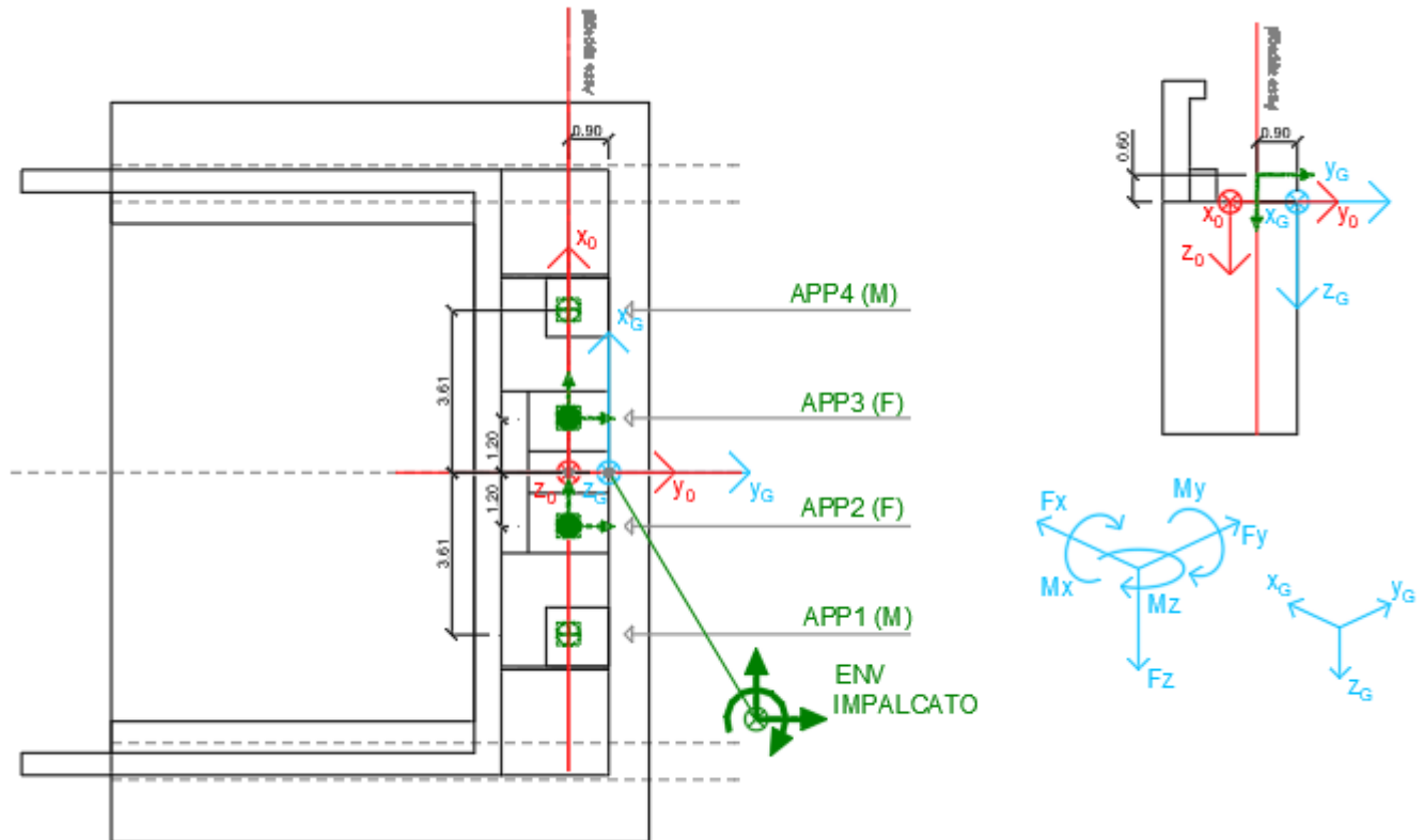
Figura 32 – Schema e sistema di riferimento utilizzato per il calcolo delle azioni applicate
