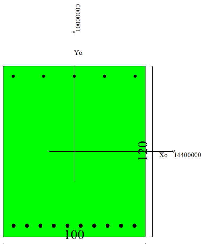
Figura 40 – Sezione trasversale muro d'ala e relativa armatura
