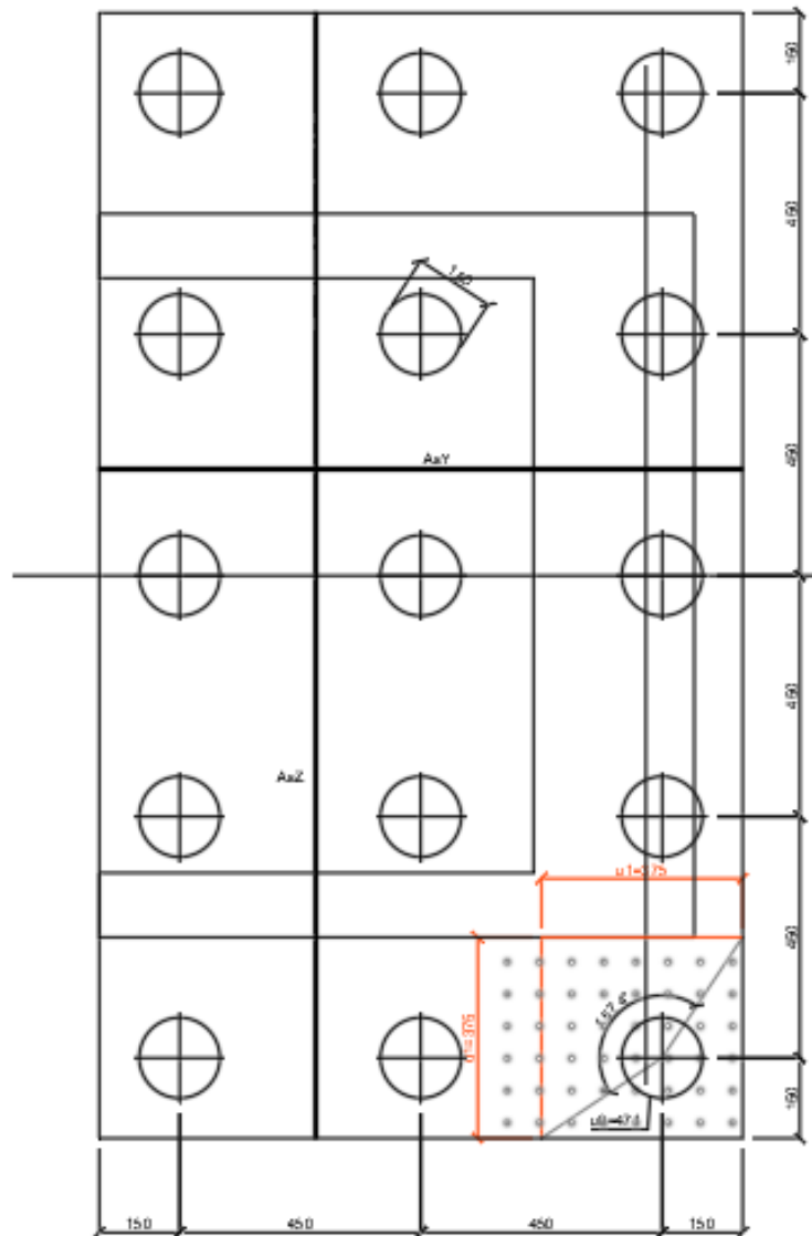
Figura 37 – Schema delle verifiche a taglio-punzonamento per il palo più caricato
