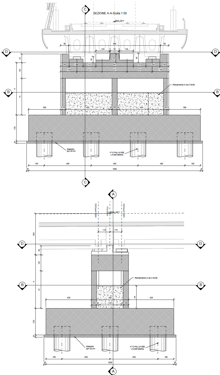
Figura 4 – Sezioni in direzione longitudinale e trasversale
