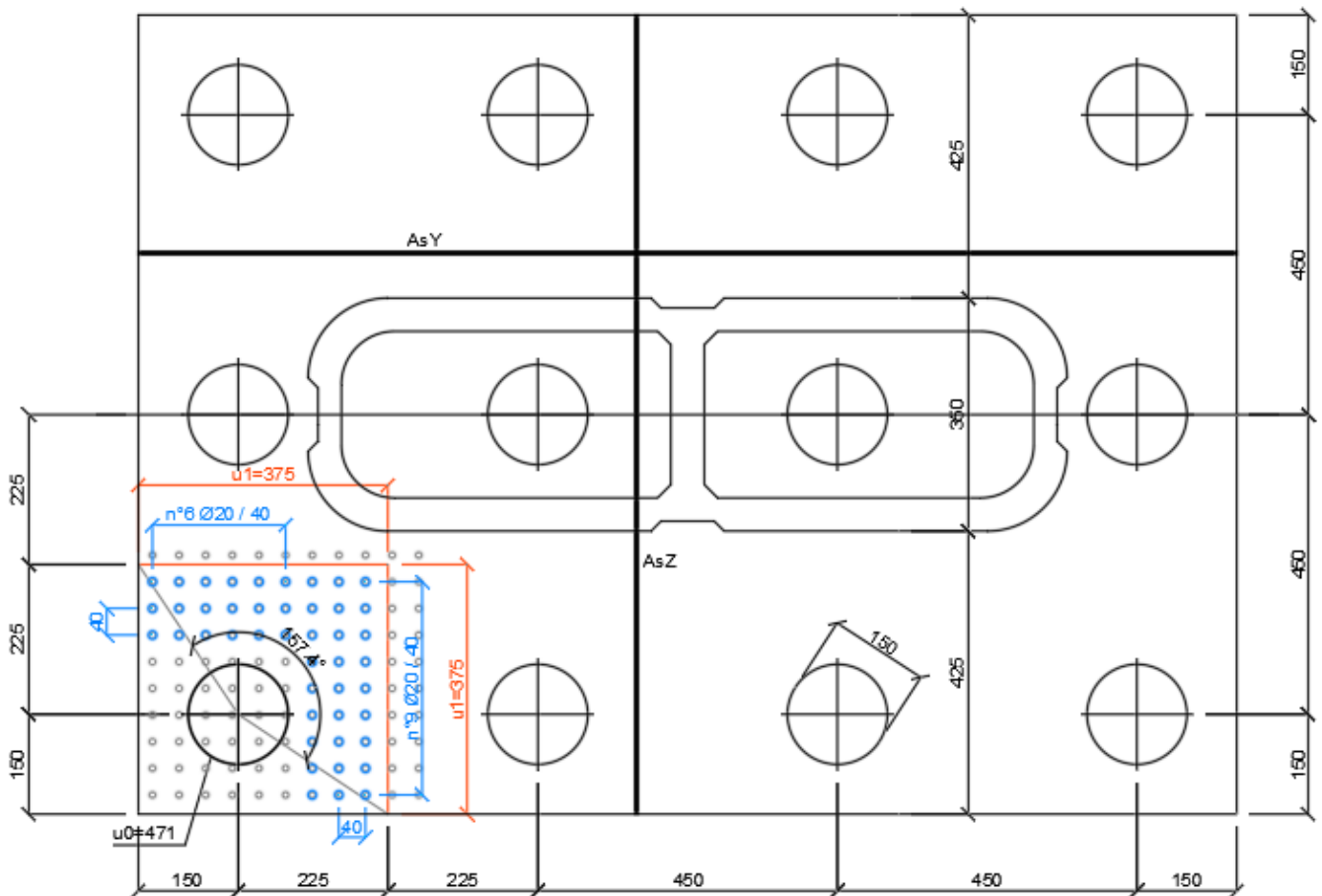
Figura 32 – Schema delle verifiche a taglio-punzonamento per il palo più caricato
