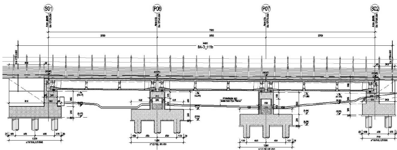
Figura 1 – Profilo longitudinale VI07
