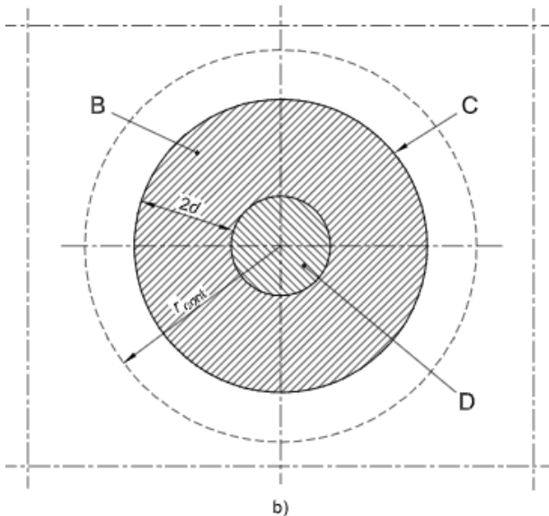
Figura 25 – Modello di verifica a punzonamento SLU
