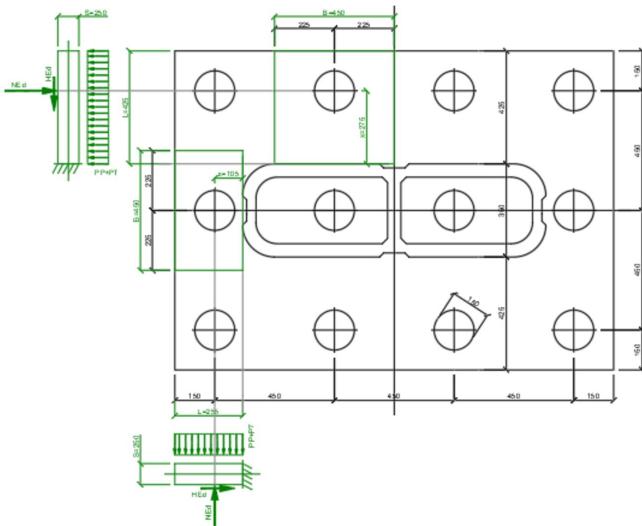
Figura 31 – Schema delle verifiche a flessione del plinto per il palo più caricato
