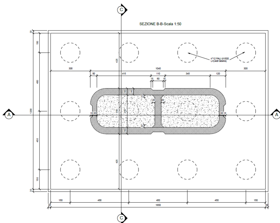
Figura 3 – Vista in pianta
