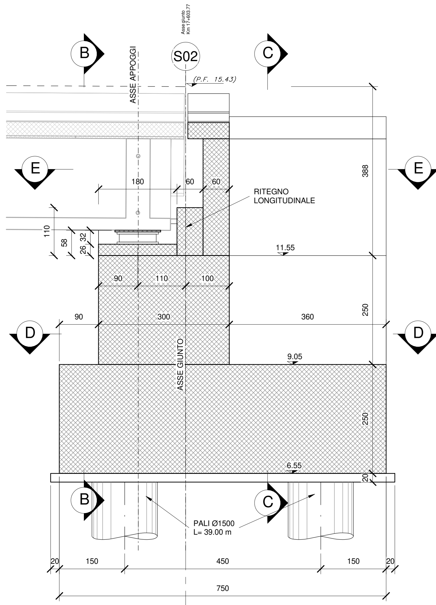
SEZIONE A-A-Scala 1:50
