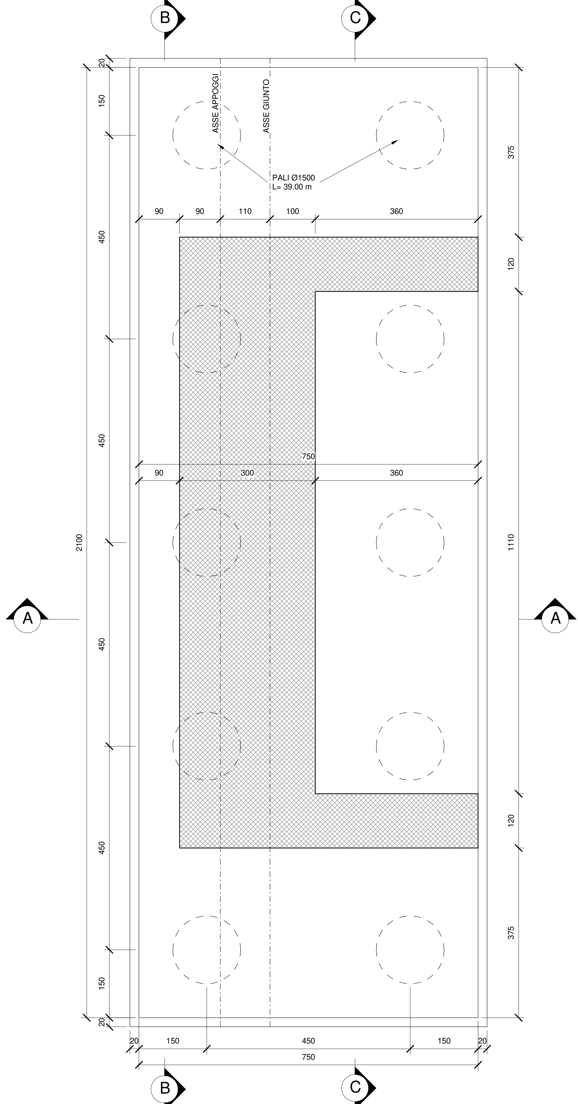
SEZIONE D-D-Scala 1:50
