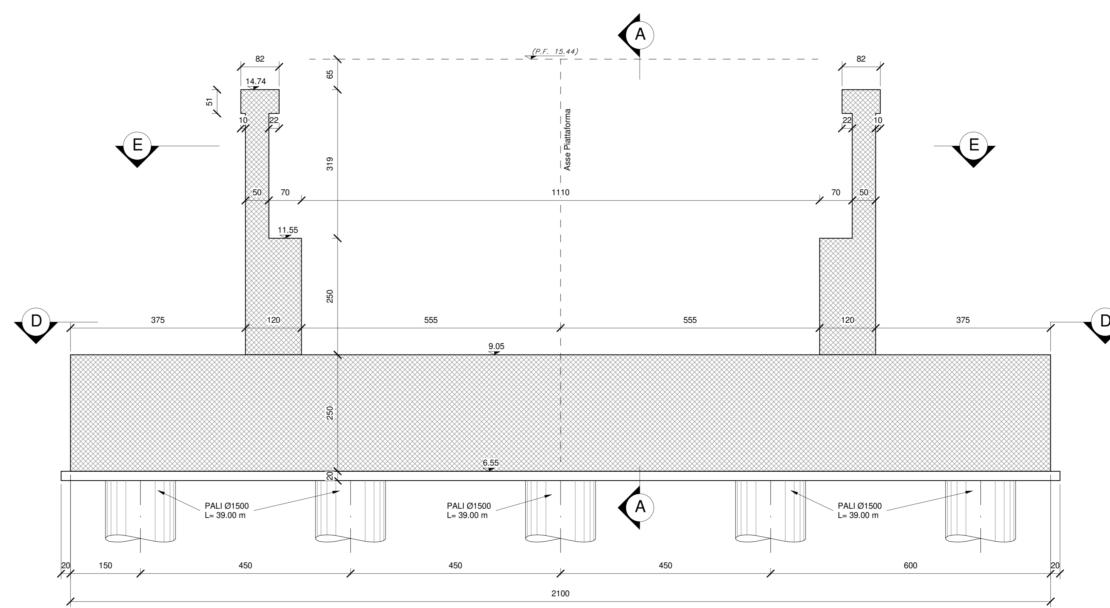
SEZIONE C-C-Scala 1:50
