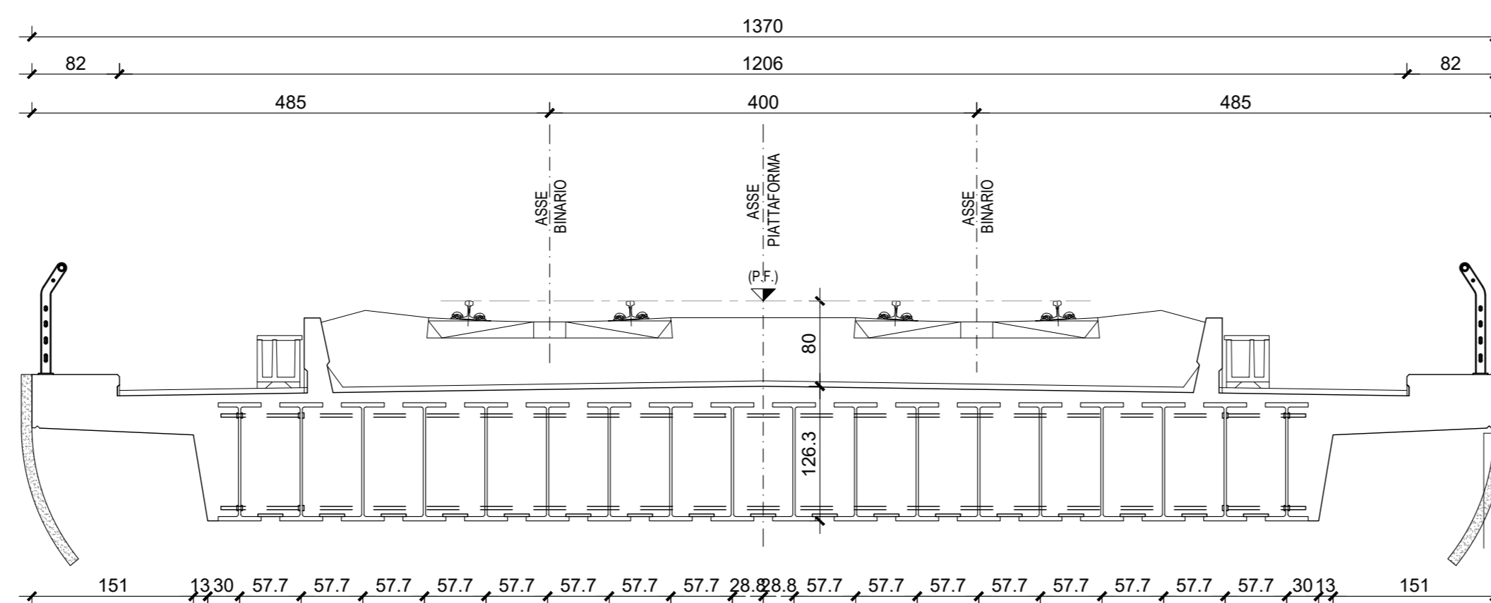
IMPALCATO Scala 1:50 SEZIONE TRASVERSALE TIPO IN CAMPATA
