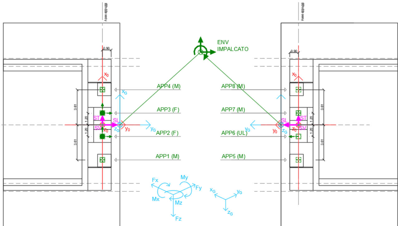
Figura 27- - Schema dei vincoli a terra impalcato
