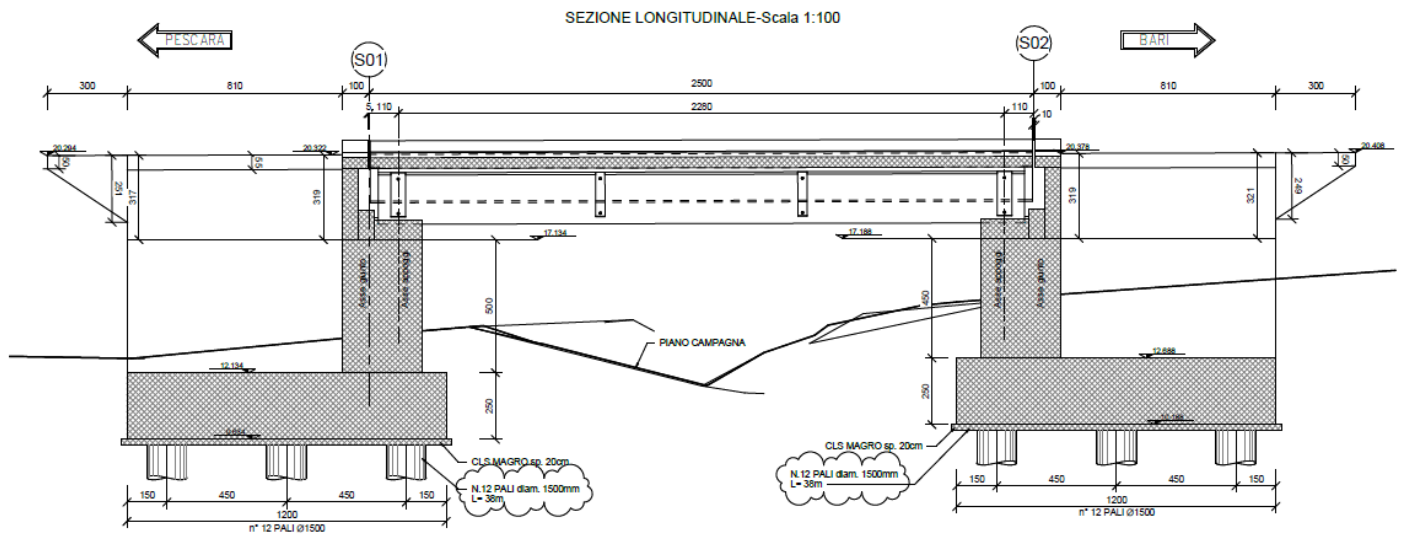
Figura 1 – Profilo longitudinale VI10
