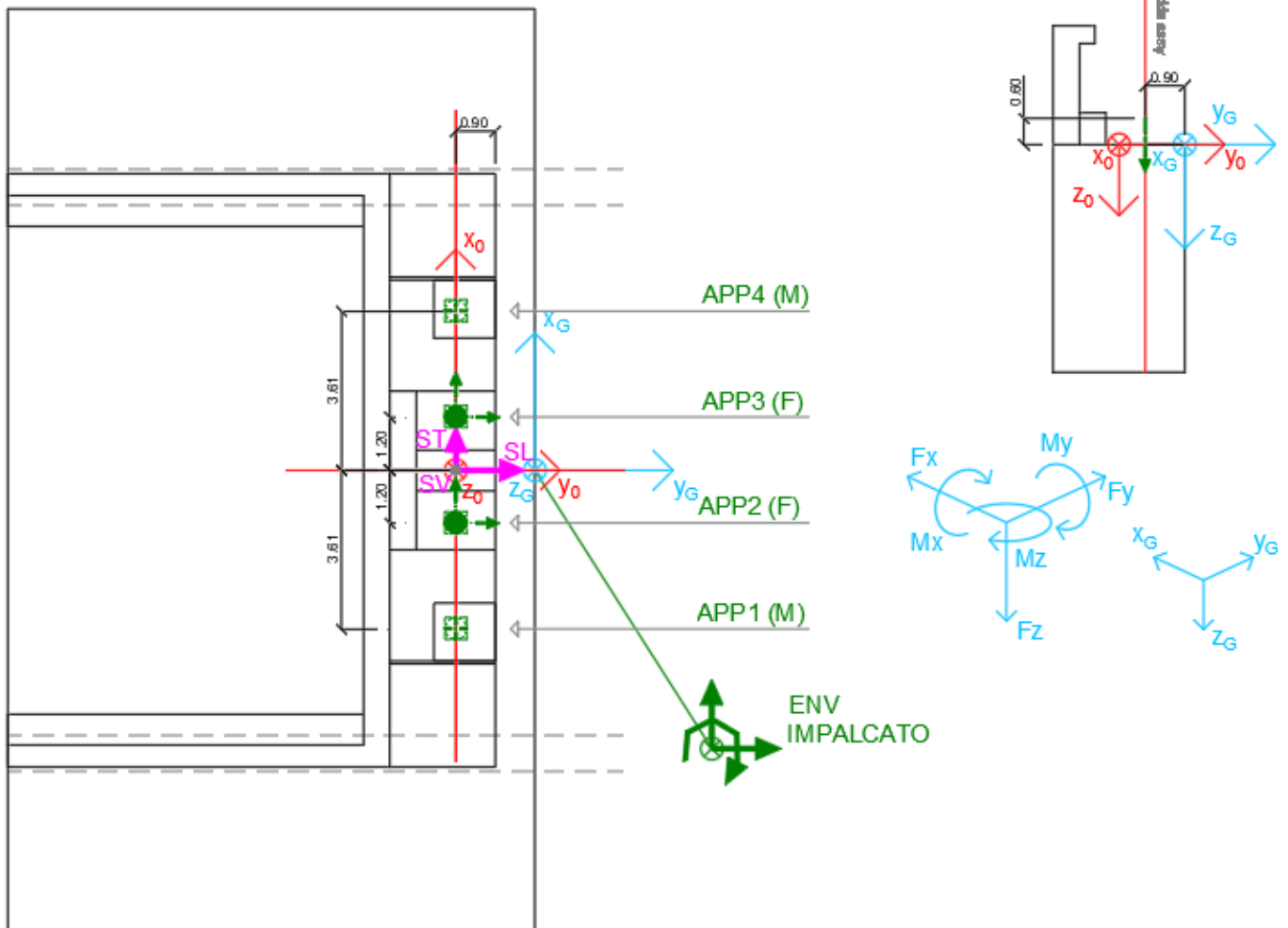
Figura 32 – Schema e sistema di riferimento utilizzato per il calcolo delle azioni applicate
