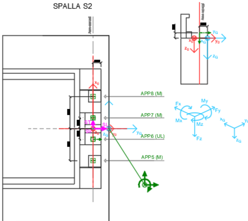
Figura 32 – Schema e sistema di riferimento utilizzato per il calcolo delle azioni applicate
