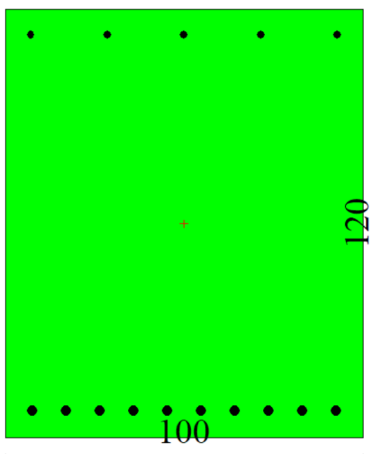
Figura 40 – Sezione trasversale muro d'ala e relativa armatura
