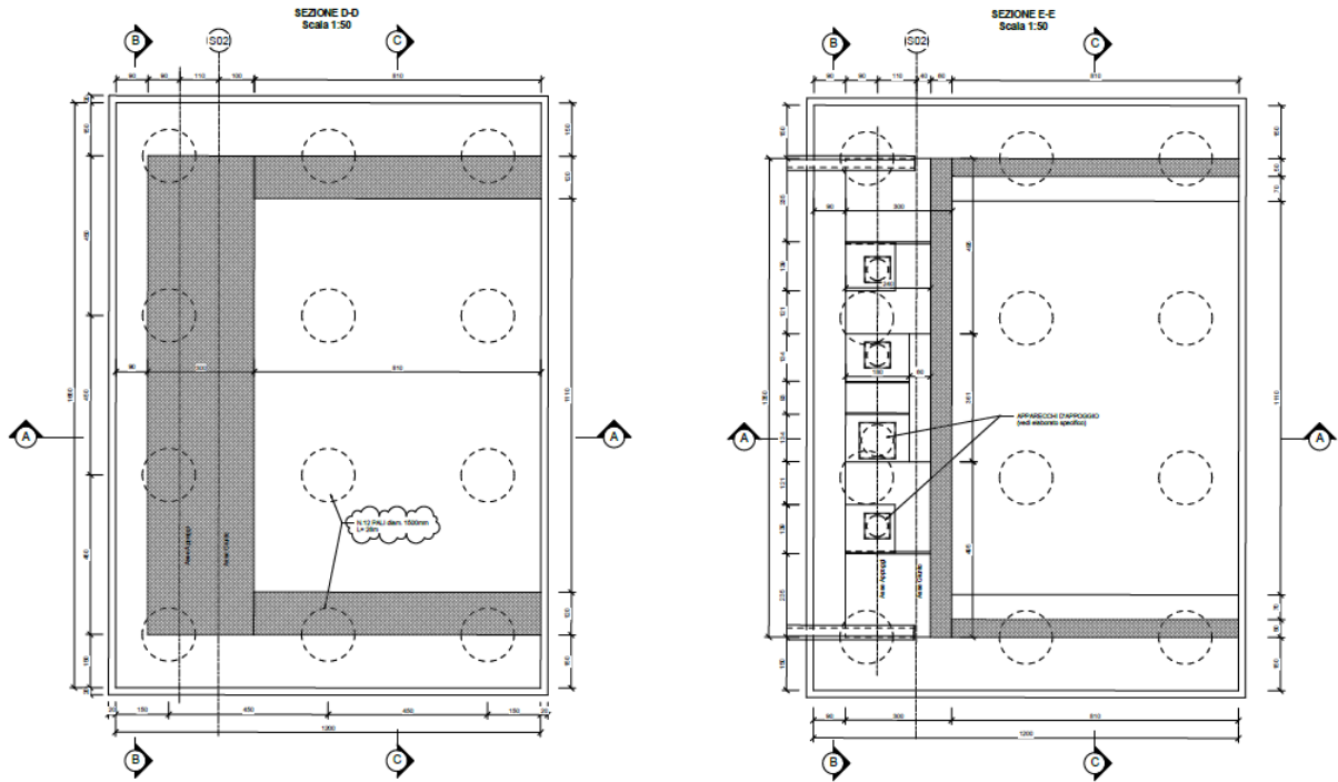
Figura 4 – Vista in pianta
