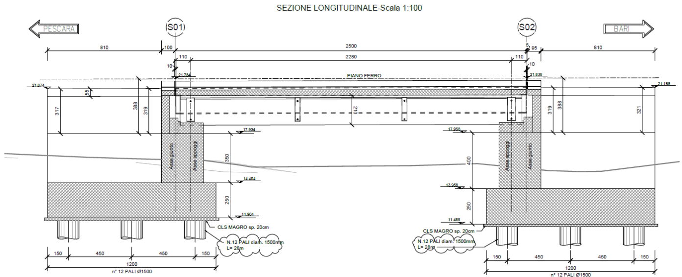
Figura 1 – Profilo longitudinale VI11
