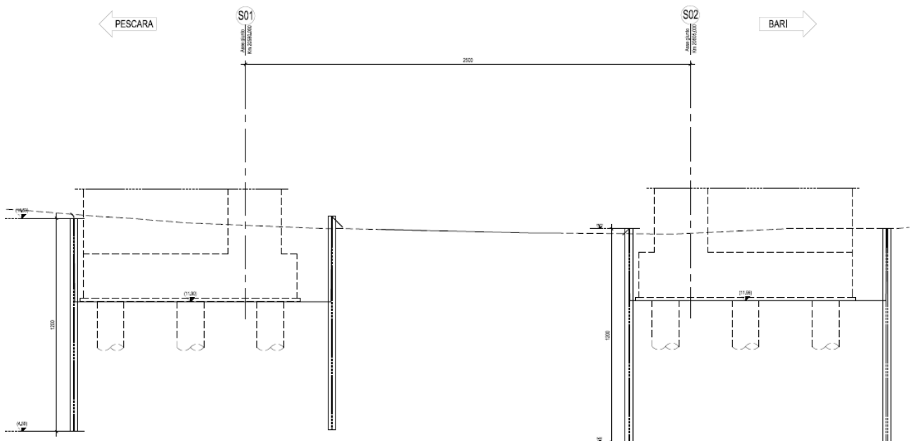
Figura 2 - Sezione del palancolato con sistema di contrasto sommitale
