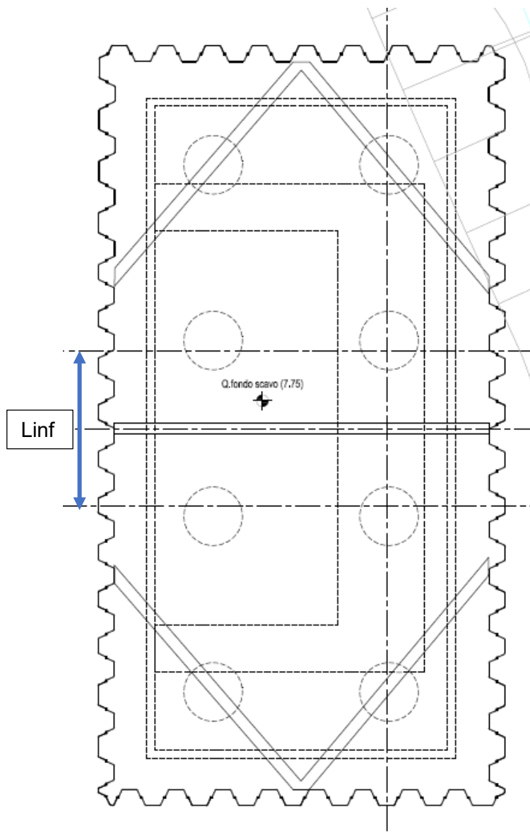
Figura 4: schema di calcolo azione assiale puntone
