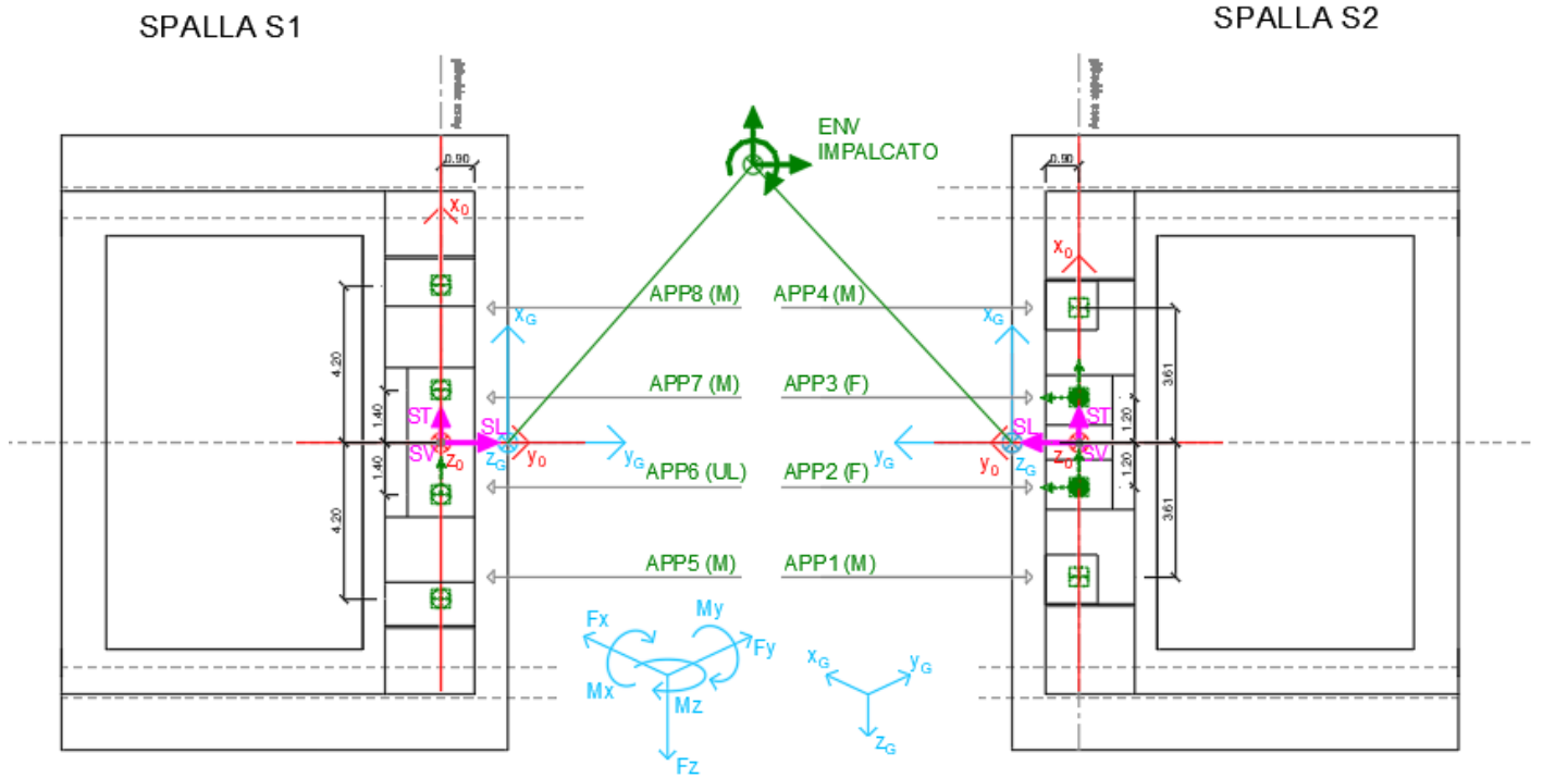
Figura 27- - Schema dei vincoli a terra impalcato
